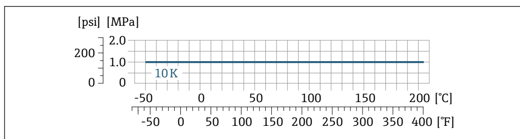
図 26 フランジ材質：1.4539 (SUS 890L 相当)；ラップジョイントフランジ（非接液）：1.4404 (SUS 316 または 316L 相当)
