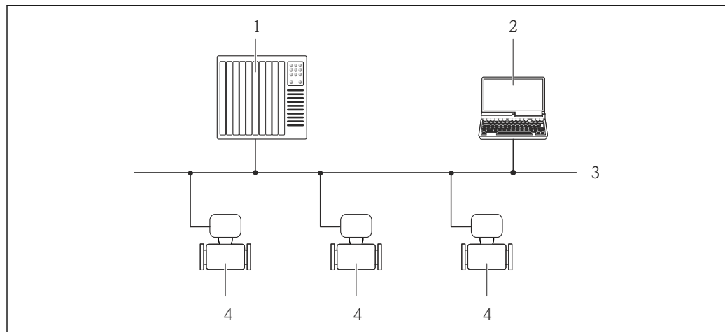
図 41 PROFIBUS DP ネットワークを介したリモート操作のオプション
