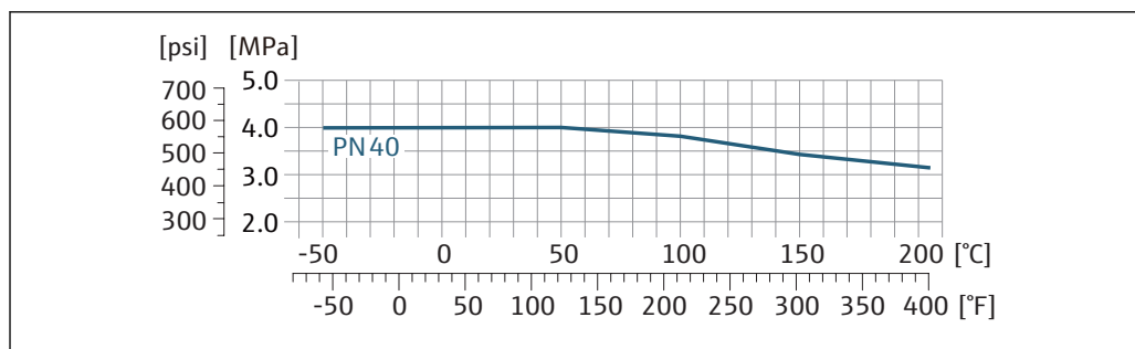
図 24 フランジ材質：1.4539 (SUS 890L 相当)、アロイ C22；ラップジョイントフランジ（非接液）：1.4404 (SUS 316 または 316L 相当)
