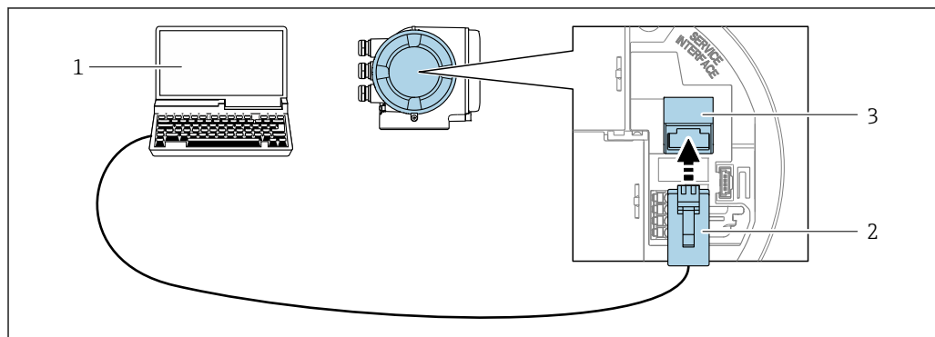
図 48 サービスインターフェイス (CDI-RJ45) 経由の接続
