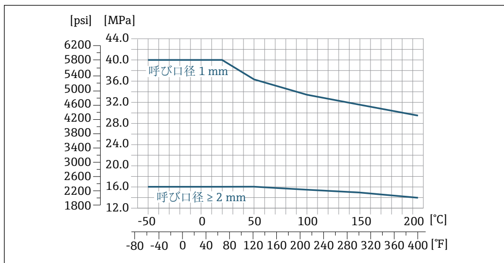
図 27 4-VCO-4 カップリング : 1.4539 (SUS 890L 相当) ; 8-VCO-4 カップリング : 1.4539 (SUS 890L 相当) ; NPTF ネジ込み式アダプタ : 1.4539 (SUS 890L 相当)
