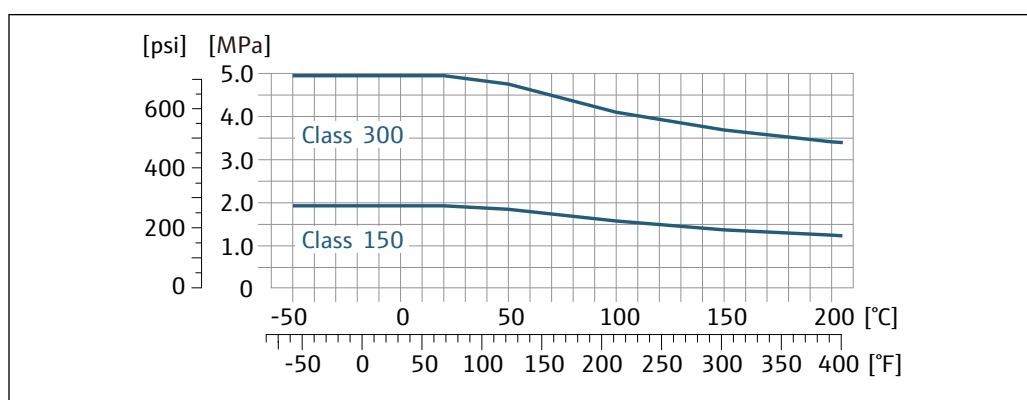
図 25 フランジ材質：1.4539 (SUS 890L 相当)；ラップジョイントフランジ（非接液）：1.4404 (SUS 316 または 316L 相当)
