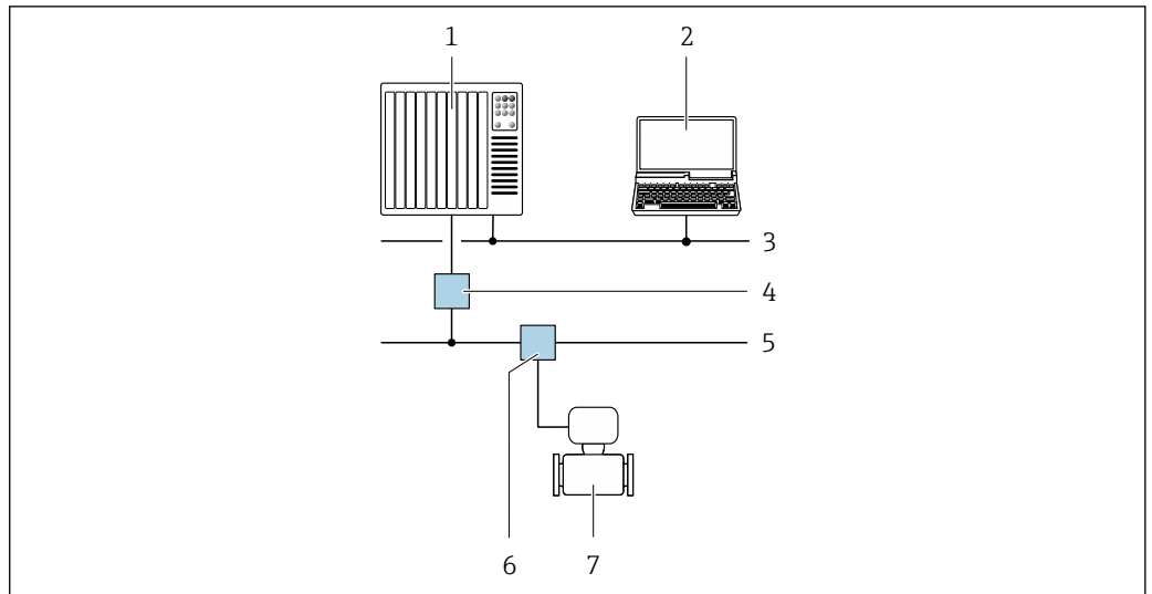
図 42 PROFIBUS PA ネットワークを介したリモート操作のオプション
