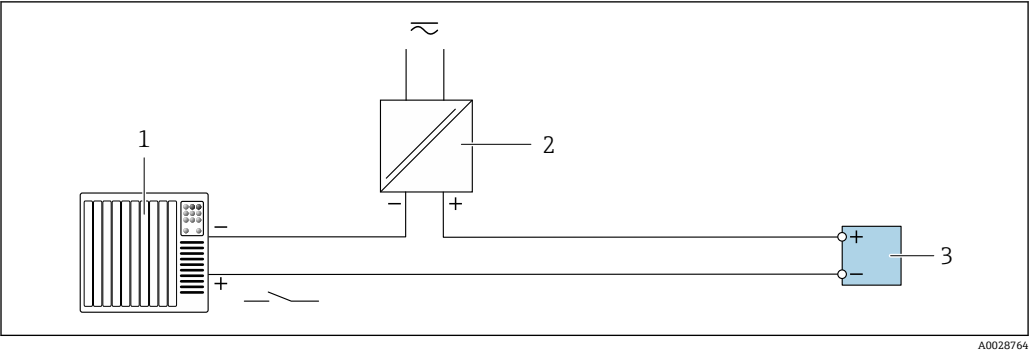
図 20 ステータス入力の接続例 1 オートメーションシステム、ステータス出力付き（例：PLC） 2 電源 3 変換器
