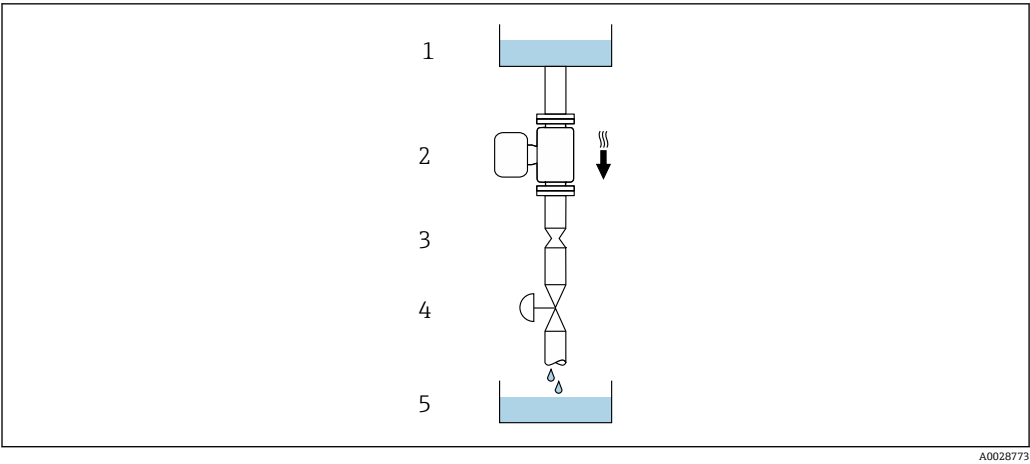
図 21 下り方向の垂直配管での設置（例: バッチアプリケーション用）
