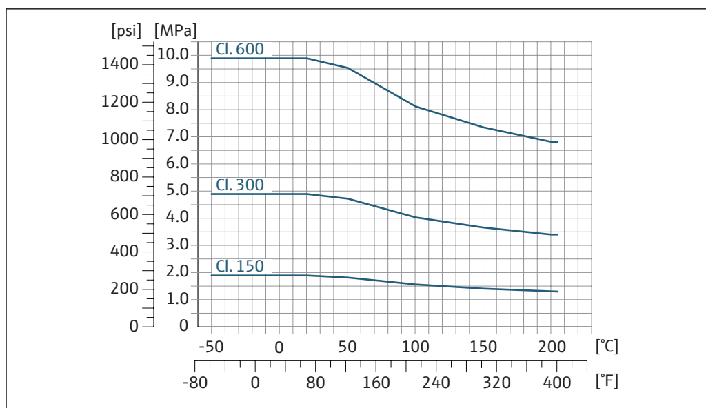
図 28 ラップジョイントフランジ、フランジ材質：1.4301 (SUS F304 相当)、接液部 アロイ C22：2.4602 (UNS N06022)
