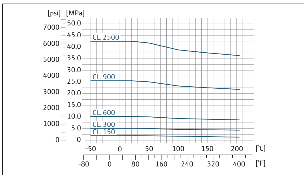
26 フランジ材質：1.4404 (SUS 316 または 316L 相当)
