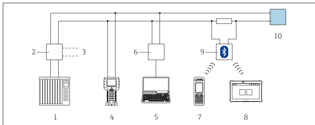
図 45 HART プロトコル経由のリモート操作オプション (パッシブ)
