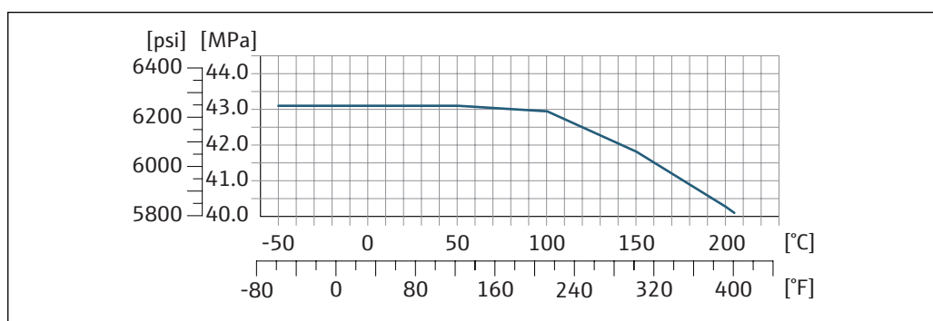
図 33 フランジ材質：アロイ C22、2.4602 (UNS N06022)
