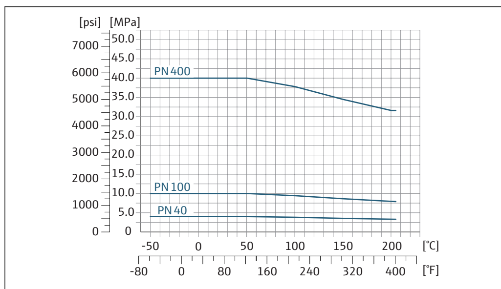
図 23 フランジ材質：1.4404 (SUS 316 または 316L 相当)
