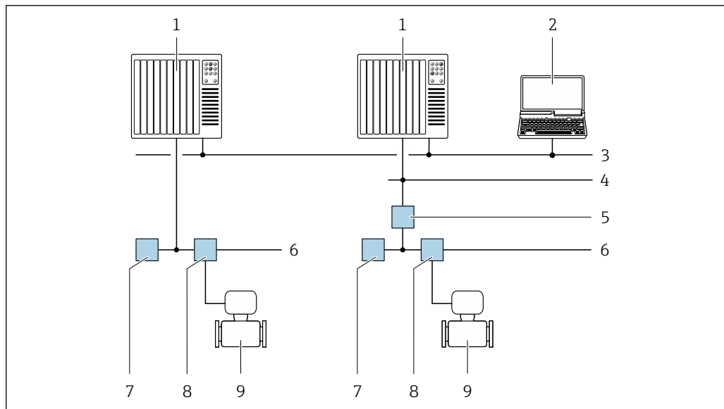
図 46 FOUNDATION フィールドバスネットワークを介したリモート操作のオプション
