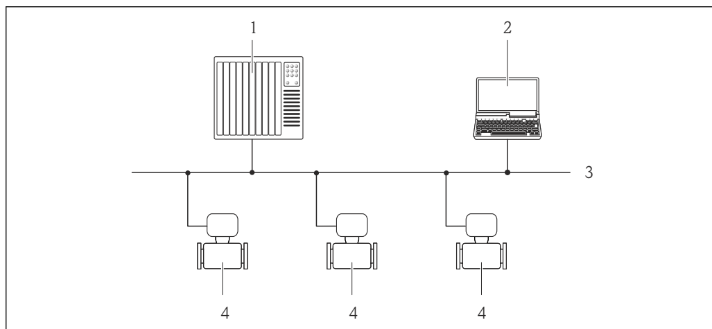
図 47 PROFIBUS DP ネットワークを介したリモート操作のオプション
