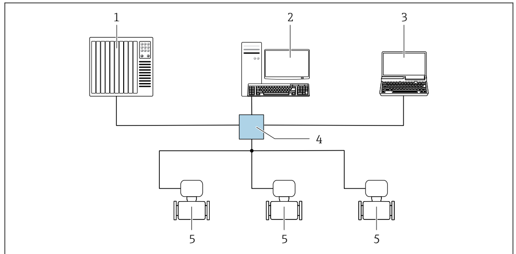
図 50 EtherNet/IP ネットワーク経由のリモート操作オプション：スター型トポロジー
