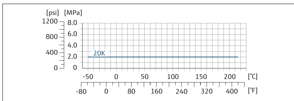
図 30 ラップジョイントフランジ、フランジ材質：1.4301 (SUS F304 相当)、接液部 アロイ C22：2.4602 (UNS N06022)
