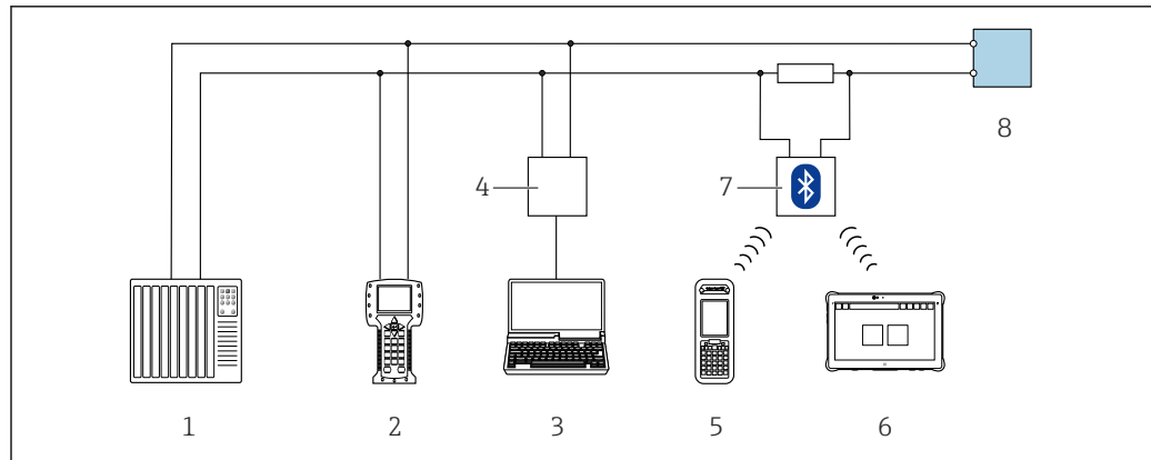
図 44 HART プロトコル経由のリモート操作オプション (アクティブ)
