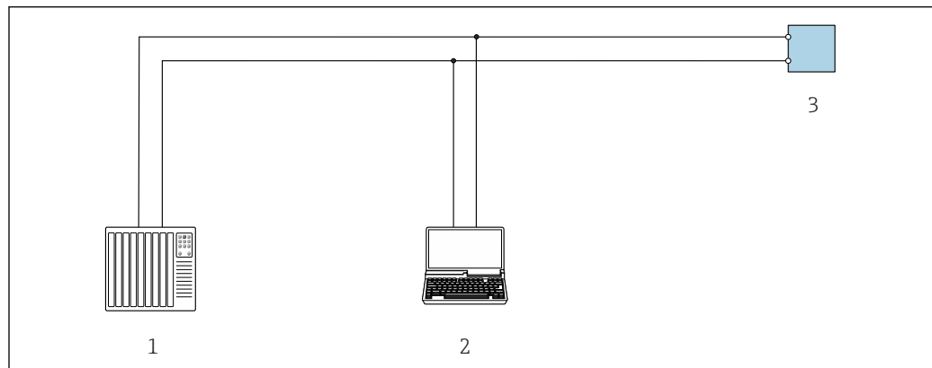
図 49 Modbus-RS485 プロトコル経由のリモート操作オプション（アクティブ）
