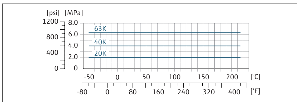
図 29 フランジ材質：1.4404 (SUS 316 または 316L 相当) またはアロイ C22、2.4602 (UNS N06022)
