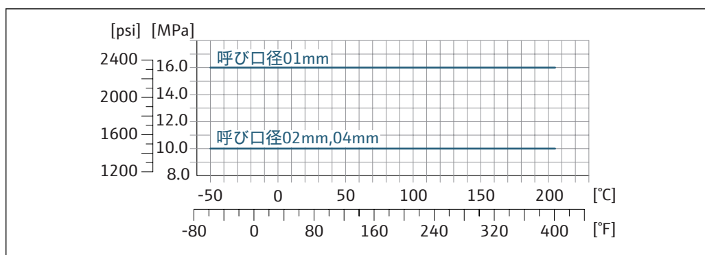
図 31 フランジ材質：1.4404 (SUS 316 または 316L 相当)
