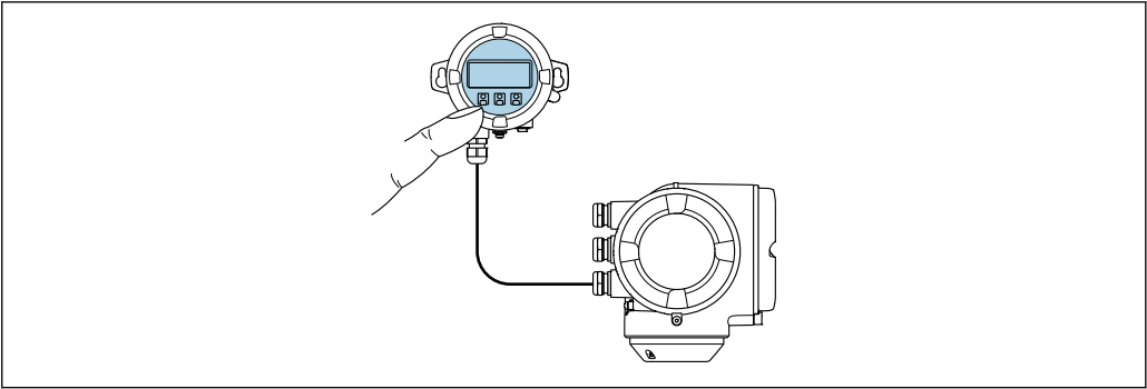
図 43 分離ディスプレイと操作モジュール DKX001 を介した操作
