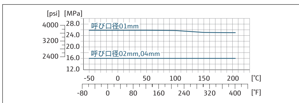
図 32 フランジ材質：アロイ C22、2.4602 (UNS N06022)
