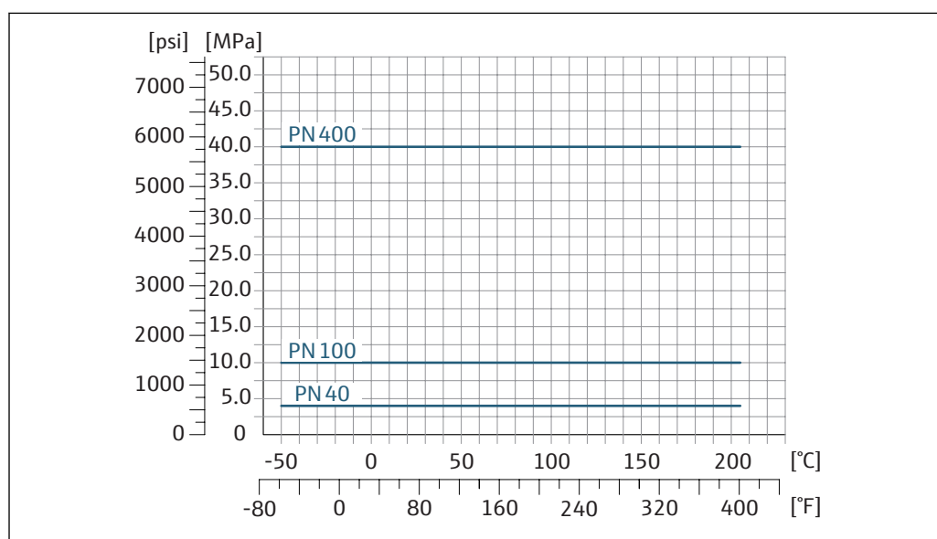
図 24 フランジ材質：アロイ C22、2.4602 (UNS N06022)
