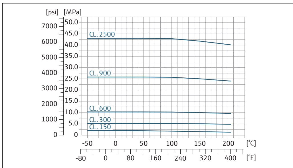
27 フランジ材質：アロイ C22、2.4602 (UNS N06022)
