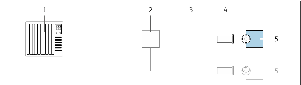
図 22 EtherNet/IP の接続例
