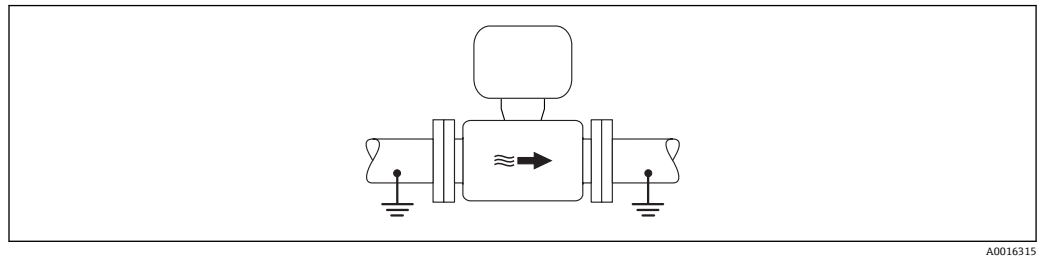
図 19 計測チューブを介した電位平衡
