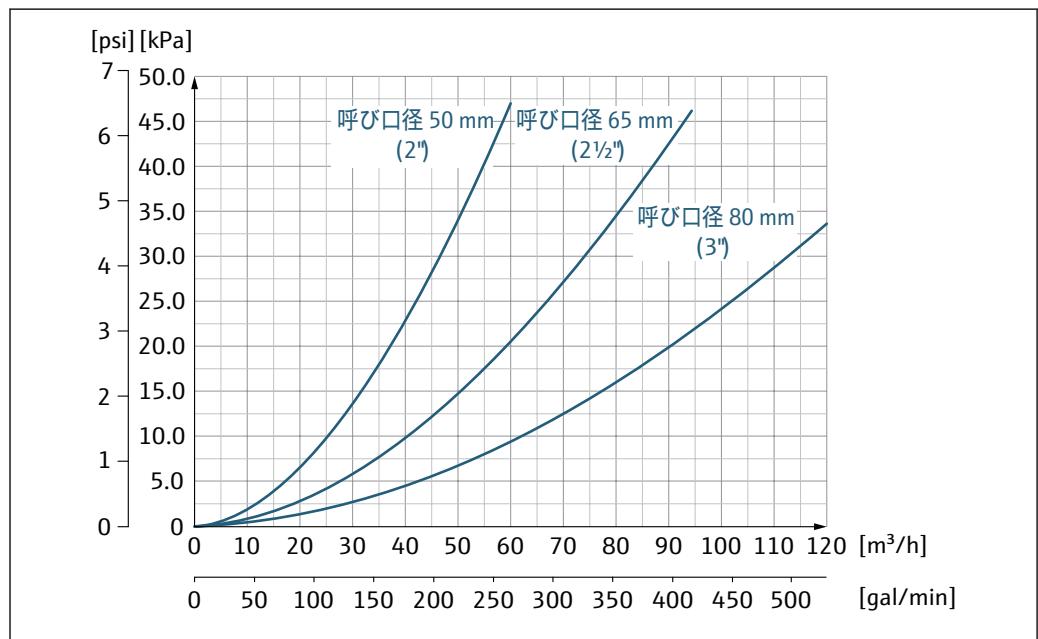
図 46 呼び口径 50~80 mm (2~3") の圧力損失: 「設計」のオーダーコード、オプション C 「固定フランジ、上流側/下流側直管長なし」の場合
