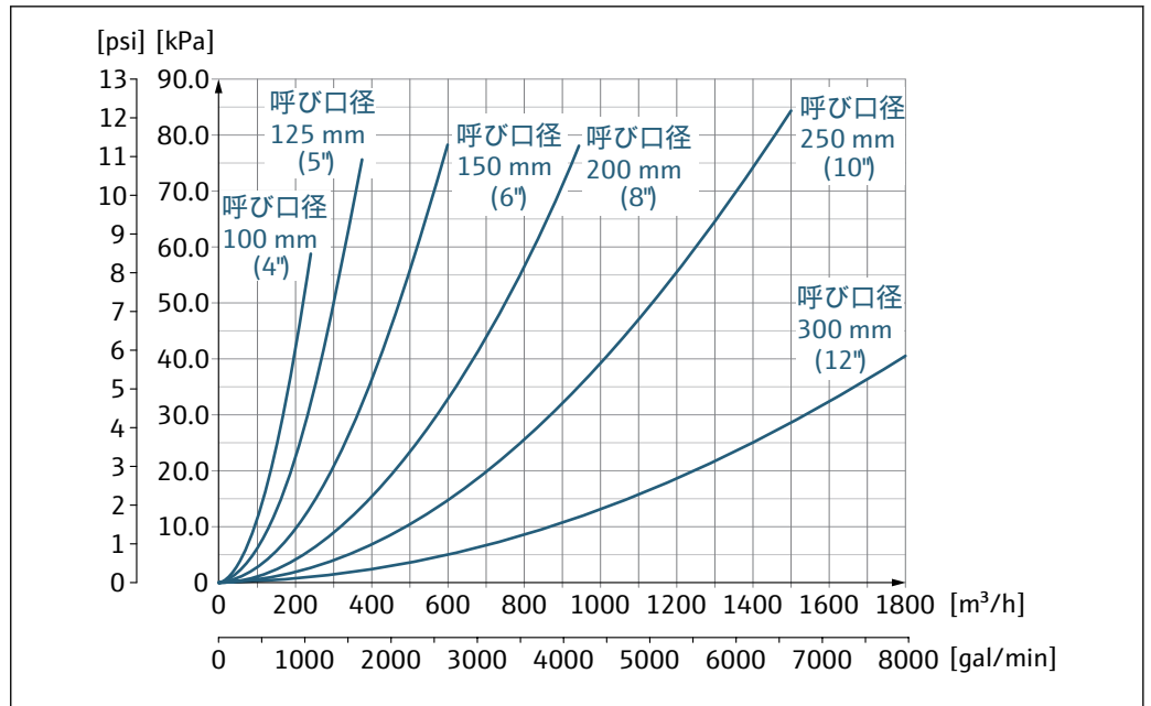
図 47 呼び口径 100~300 mm (4~12") の圧力損失:「設計」のオーダーコード、オプション C「固定フランジ、上流側/下流側直管長なし」の場合
