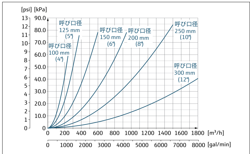
図 48 呼び口径 100～300 mm (4～12") の圧力損失：「設計」のオーダーコード、オプション C「固定フランジ、上流側/下流側直管長なし」の場合
