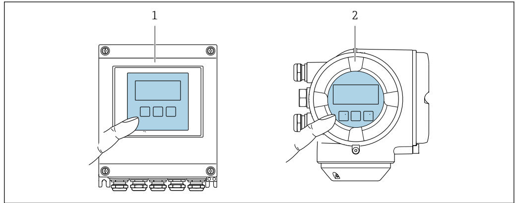
図 50 タッチコントロールによる操作
