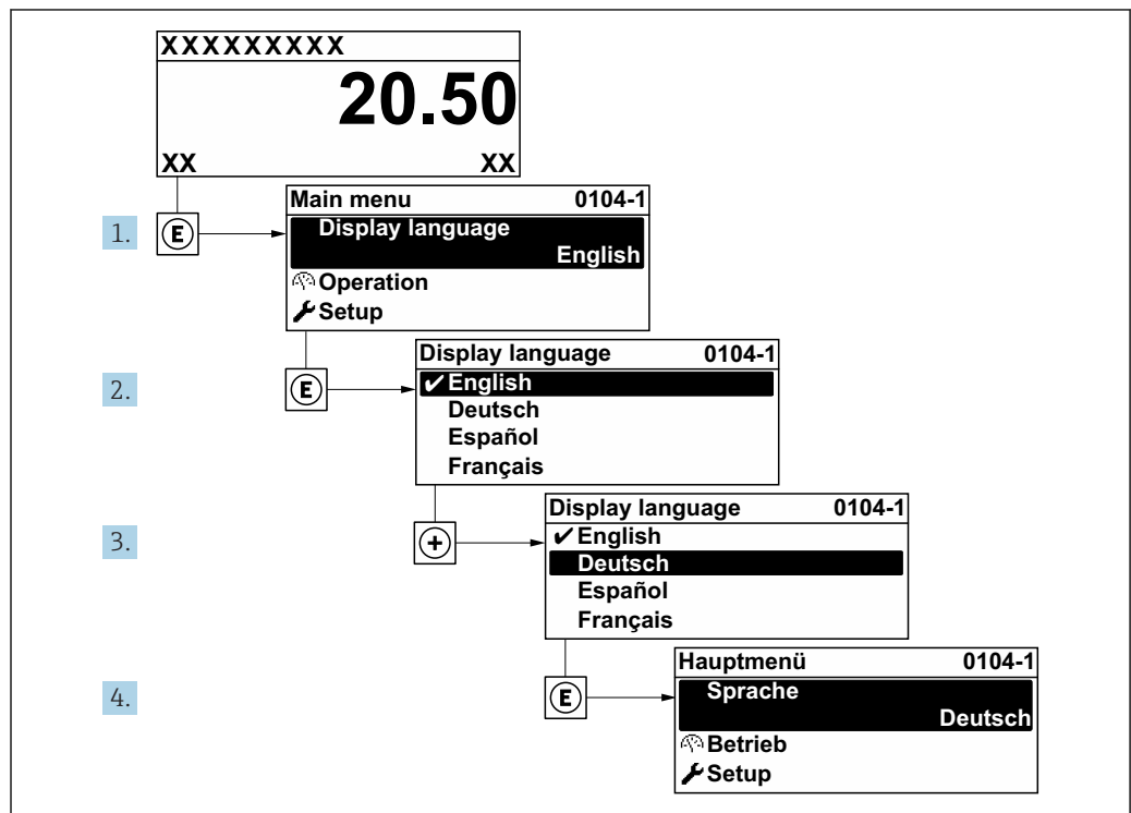
図 38 現場表示器の表示例
