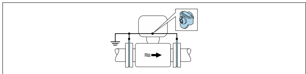
図 22 接地端子およびアースリングを介した電位平衡
