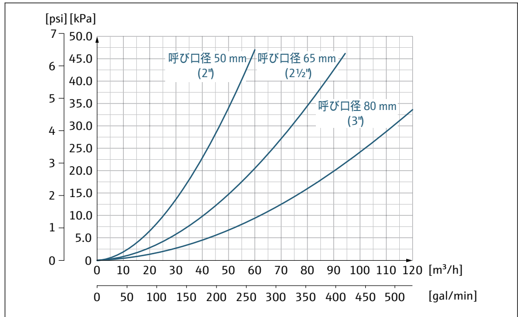
図 47 呼び口径 50～80 mm (2～3") の圧力損失：「設計」のオーダーコード、オプション C「固定フランジ、上流側/下流側直管長なし」の場合
