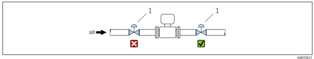
図 6 コントロールバルブ下流側のセンサ設置は推奨されない
