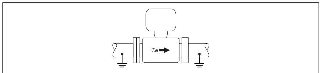
図 20 計測チューブを介した電位平衡
