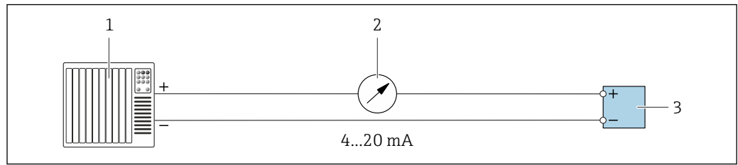
図 24 4~20 mA 電流出力（アクティブ）の接続例
