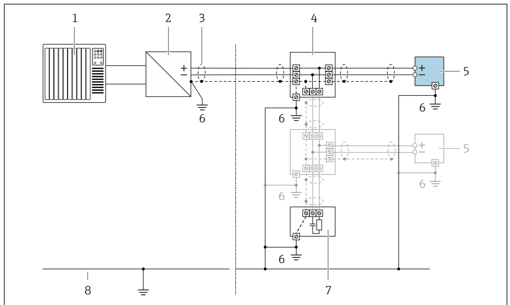
図 23 FOUNDATION フィールドバスの接続例
