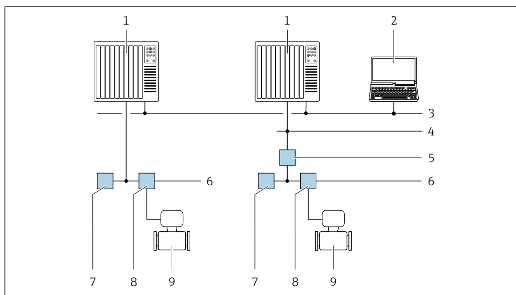
図 35 FOUNDATION フィールドバスネットワークを介したリモート操作のオプション
