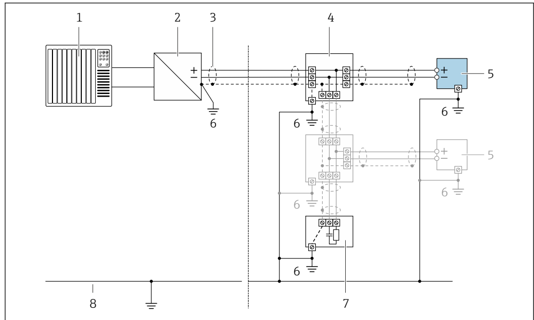
図 17 FOUNDATION フィールドバスの接続例
