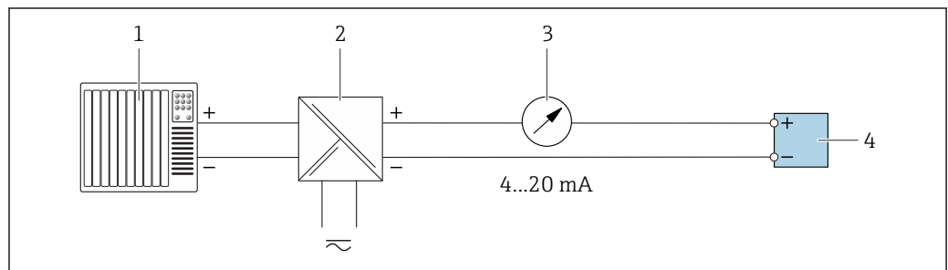
図 25 4~20 mA 電流出力（パッシブ）の接続例
