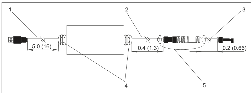
図 3 Commubox FXA291 およびコンポーネント、寸法単位 m (ft)
