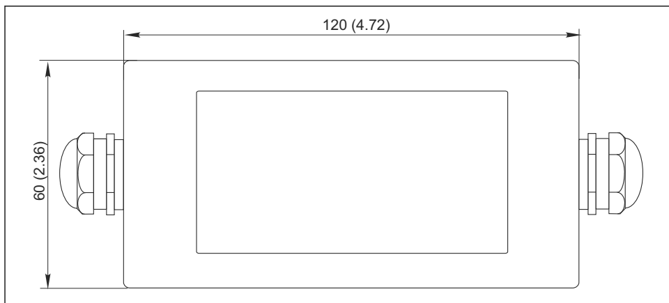
図 4 上面図、寸法単位 mm (inch)
