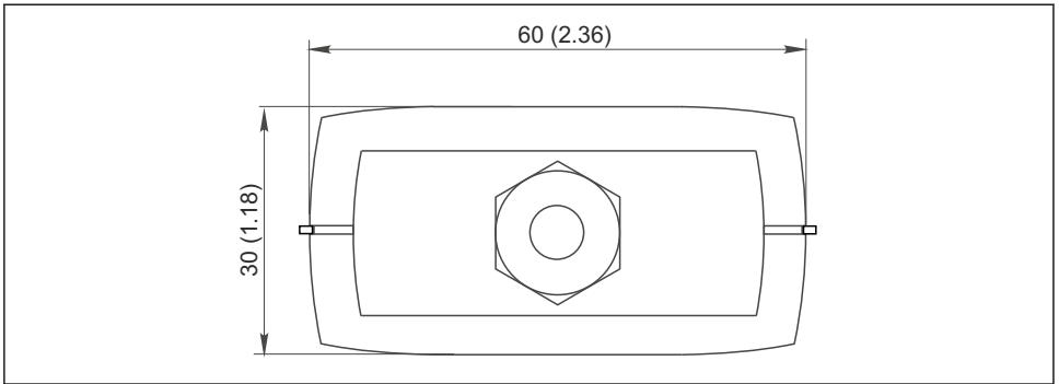
図 5 側面図 (CDI 接続/機器側)、寸法単位 mm (inch)
