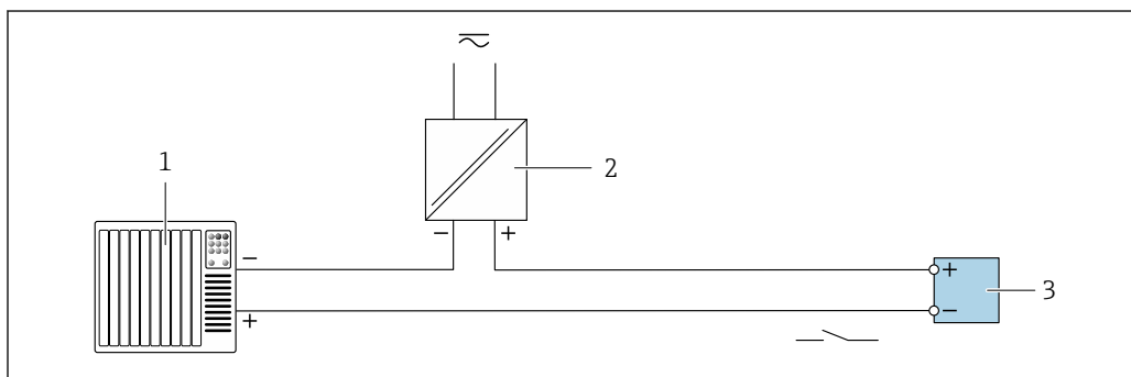
28 Пример подключения релейного выхода (пассивного)
