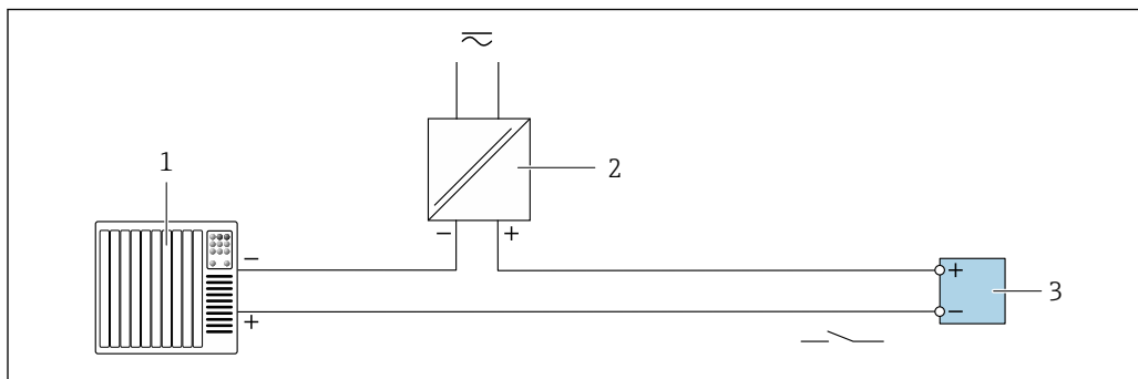
27 Пример подключения для релейного выхода (пассивного)
