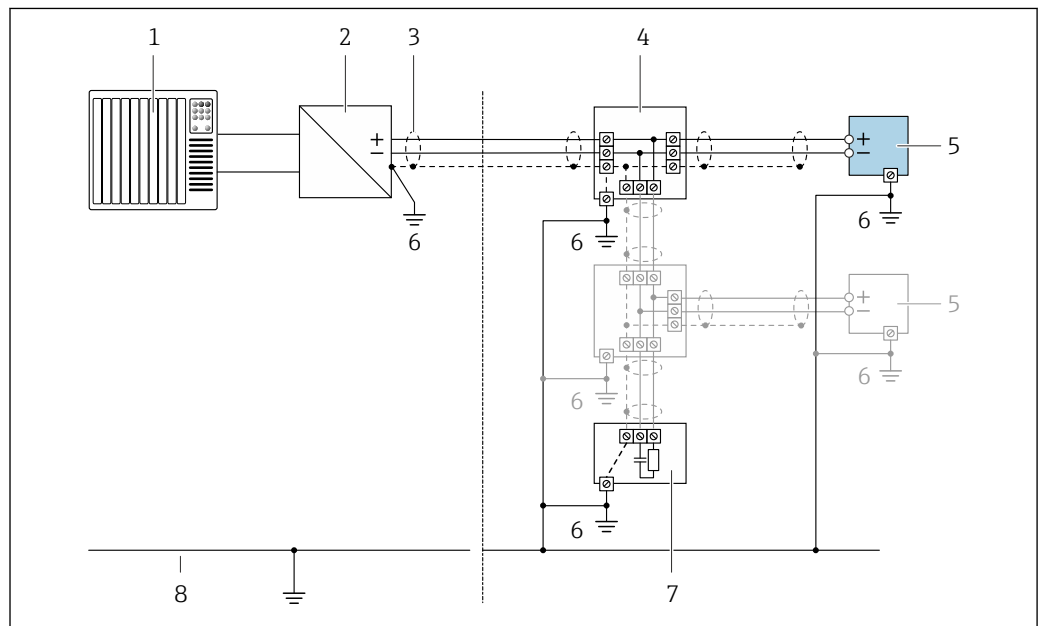
23 Пример подключения для PROFIBUS PA
