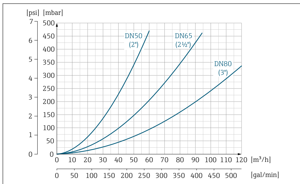
47 Падение давления DN 50–80 (2–3 дюйма) с кодом заказа для параметра «Конструкция», опция C, «Фиксированный фланец, без входных/выходных участков»
