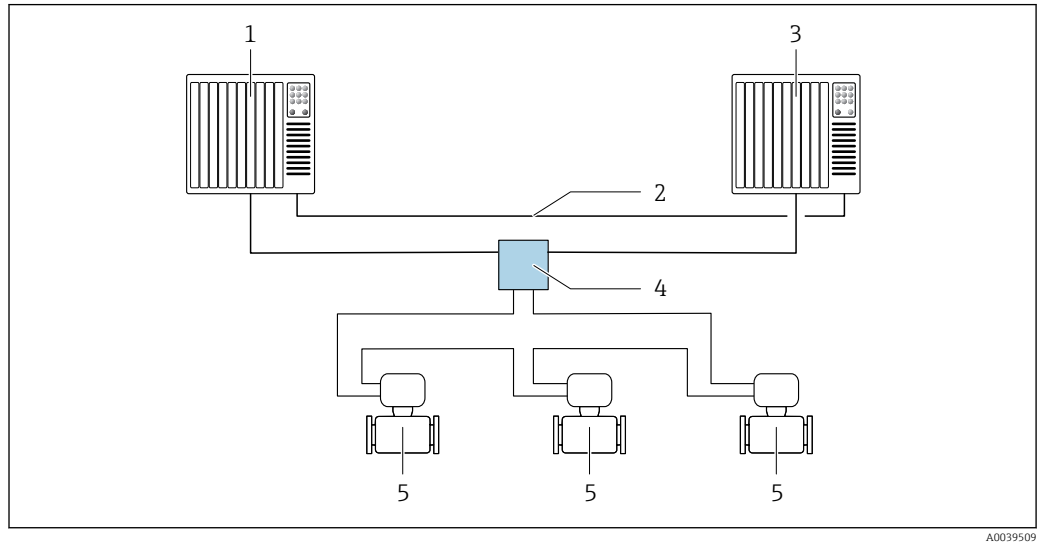
39 Exemplo do layout de um sistema redundante (S2): topologia anelar
