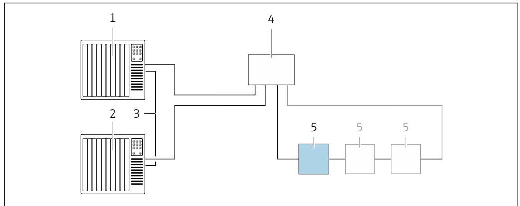
23 Exemplo de conexão para redundância do sistema S2
