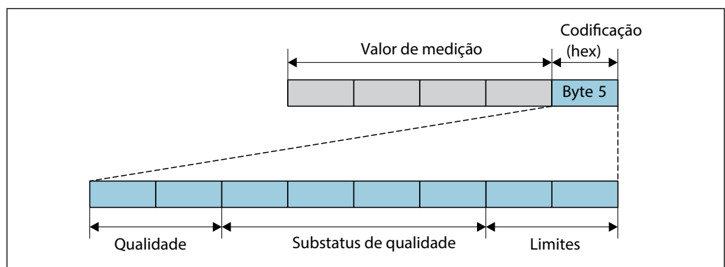
44 Estrutura do do byte de codificação
