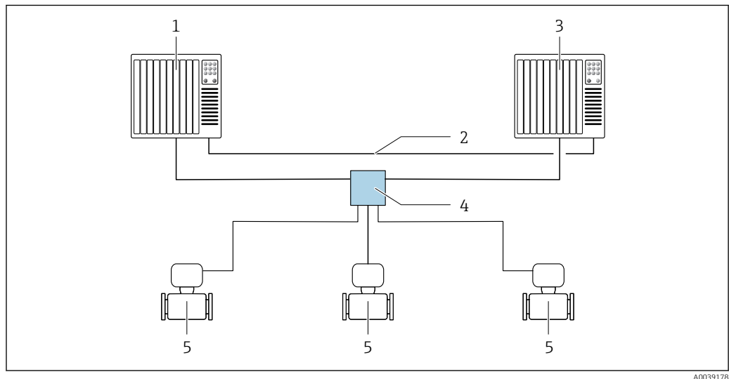
40 Exemplo do layout de um sistema redundante (S2): topologia estrela
