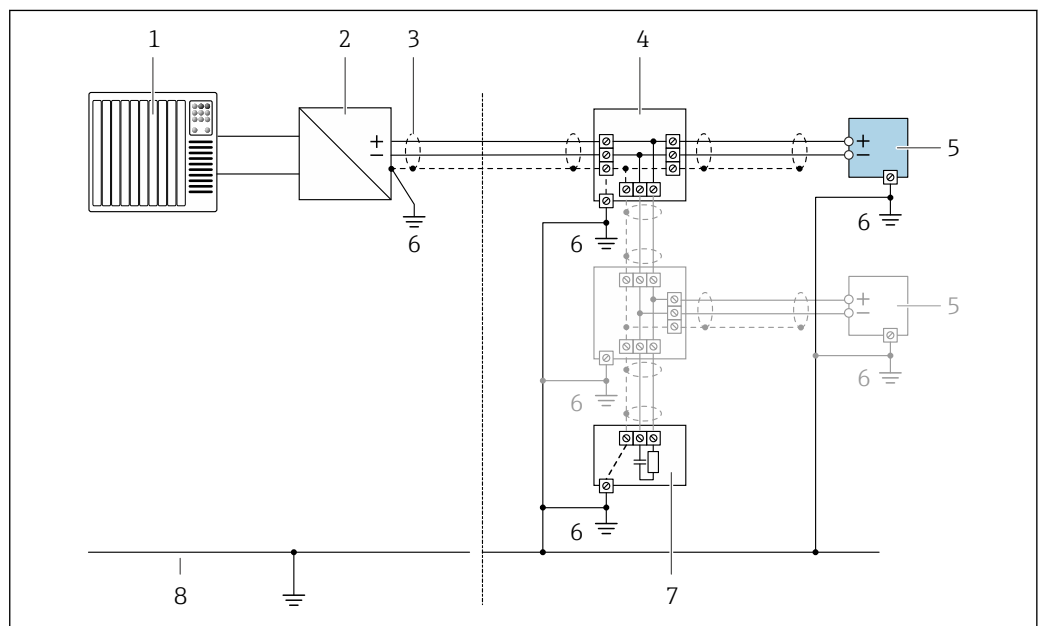
23 Exemplo de conexão para o FOUNDATION Fieldbus
