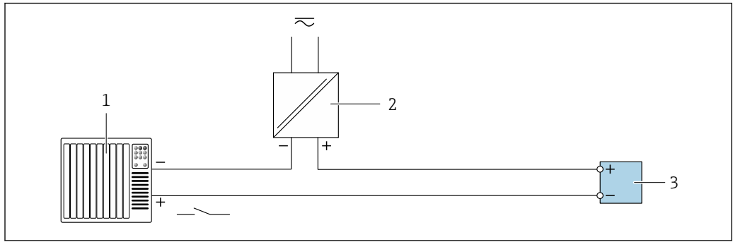
30 Exemplo de conexão para entrada de status
