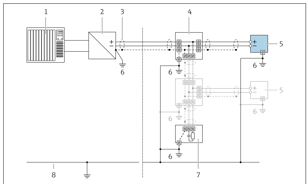
17 Exemplo de conexão para FOUNDATION Fieldbus
