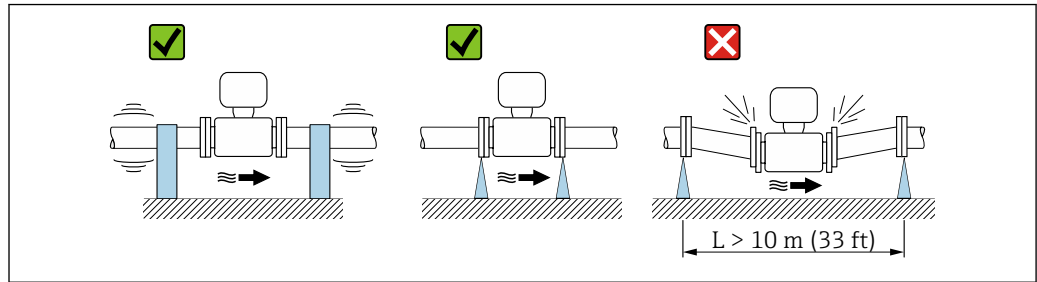
8 Medidas para prevenir a vibração do equipamento
