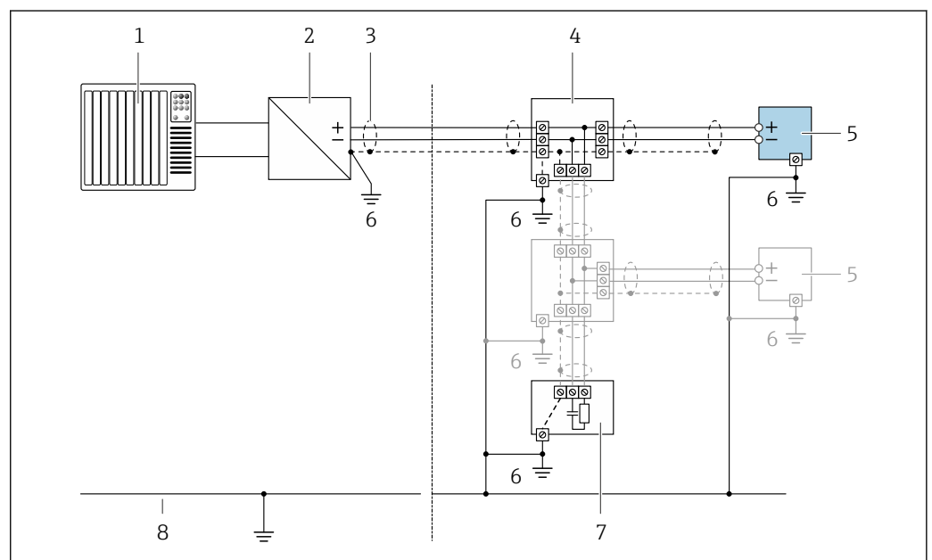
17 Exemplo de conexão para PROFIBUS PA
