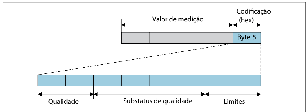
42 Estrutura do byte do status do
