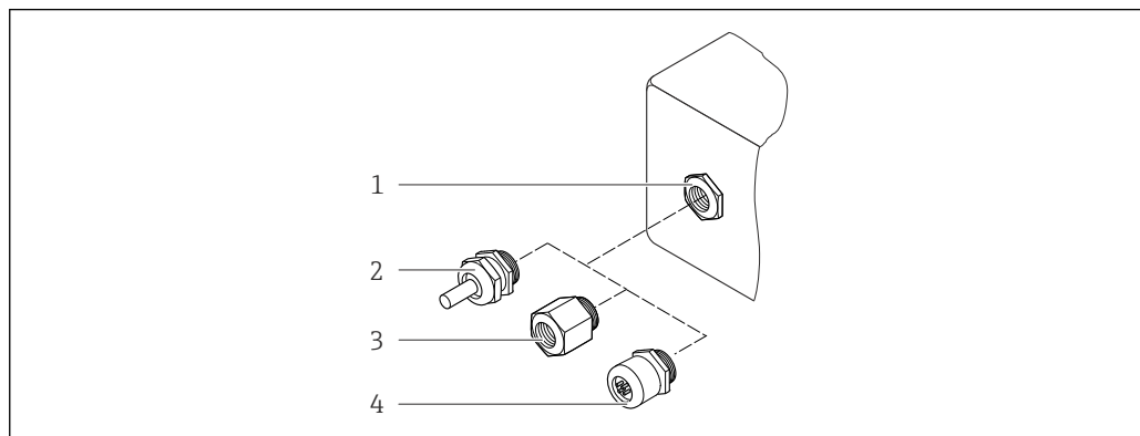
49 Possíveis entradas para cabo/prensa-cabos
