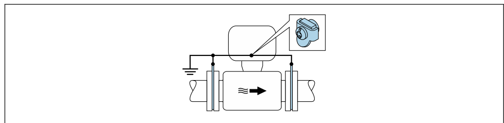
22 Equalização de potencial através de terminal de terra e discos de terra
