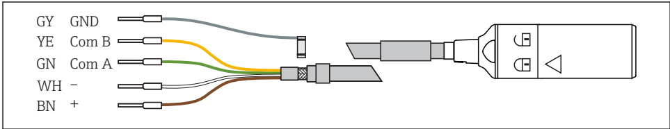
13 Cabo de medição CYK10
