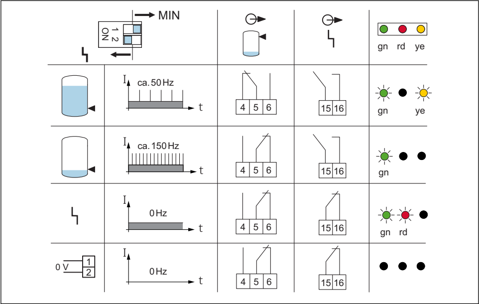
图 16 继电器响应和故障信号
