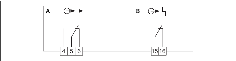
图 8 连接输出信号
