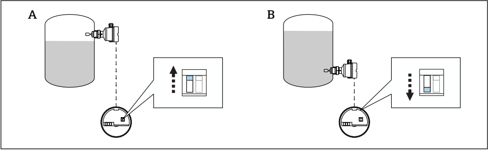
图 13 电子插件上的开关位置 (FEL67)
