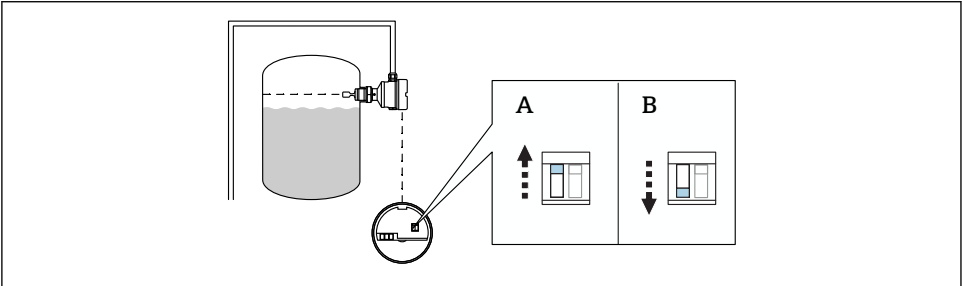
图 14 电子插件上的开关位置 (FEL57)
