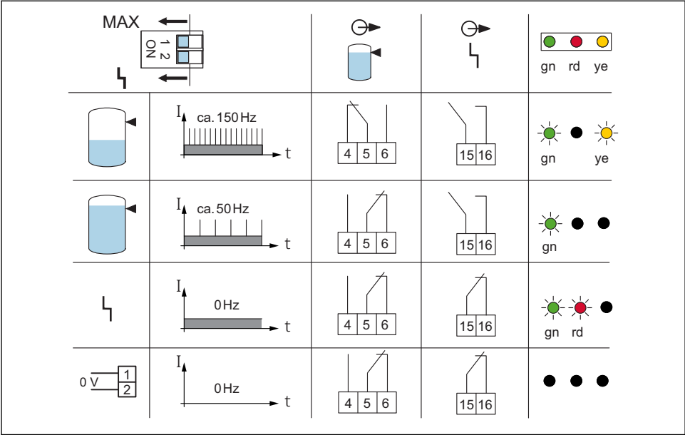
15 继电器响应和故障信号
