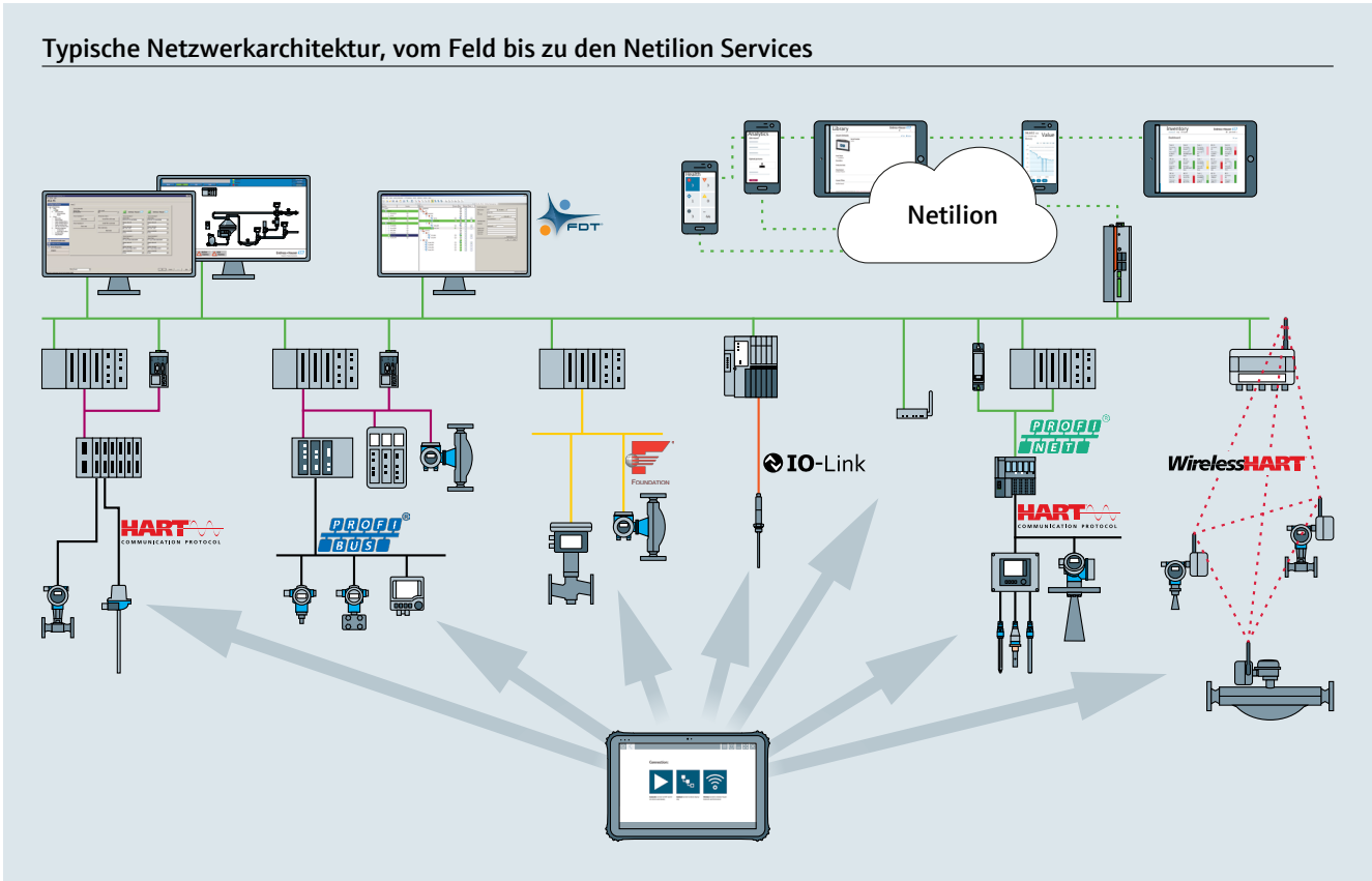
Field Xpert SMT50 kommuniziert mit HART, PROFIBUS, FOUNDATION Fieldbus sowie WirelessHART (und vielen weiteren) Feldgeräten
