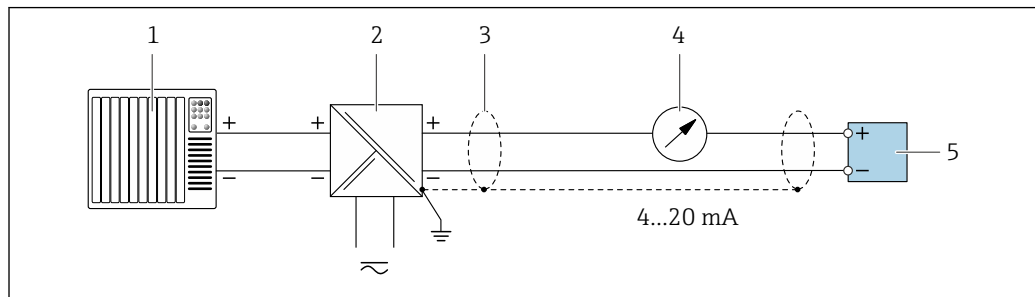
4 Exemplo de conexão para saída de corrente de 4 a 20 mA HART (passiva)
