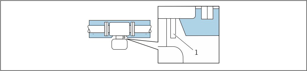
21 Isolamento térmico com pescoço estendido livre e célula de medição de pressão
