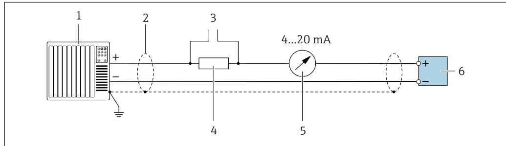
3 Exemplo de conexão para saída de corrente de 4 a 20 mA HART (ativa)
