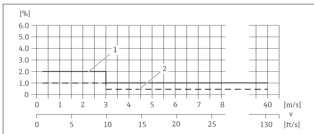
Fig. 16 Exemplo para erro medido máximo (vazão volumétrica) em % o.r.
