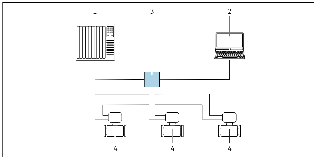
51 Opcje obsługi zdalnej z wykorzystaniem protokołu PROFINET: sieć o topologii pierścienia
