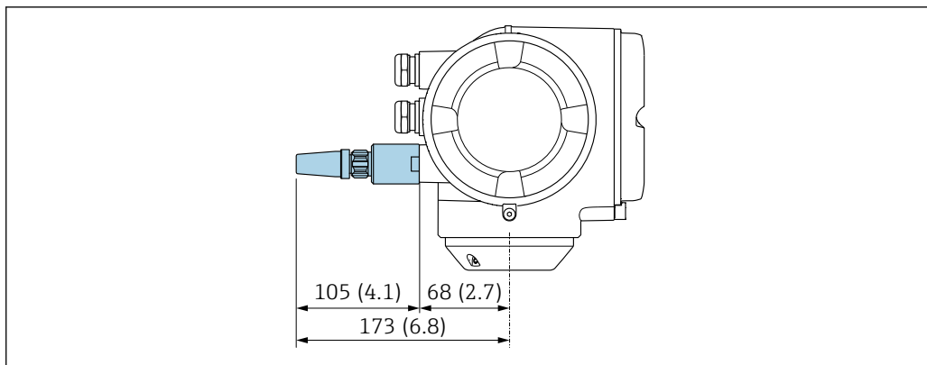
37 Jednostka: mm (cale)
