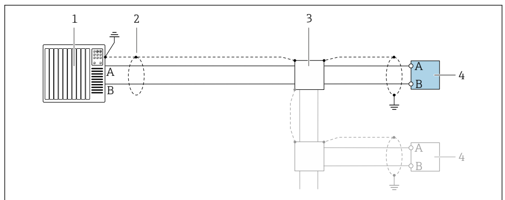
6 Przykład podłączenia wersji PROFIBUS, strefa niezagrażona wybuchem i Strefa 2/Dział 2
