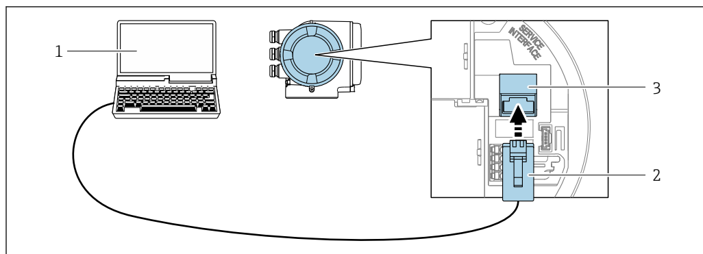
52 Podłączenie poprzez interfejs serwisowy (CDI-RJ45)
