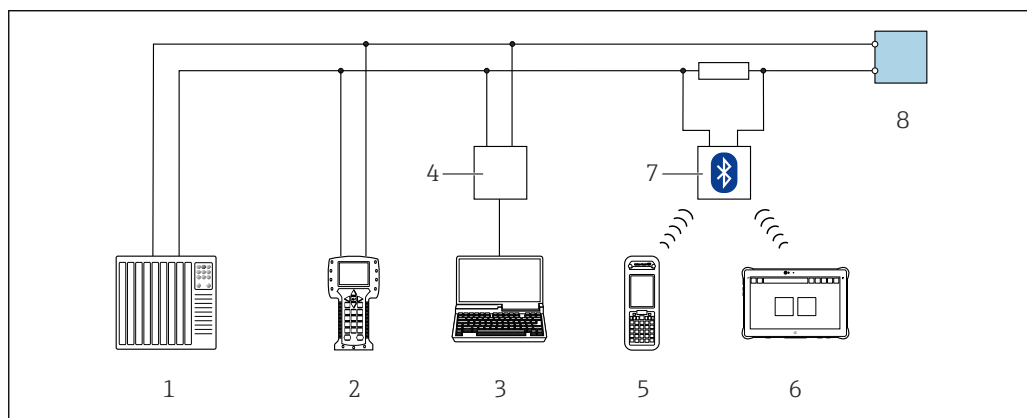
42 Opcje obsługi zdalnej z wykorzystaniem systemu sterowania z wyjściem HART (aktywnym)
