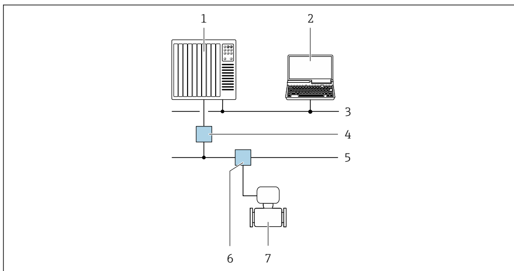
46 Opcje obsługi zdalnej z wykorzystaniem protokołu PROFIBUS PA
