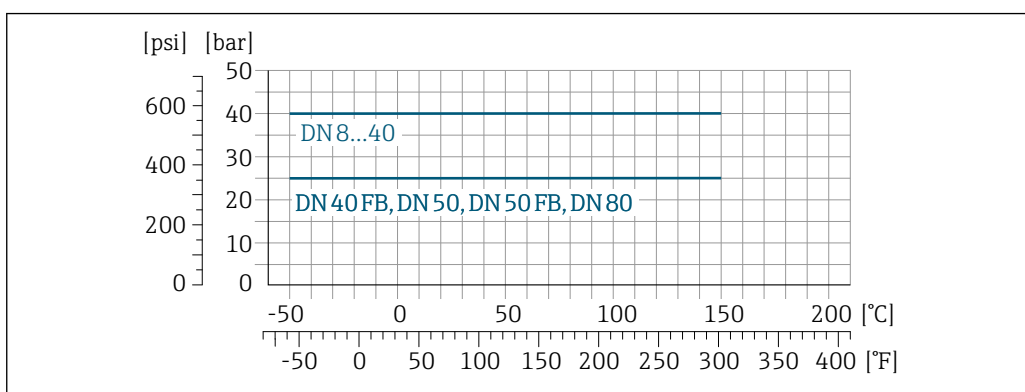
27 Materiał przyłącza gwintowego: tytan Grade 2
