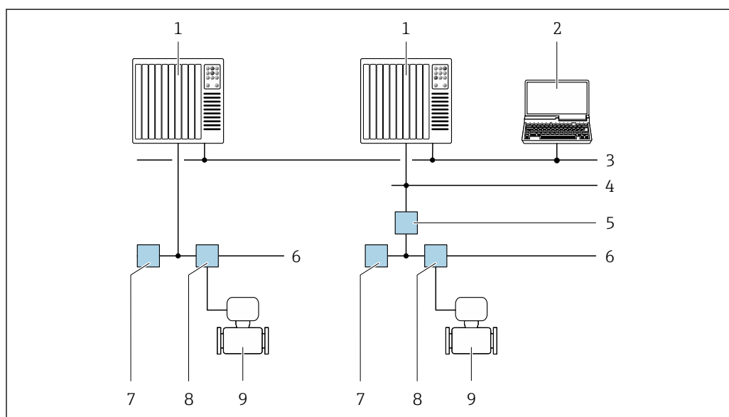
44 Opcje obsługi zdalnej z wykorzystaniem protokołu FOUNDATION Fieldbus
