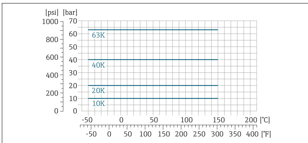
25 Materiał kołnierza: stal k.o. 1.4301 (304). Części zwilżane: tytan.
