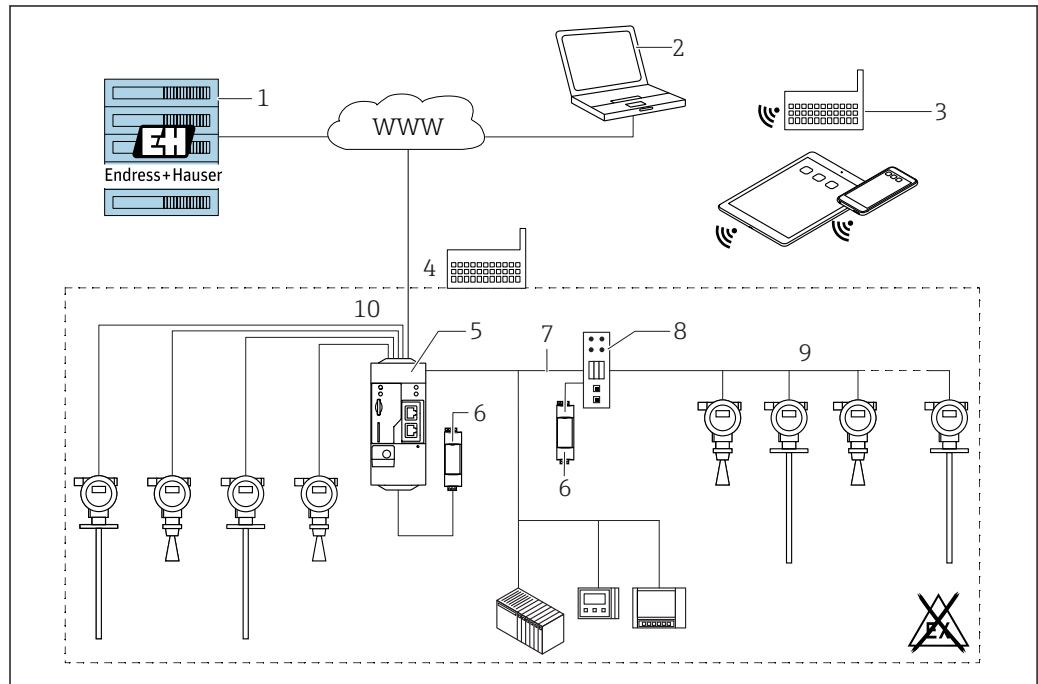
図 47 SupplyCare Hosting SCH30 を使用した在槽管理プラットフォームの例
