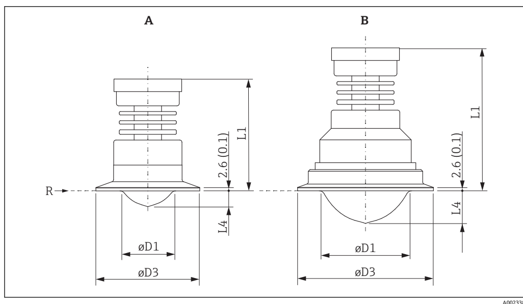
図 36 トリクランプ接続付き機器の寸法。測定単位 mm (in)
