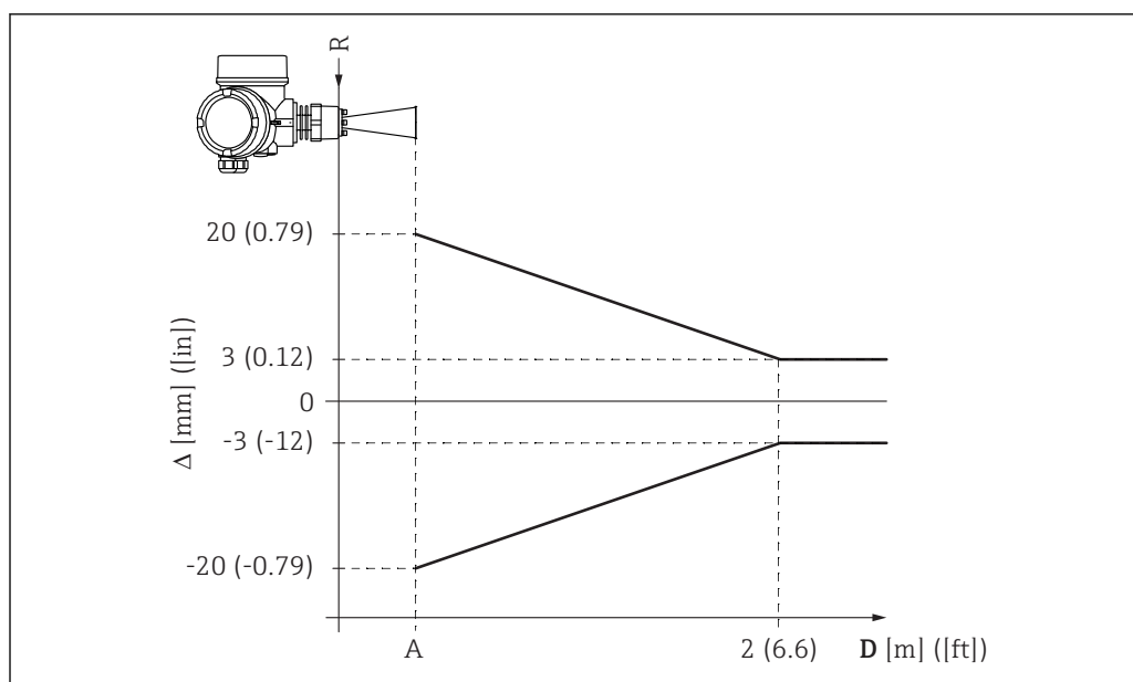
図 19 近範囲アプリケーションにおける最大測定誤差、「アドバンスドダイナミックス」アプリケーションパッケージ付きバージョンの値
