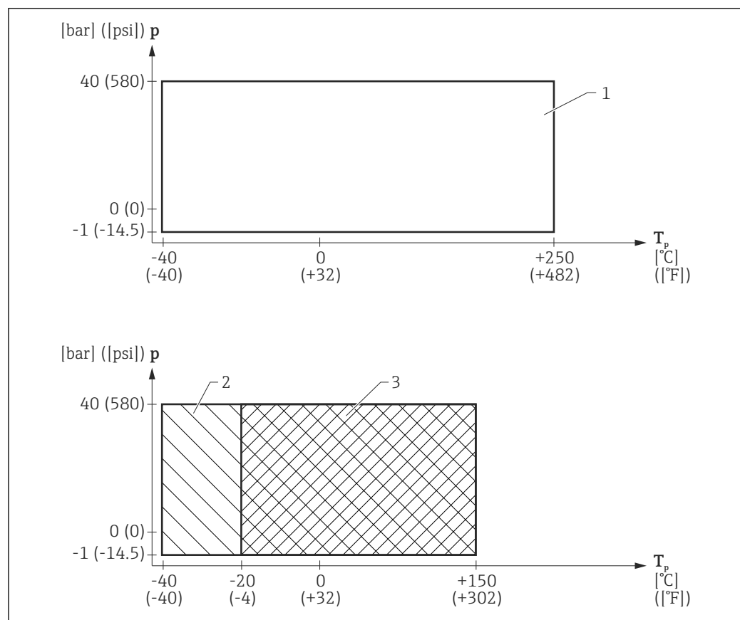
図 25 FMR51 : プロセス温度およびプロセス圧力の許容範囲
