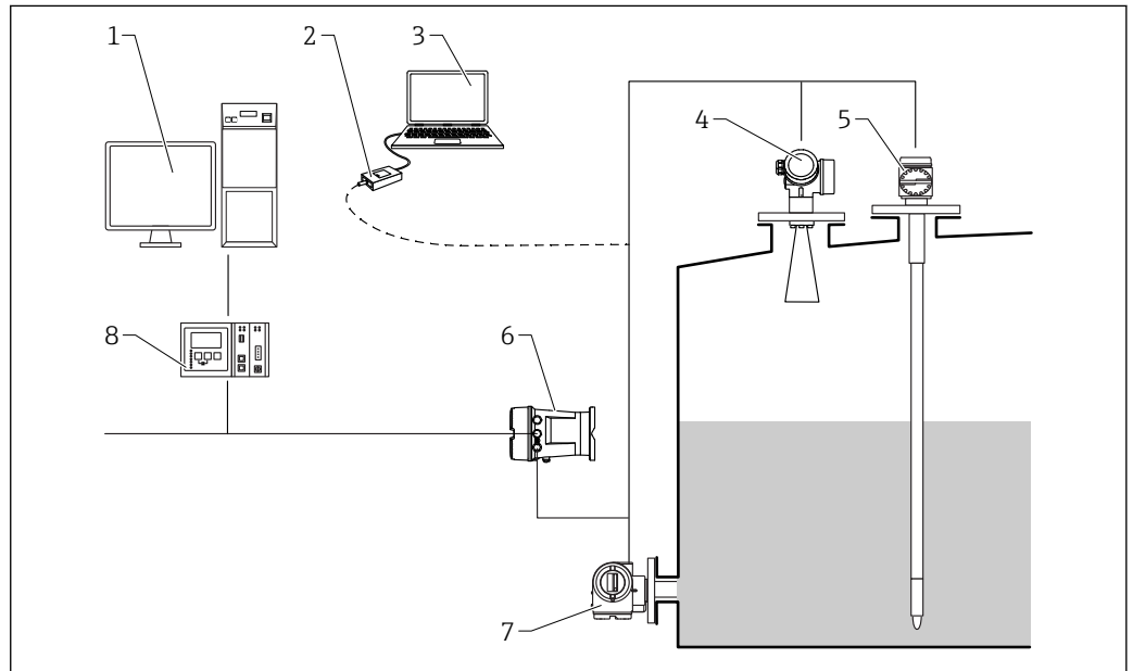
図 45 以下のコンポーネントで構成される計測システム
