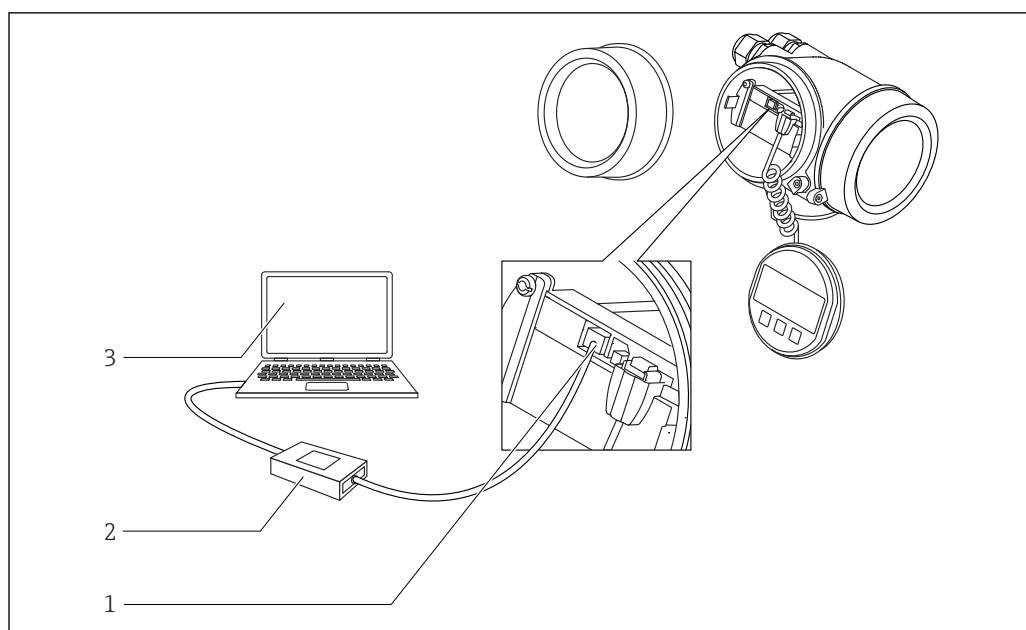
図 44 サービスインターフェイス（CDI）経由の DeviceCare/FieldCare
