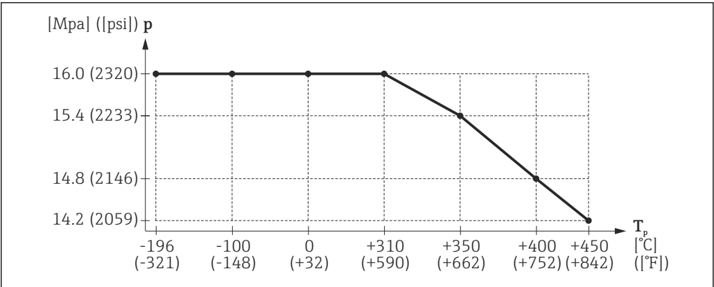
26 FMR51 : HT バージョンのプロセス温度およびプロセス圧力の許容範囲 (仕様コード 090「シール」、バージョン D2)
