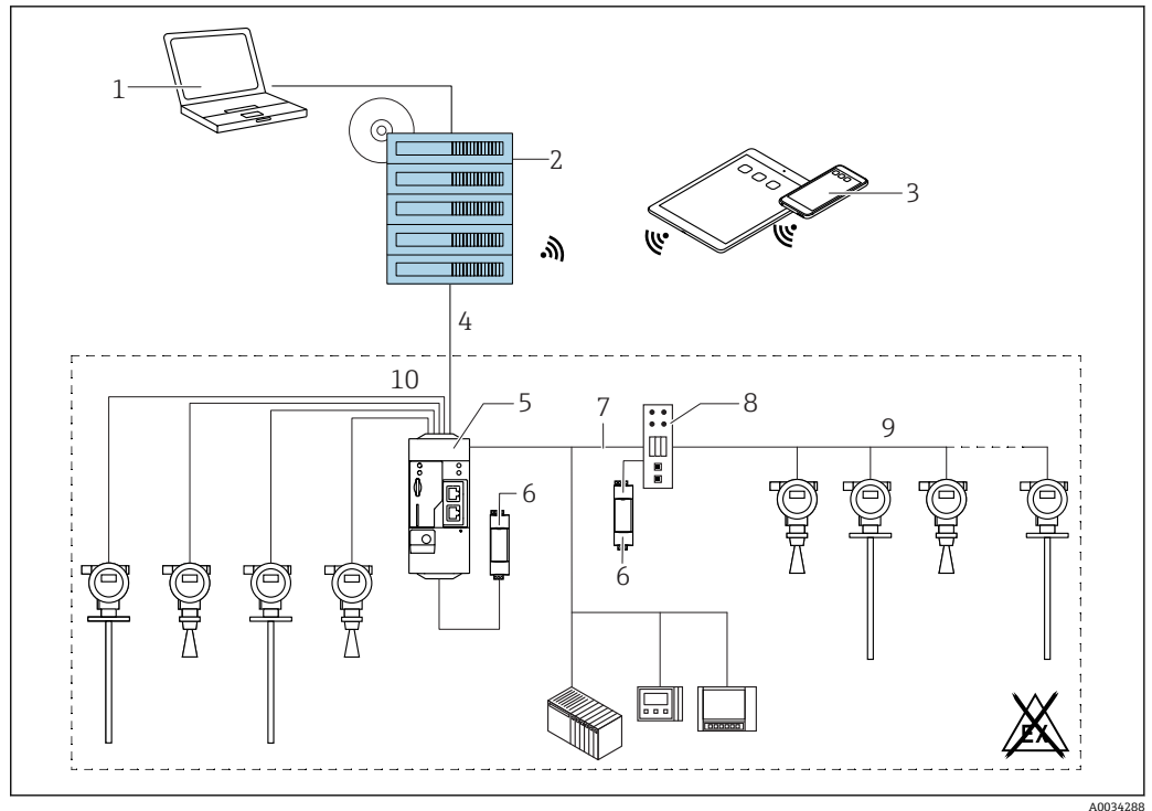
46 SupplyCare Enterprise SCE30B を使用した在槽管理プラットフォームの例
