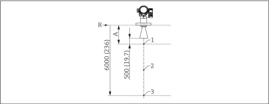
48 3 点リニアリティプロトコルの各点、使用単位 : mm (in)
