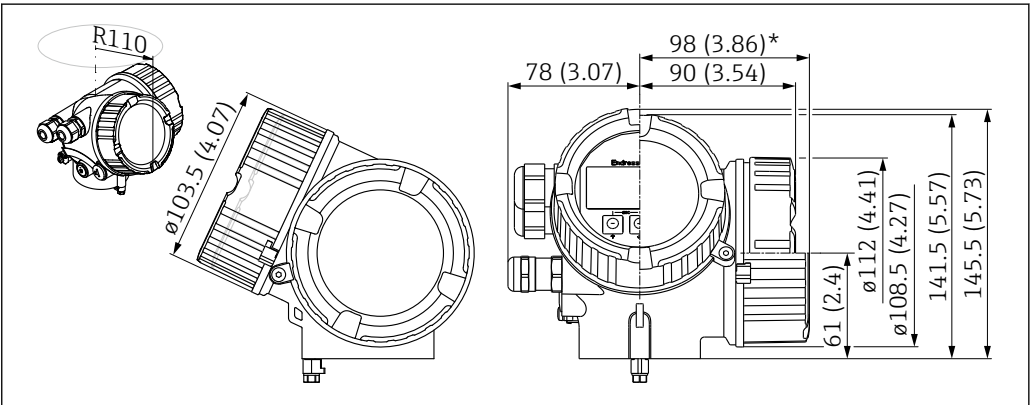
30 ハウジング GT20 (アルミダイカスト、塗装)。測定単位 mm (in)
