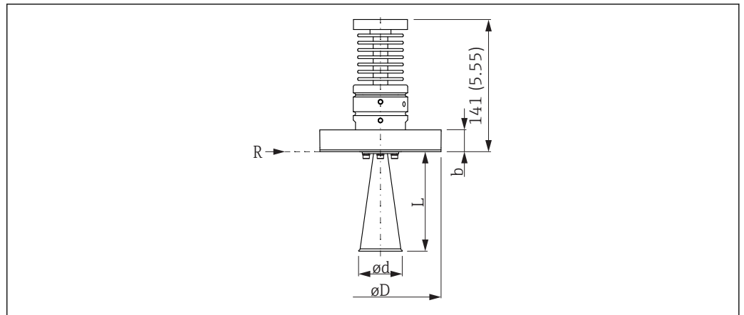
図 34 アンテナの寸法、バージョン T < 450 °C (842 °F)。測定単位 mm (in)
