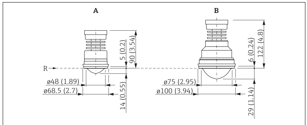
図 35 ミルクパイプ接続（DIN11851）付き機器の寸法。測定単位 mm (in)
