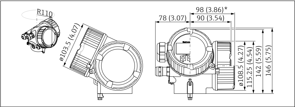
28 ハウジング GT18 (SUS 316L 相当)。測定単位 mm (in)
