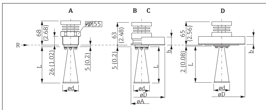
図 31 アンテナの寸法（伸長アンテナなしの場合）。測定単位 mm (in)
