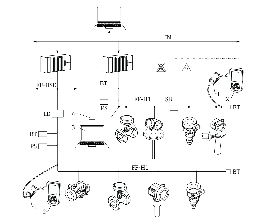
図 43 FOUNDATION フィールドバスシステム構成および関連するコンポーネント
