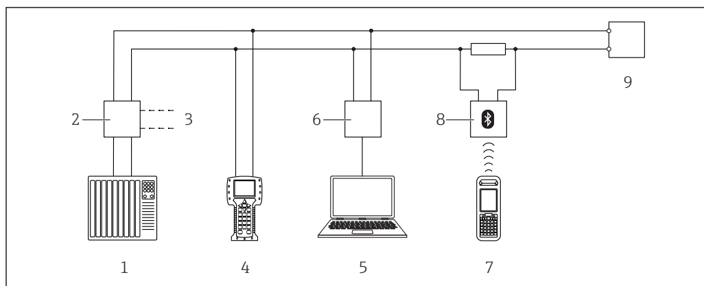
図 41 HART 経由のリモート操作用オプション
