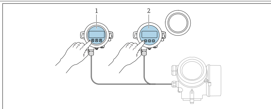
図 38 FHX50 操作オプション
