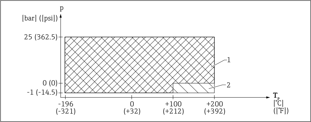
27 FMR52 : プロセス温度およびプロセス圧力の許容範囲
