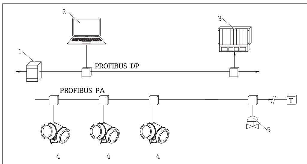
図 42 PROFIBUS PA プロトコルを介したリモート操作用のオプション
