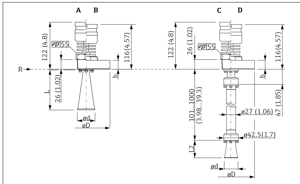
図 33 アンテナの寸法、バージョン T < 250 °C (482 °F)。測定単位 mm (in)
