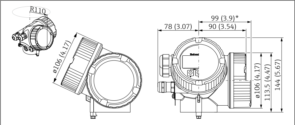
29 GT19 ハウジング (プラスチック PBT)。測定単位 mm (in)
