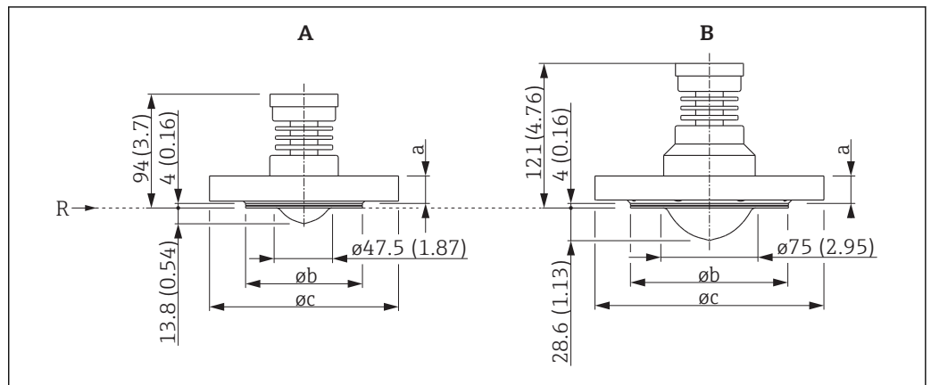
図 37 フランジ付き機器の寸法。測定単位 mm (in)
