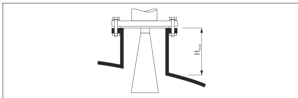
21 ホーンアンテナのノズル高 (FMR51)
