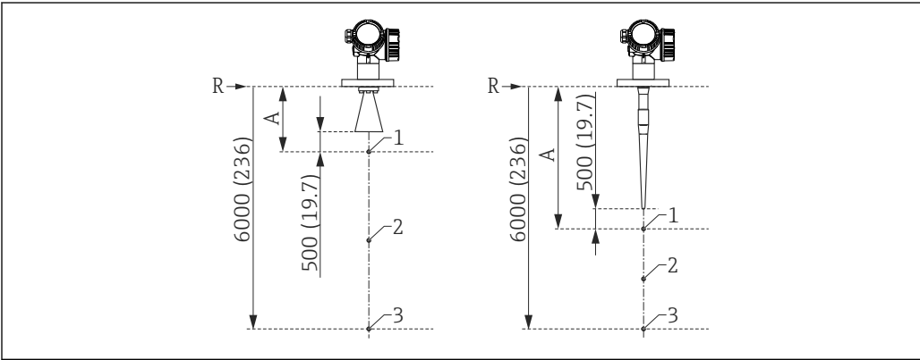
42 Pontos do protocolo de linearidade de 3 pontos; unidade de engenharia: mm (pol.)
