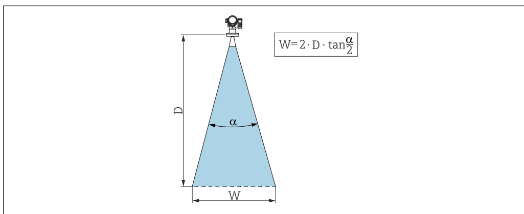
18 Relação entre o ângulo do feixe \alpha , a distância D e o diâmetro da largura do feixe W
