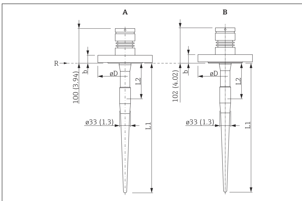
29 Dimensões do equipamento com flange. Unidade de medida mm (in)
