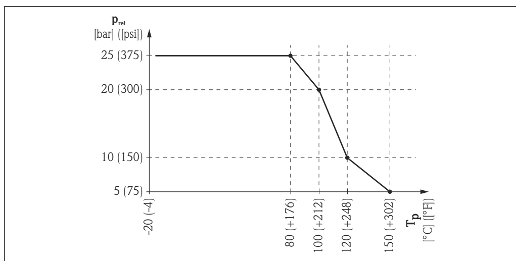
25 FMR54 com antena planar: Faixa permitida para temperatura do processo e pressão do processo
