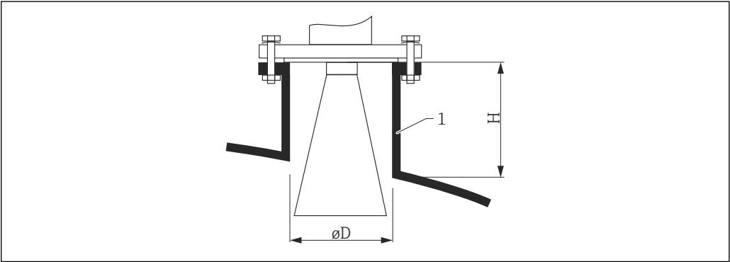
20 Altura e diâmetro do bocal para a antena piramidal
