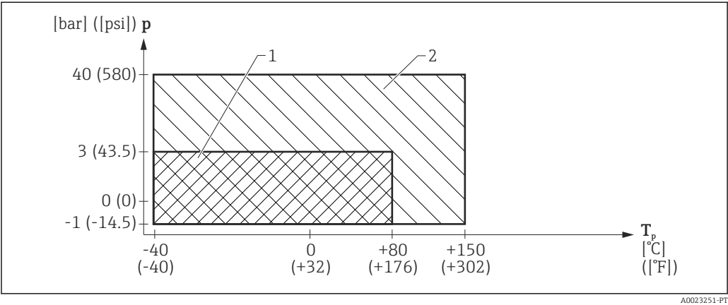
23 FMR53: Faixa permitida para temperatura do processo e pressão do processo
