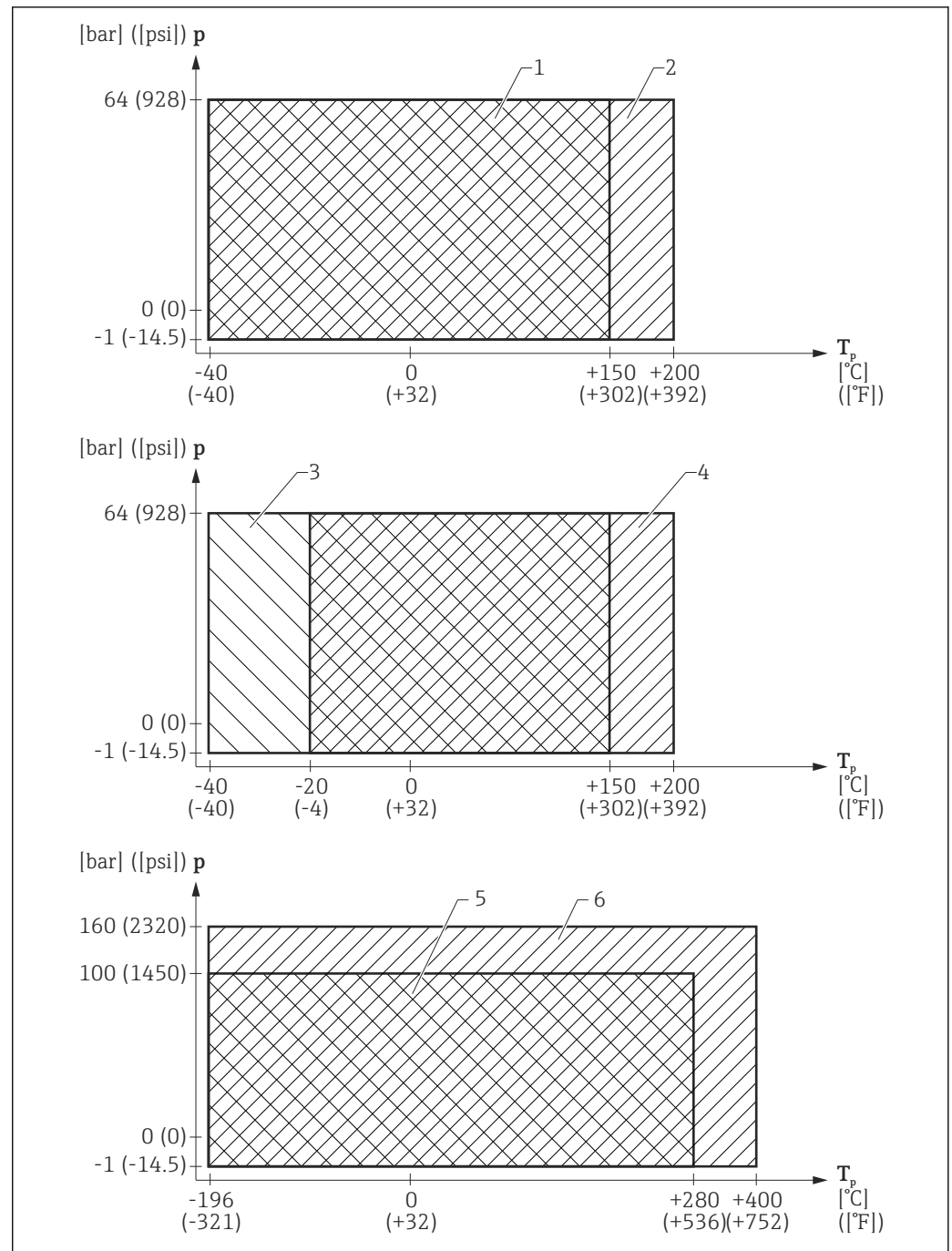
24 FMR54 com antena piramidal: Faixa permitida para temperatura do processo e pressão do processo
