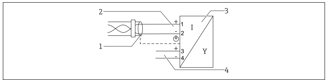
図 13 ブロック図：PROFIBUS PA / FOUNDATION フィールドバス
