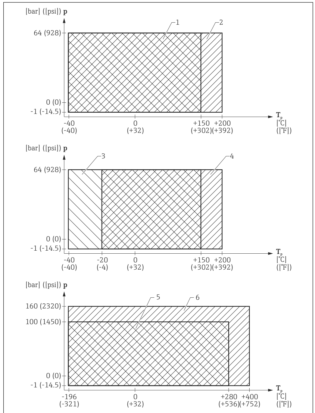
図 24 ホーンアンテナ付き FMR54 : プロセス温度およびプロセス圧力の許容範囲
