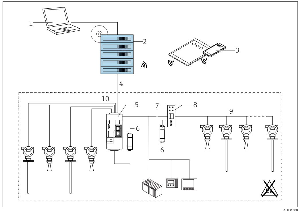
図 40 SupplyCare Enterprise SCE30B を使用した在槽管理プラットフォームの例
