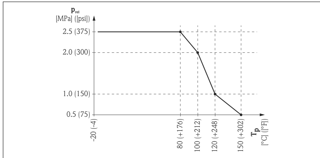
図 25 プレーナアンテナ付き FMR54 : プロセス温度およびプロセス圧力の許容範囲
