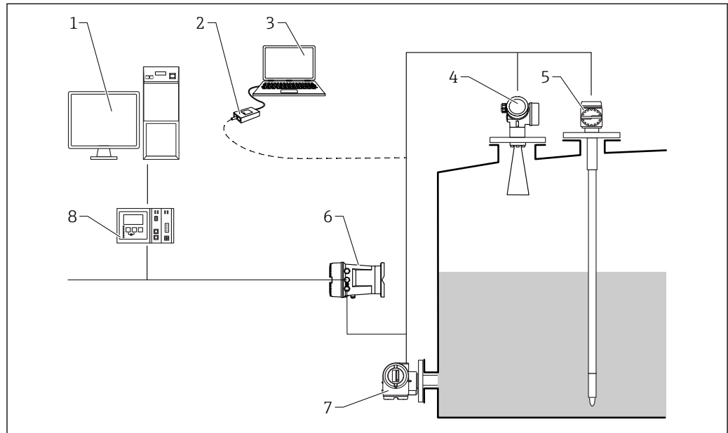
図 39 以下のコンポーネントで構成される計測システム
