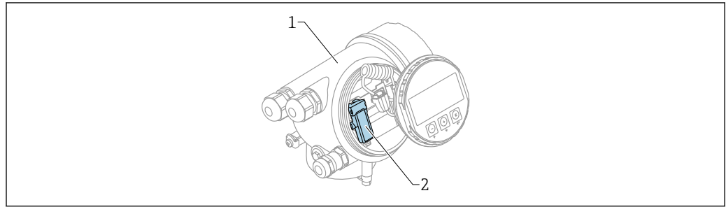
図 33 Bluetooth モジュール搭載の機器
