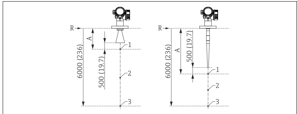
図 42 3点リニアリティプロトコルの各点、使用単位：mm (in)
