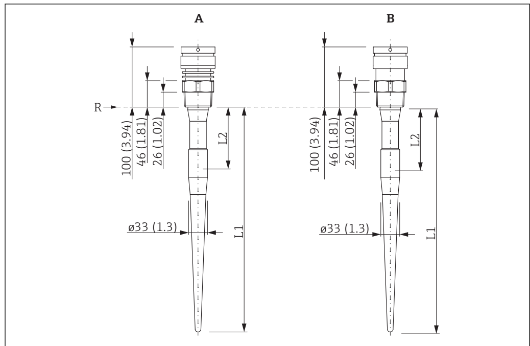
図 30 ネジ接続付き機器の寸法。測定単位 mm (in)
