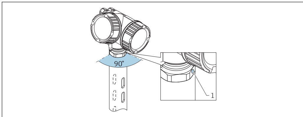
図 21 内筒管への設置
