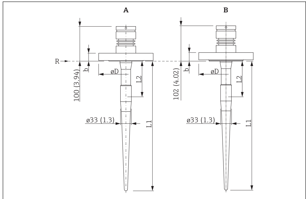
図 29 フランジ付き機器の寸法。測定単位 mm (in)
