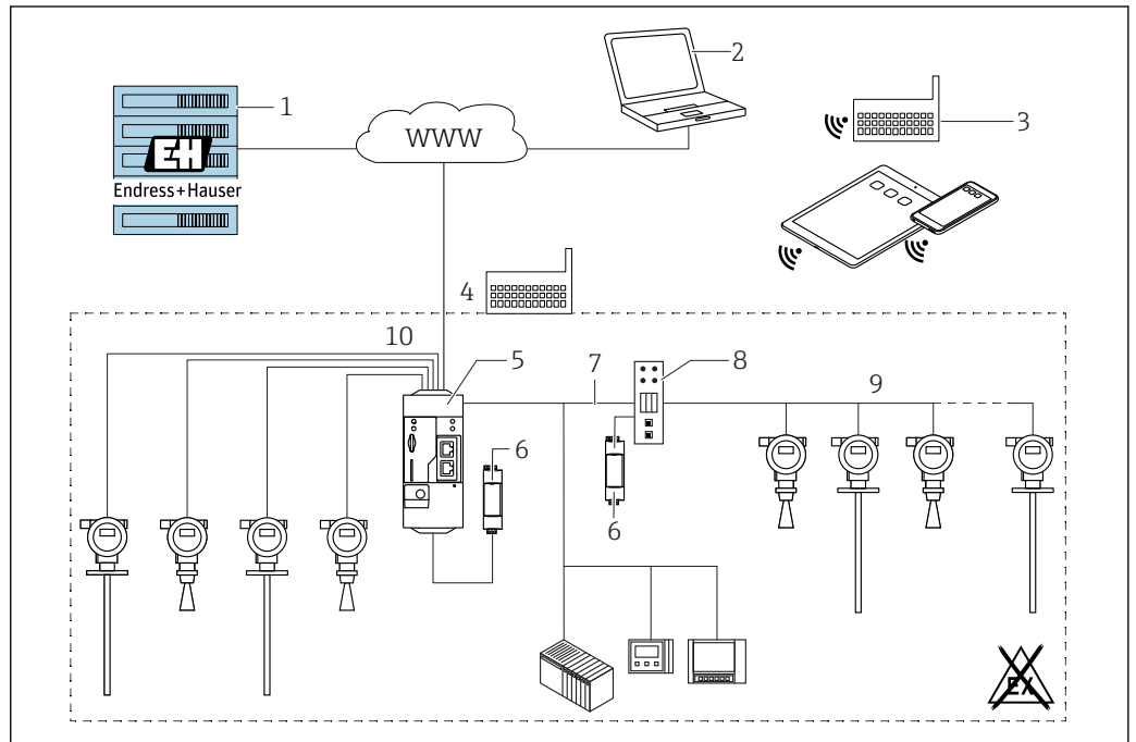
図 41 SupplyCare Hosting SCH30 を使用した在庫管理プラットフォームの例
