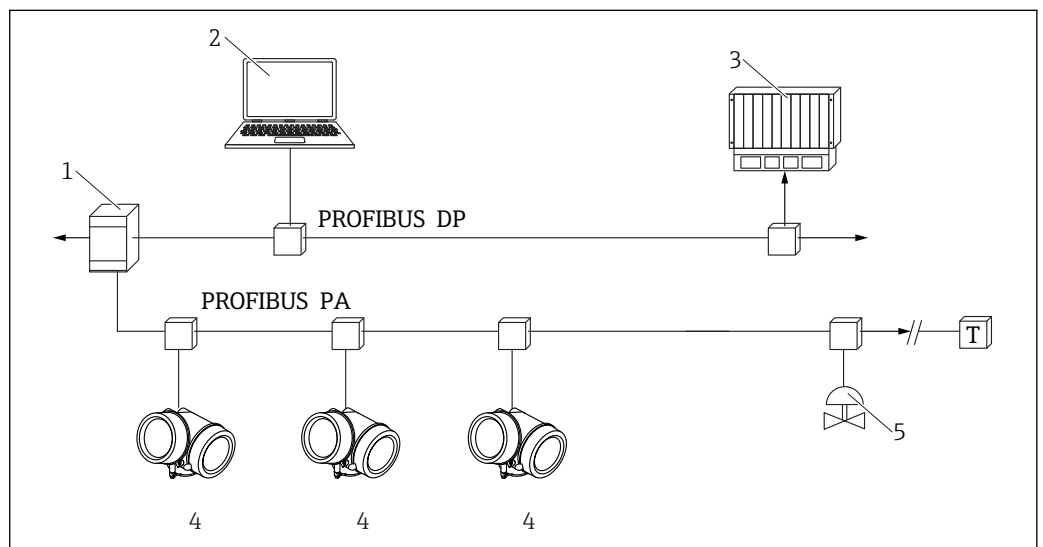
図 36 PROFIBUS PA プロトコルを介したリモート操作用のオプション
