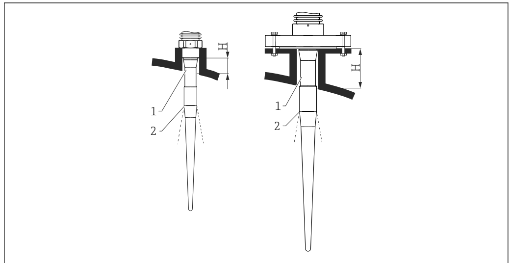
図 19 ロッドアンテナのノズル高 (FMR53)
