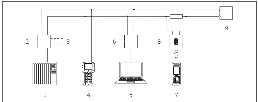
図 35 HART 経由のリモート操作用オプション
