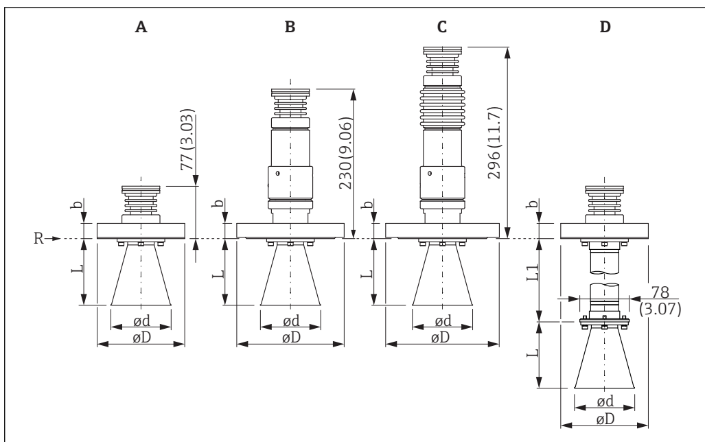
図 31 ホーンアンテナ付き FMR54 の寸法。測定単位 mm (in)
