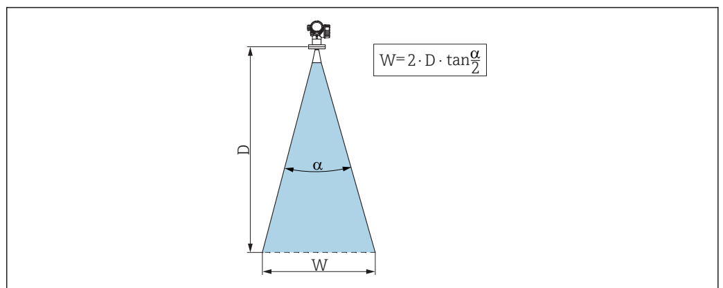
図 18 ビーム放射角 \alpha 、距離 D およびビーム幅 W の関係
