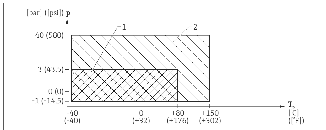
図 23 FMR53 : プロセス温度およびプロセス圧力の許容範囲
