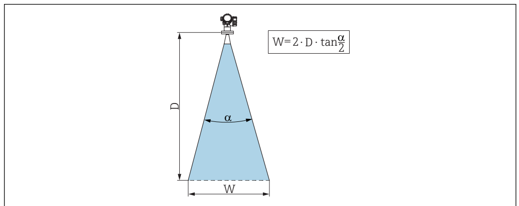
19 Rapporto tra angolo di emissione \alpha , distanza D e diametro del lobo di emissione W
