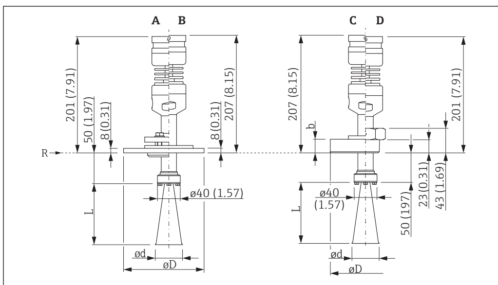
37 Dimensioni di FMR57 con antenna a cono - versione per alta temperatura; unità ingegneristica: mm (in)
