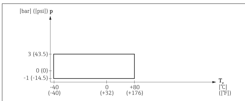
26 FMR56: campo consentito per temperatura e pressione di processo
