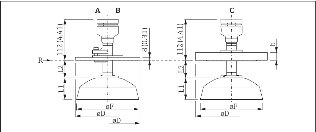
38 Dimensioni di FMR57 con antenna parabolica, unità ingegneristica: mm (in)
