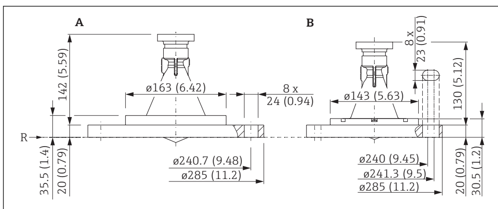
35 Dimensioni di FMR56 con flangia slip-on 6"/DN150. Unità di misura mm (in)
