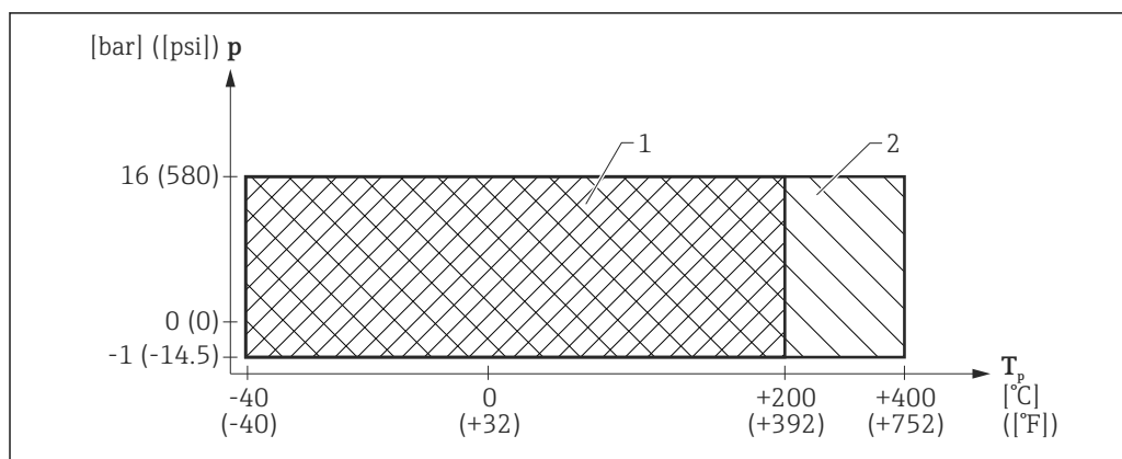
27 FMR57: campo consentito per temperatura e pressione di processo
