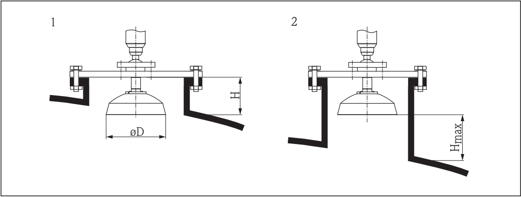
23 Montaggio del tronchetto del misuratore Micropilot FMR57 con antenna parabolica
