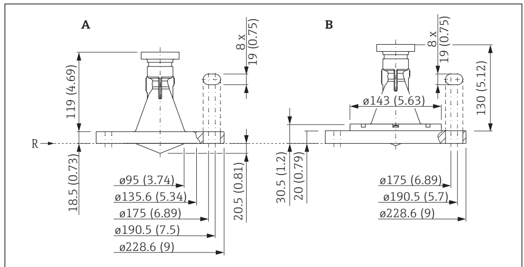
34 Dimensioni di FMR56 con flangia slip-on 4"/DN100. Unità di misura mm (in)
