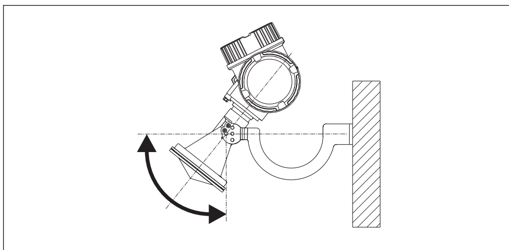
21 Montaggio dell'antenna a cono con staffa di montaggio
