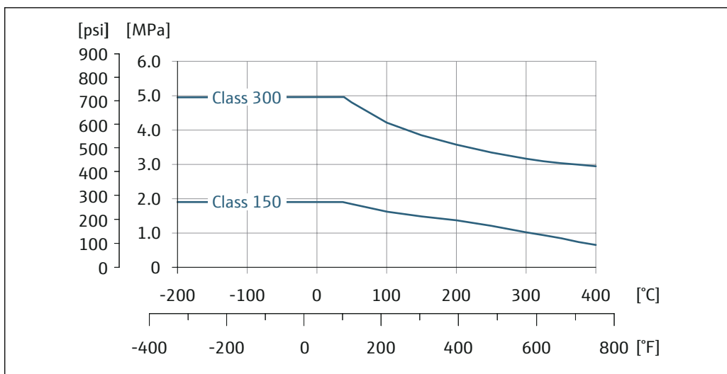
図 18 フランジ接続材質：ステンレス、複数の認証、1.4404/SUS F316 または F316L 相当
