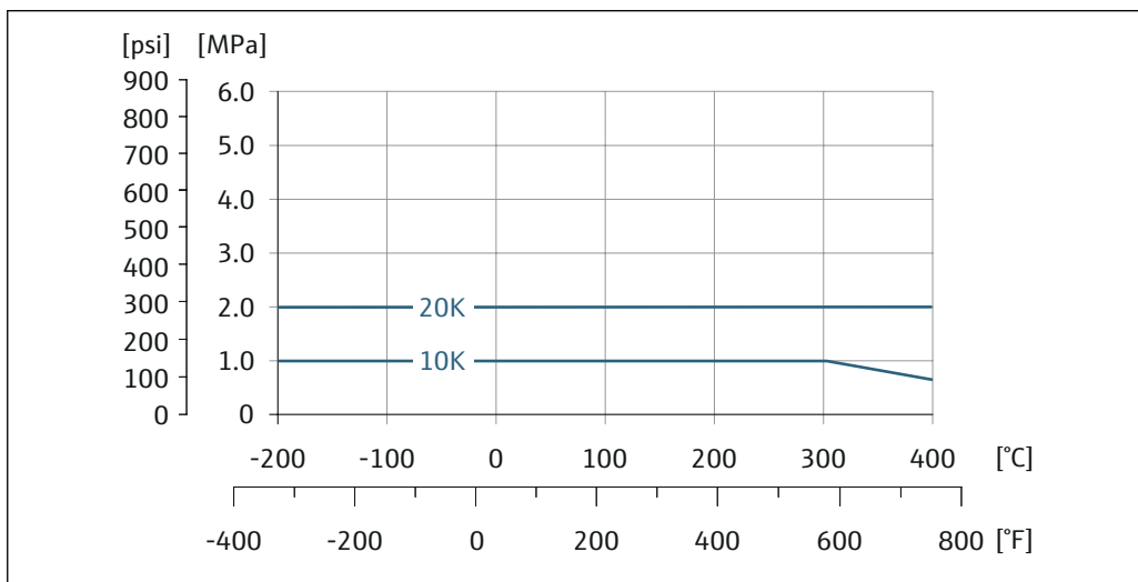
図 19 フランジ接続材質：ステンレス、複数の認証、1.4404/SUS F316 または F316L 相当
