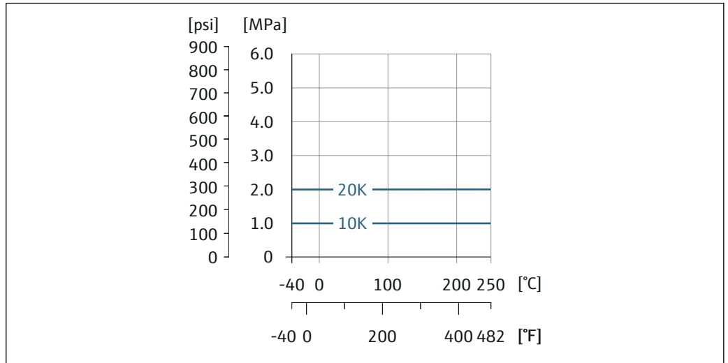
図 22 フランジ接続材質 : 鋳造アロイ、CX2MW (アロイ C22/2.4602 と同等)
