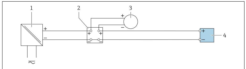
図 10 4~20 mA 電流入力の接続例
