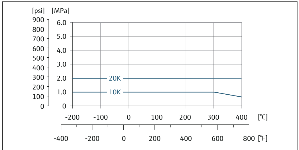
図 21 フランジ接続材質 : ステンレス、複数の認証、1.4404/SUS F316 または F316L 相当
