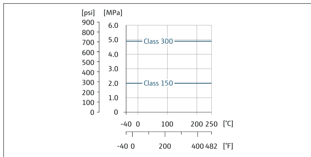
図 20 フランジ接続材質：鋳造アロイ、CX2MW (アロイ C22/2.4602 と同等)
