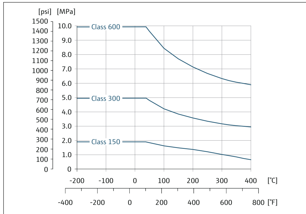
図 19 フランジ接続材質：ステンレス、複数の認証、1.4404/SUS F316 または F316L 相当
