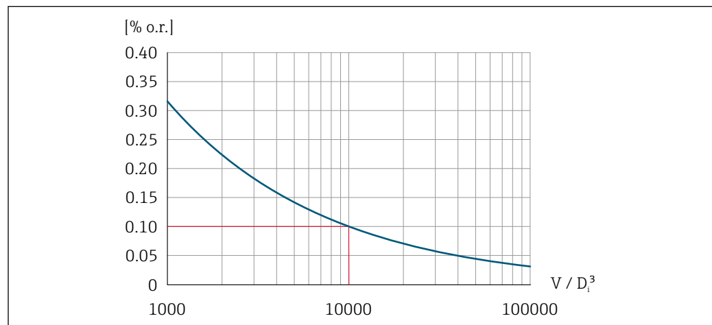
図 12 繰返し性 = 0.1 % o.r.、V = 10000 × D i 3 の体積測定値 [m 3 ] において
