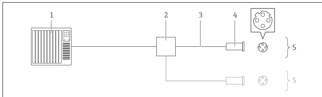
図 15 PROFINET の接続ケーブル
