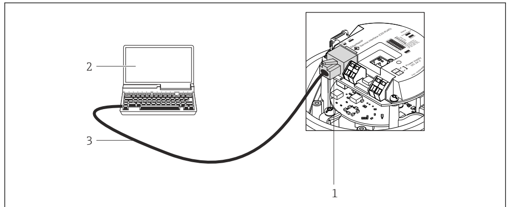
☒ 41 「出力」のオーダーコードの接続、オプション L : PROFIBUS DP
