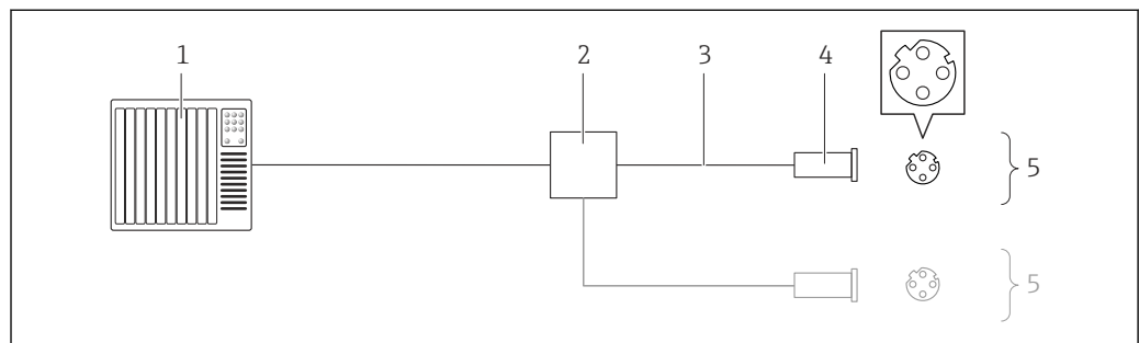
図 14 EtherNet/IP の接続例
