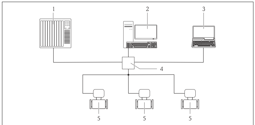
図 38 Ethernet ベースのフィールドバス経由のリモート操作オプション
