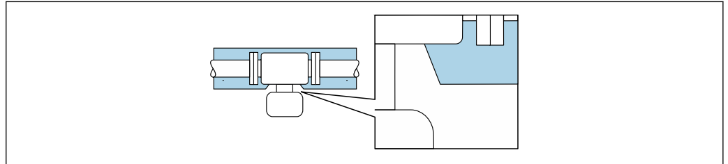
図 32 伸長ネックを覆わない断熱：
