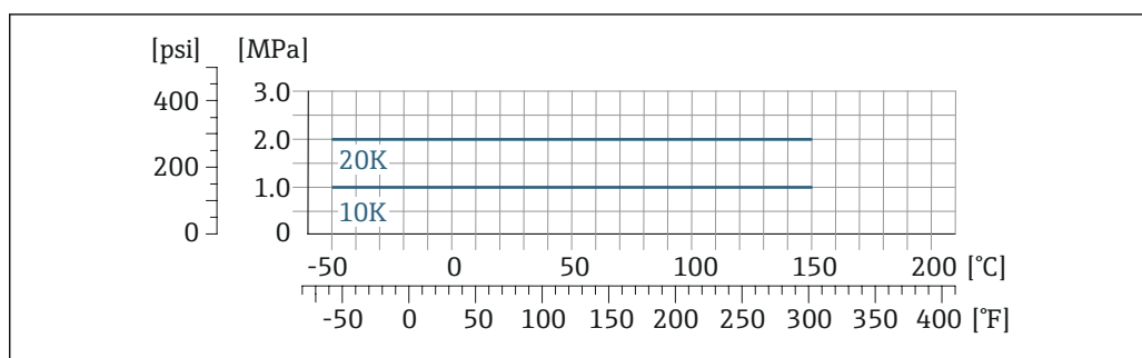
図 25 フランジ材質 1.4404 (SUS F316 または F316L 相当)
