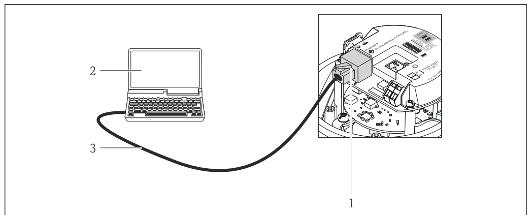
☒ 42 「出力」のオーダーコードの接続、オプション N : EtherNet/IP
