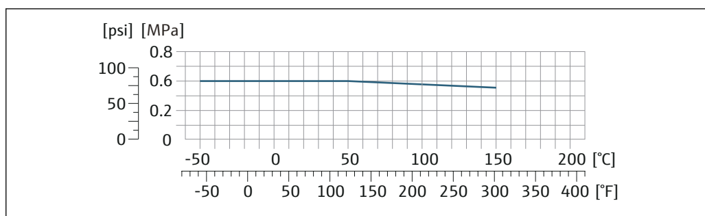
図 30 接続部の材質 1.4435 (SUS 316L 相当)
