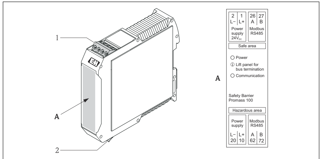
図 7 Promass 100 安全バリア、端子付き
