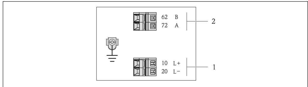
図 4 Modbus RS485 端子の割当て、本質安全区域用の接続の種類 (Promass 100 安全バリアを介した接続)
