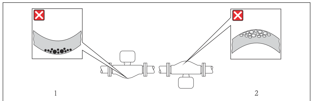
☒ 19 弓形計測チューブセンサの取付方向
