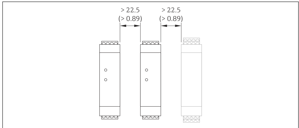
図 20 Promass 100 安全バリアまたはその他のモジュールとの最小距離。単位 mm (in)
