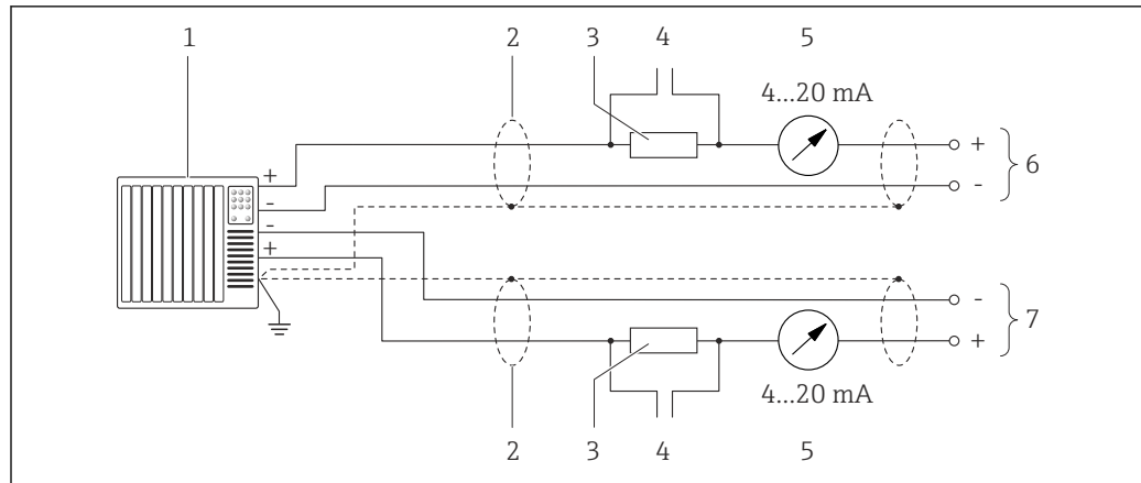
図 17 電流入力（アクティブ）を介した HART 入力（マスタモード）の接続例
