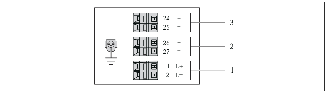
㉔ 1 端子の割当て 4 ~ 20 mA HART、パルス/周波数/スイッチ出力付き
