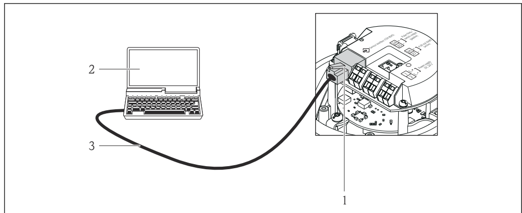
図 40 「出力」のオーダーコードの接続、オプション B：4～20 mA HART、パルス/周波数/スイッチ出力
