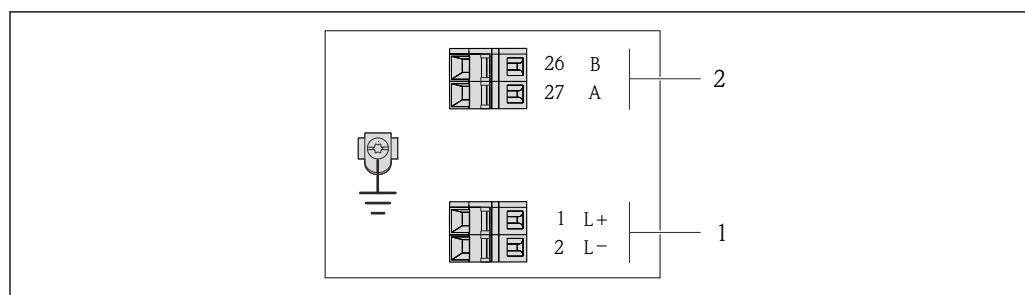
図 2 PROFIBUS DP 端子の割当て
