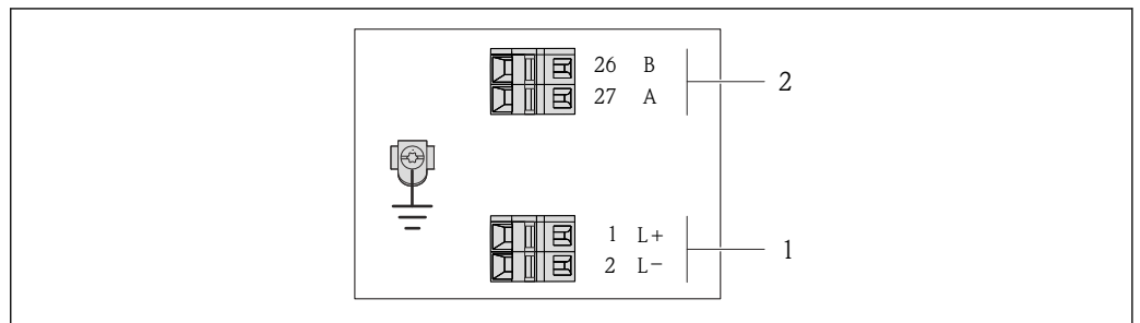
図 3 Modbus RS485 端子の割当て、非危険場所および Zone 2/Div. 2 用の接続の種類
