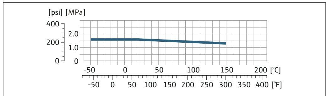
図 29 接続部の材質 1.4435 (SUS 316L 相当)
