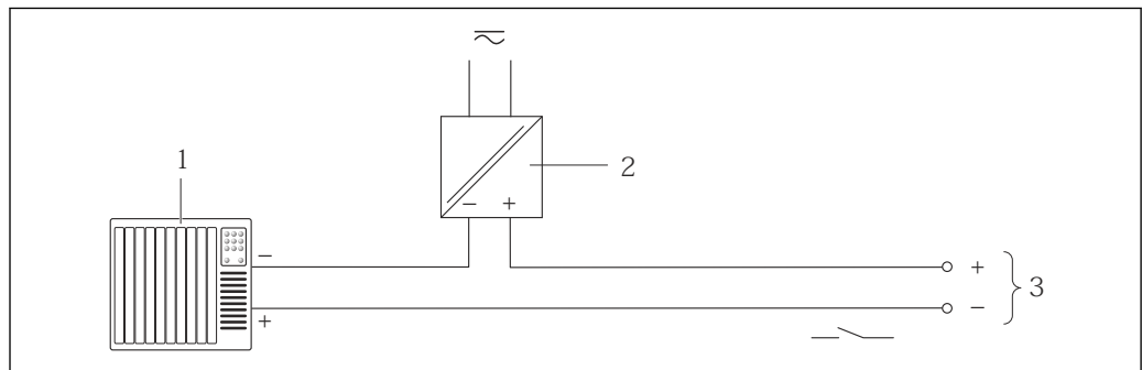
図 10 スイッチ出力（パッシブ）の接続例
