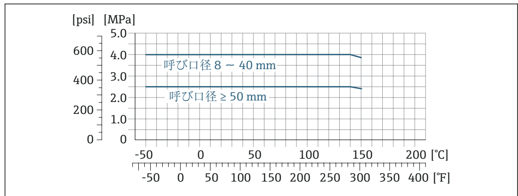
図 28 接続部の材質 1.4435 (SUS 316L 相当)
