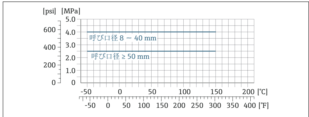
図 27 フランジ材質 1.4435 (SUS 316L 相当)
