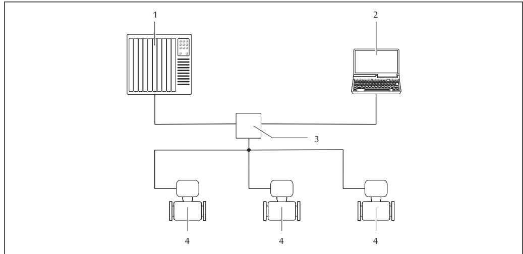
図 39 PROFINET ネットワーク経由のリモート操作オプション
