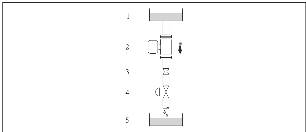
図 18 下り方向の垂直配管での設置（例: バッチアプリケーション用）
