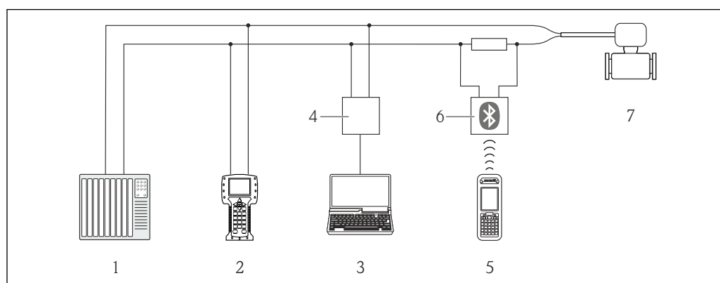
図 36 HART 経由のリモート操作オプション
