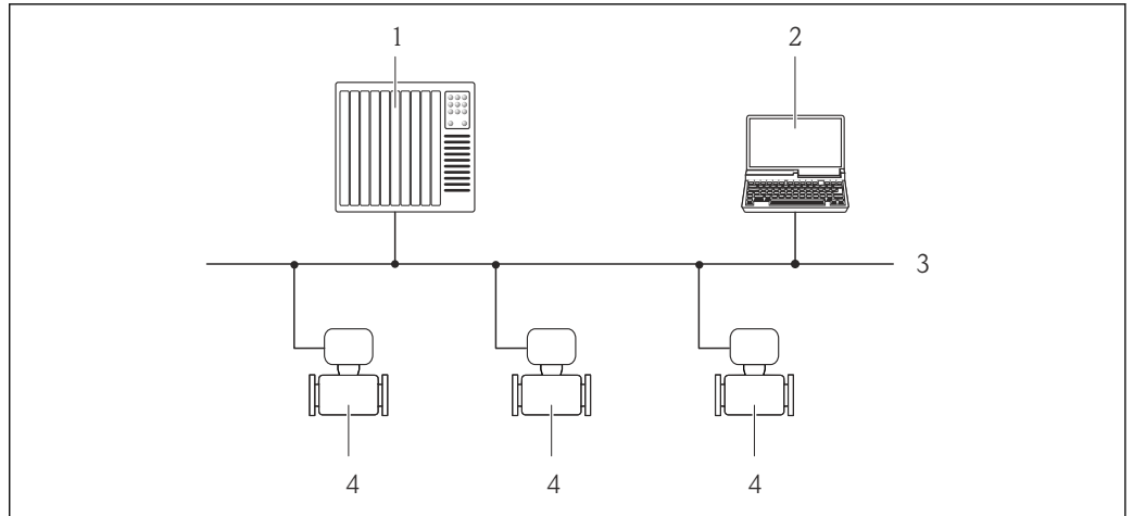
図 37 PROFIBUS DP ネットワークを介したリモート操作のオプション
