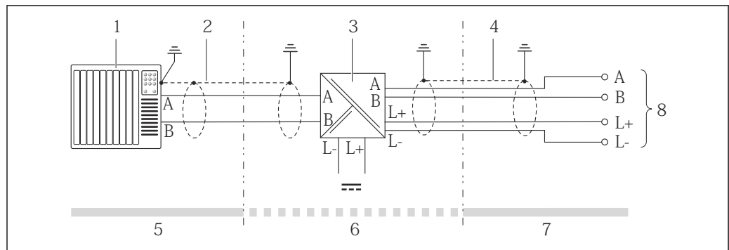
図 13 Modbus RS485 (本质安全) の接続例
