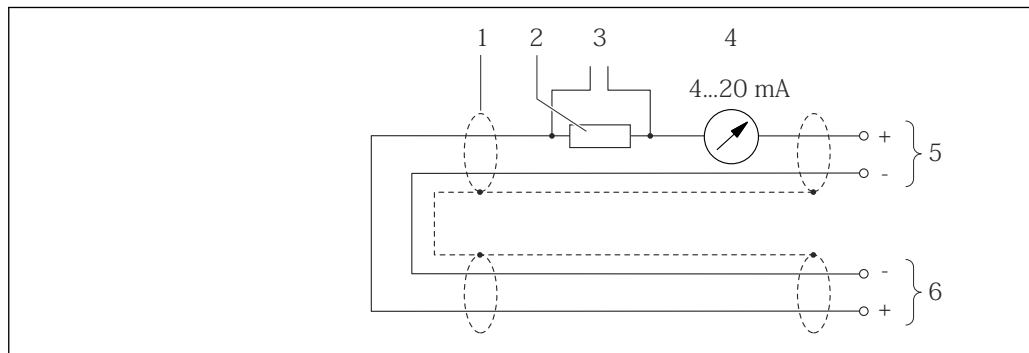
図 16 電流入力 (アクティブ) を介した HART 入力 (バーストモード) の接続例
