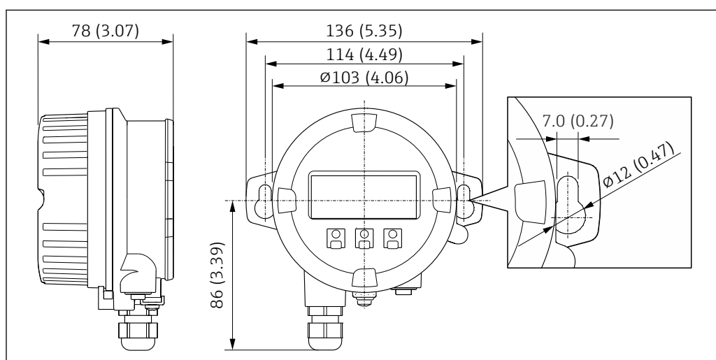
図 36 単位 mm (in)
