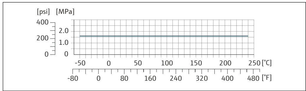
図 30 接続部の材質 1.4404 (SUS 316/316L 相当)
