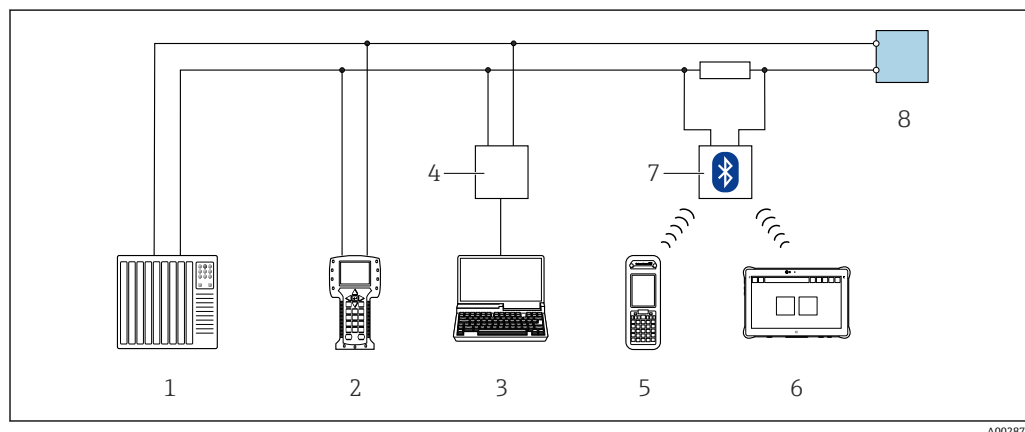
図 47 HART プロトコル経由のリモート操作オプション (アクティブ)
