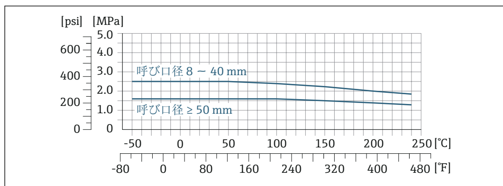
図 28 接続部の材質 1.4404 (SUS 316/316L 相当)
