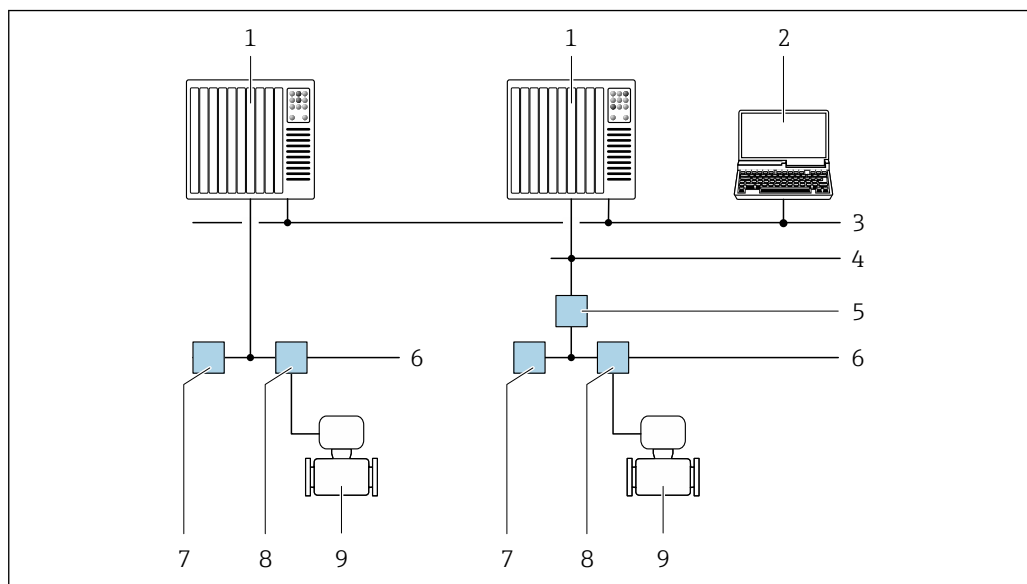
図 49 FOUNDATION フィールドバスネットワークを介したリモート操作用のオプション
