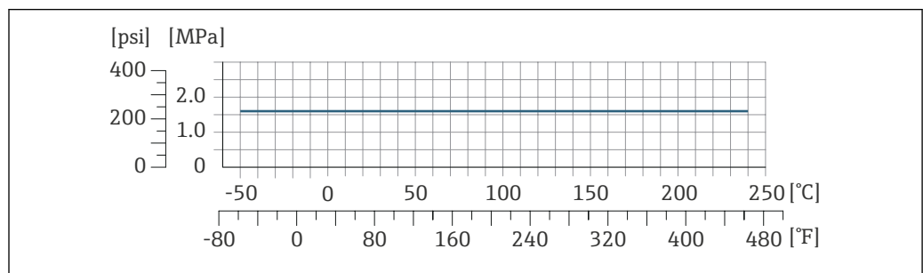
図 31 接続部の材質 1.4404 (SUS 316/316L 相当)
