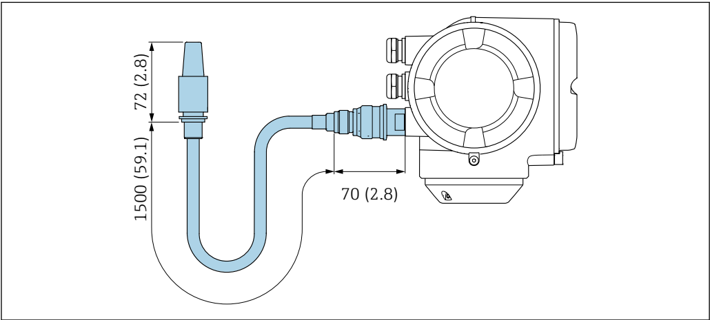
図 43 単位 mm (in)
