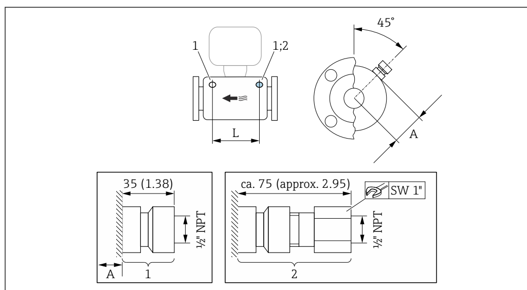
39 単位 mm (in)
