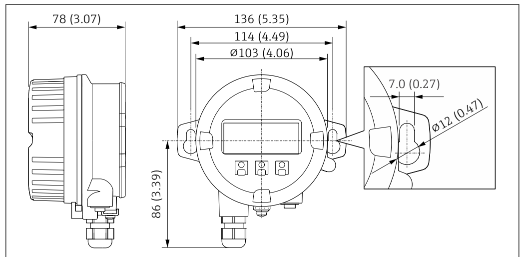
41 単位 mm (in)
