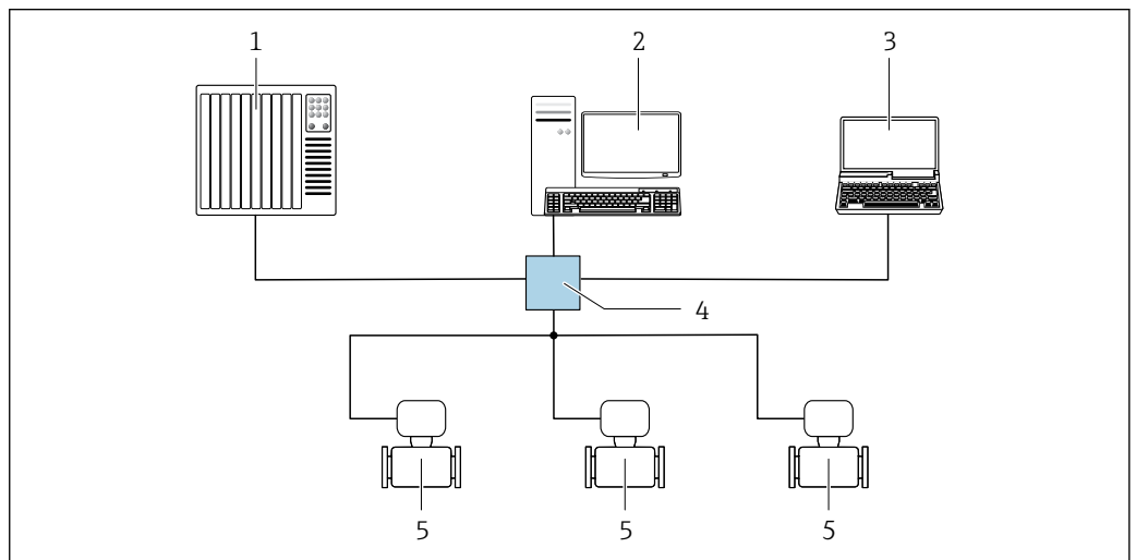
図 53 EtherNet/IP ネットワーク経由のリモート操作オプション：スター型トポロジー
