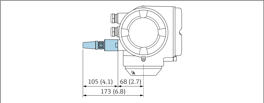
図 42 単位 mm (in)
