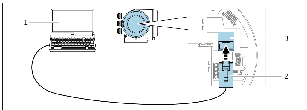
図 57 サービスインターフェイス（CDI-RJ45）経由の接続
