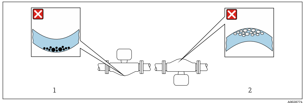
図 22 弓形計測チューブセンサの取付方向
