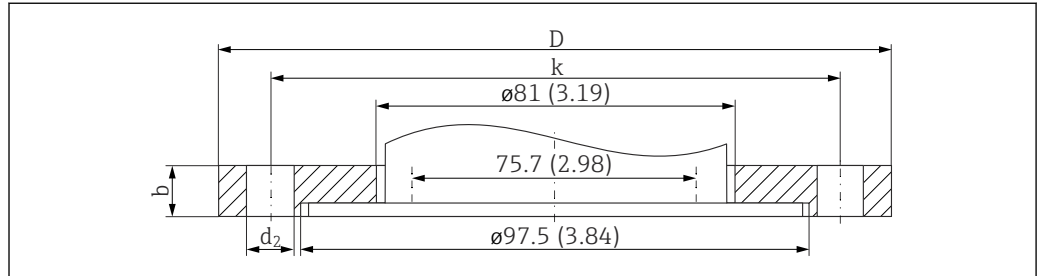
図 8 FAU80 スリップオンフランジの寸法（アダプタフランジなし）。測定単位 mm (in)
