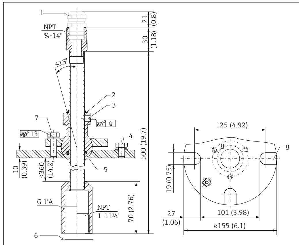
図 14 FAU40 角度調節器。測定単位 mm (in)
