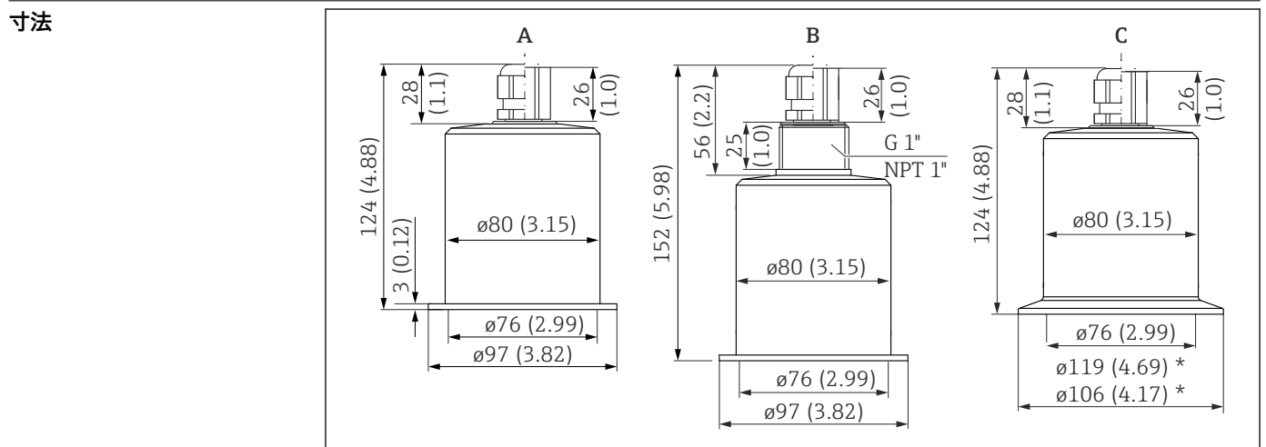
図 10 寸法。測定単位 mm (in)
