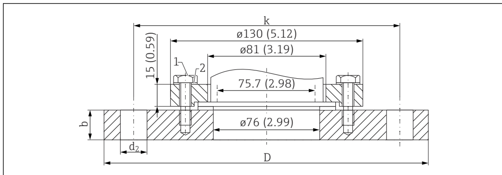
図 9 FAU80 スリップオンフランジの寸法（アダプタフランジ付き）。測定単位 mm (in)
