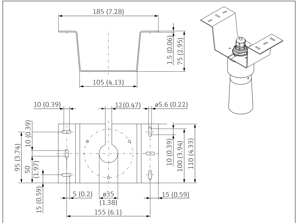
図 13 天井取付け用の取付ブラケット。測定単位 mm (in)
