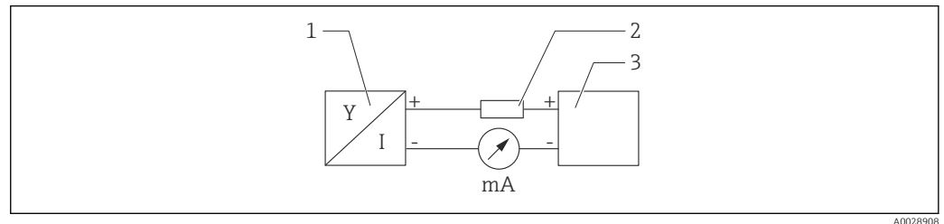
1 Schemat blokowy podłączenia wersji HART
