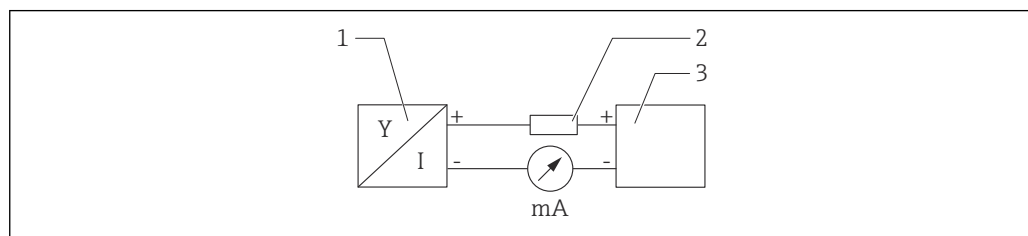
1 Schemat blokowy podłączenia wersji HART
