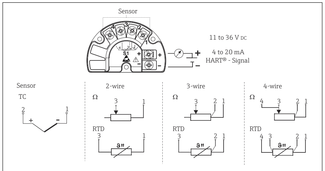
3 Conectando o transmissor
