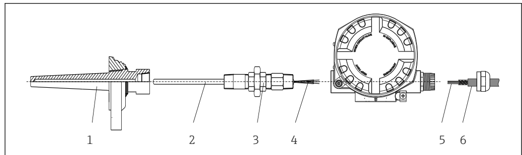
5 Montagem direta do transmissor de campo no sensor
