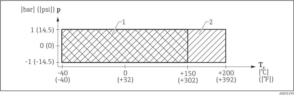
20 FMR67: Rango admisible para la temperatura del proceso y la presión del proceso, antena, PTFE DN80, brida UNI 316L
