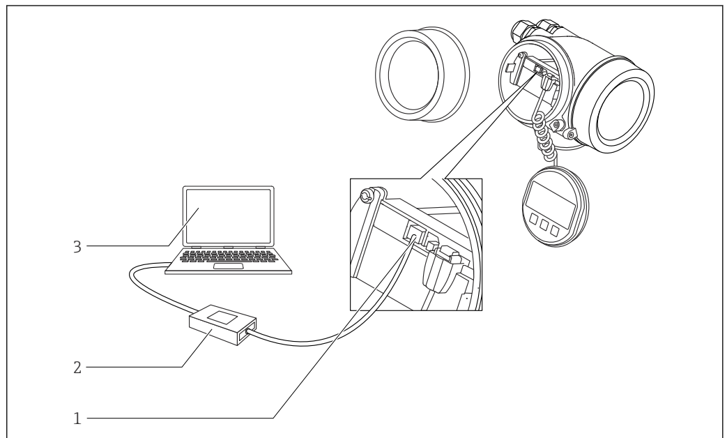
38 DeviceCare/FieldCare mediante interfaz de servicio (CDI)
