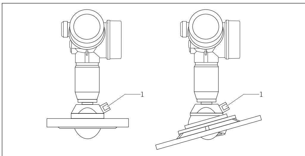
17 Conexión integrada de aire de purga para antenas de montaje enrasado
