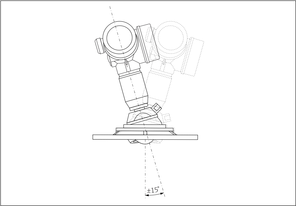
15 Micropilot FMR67 con unidad de alineación
