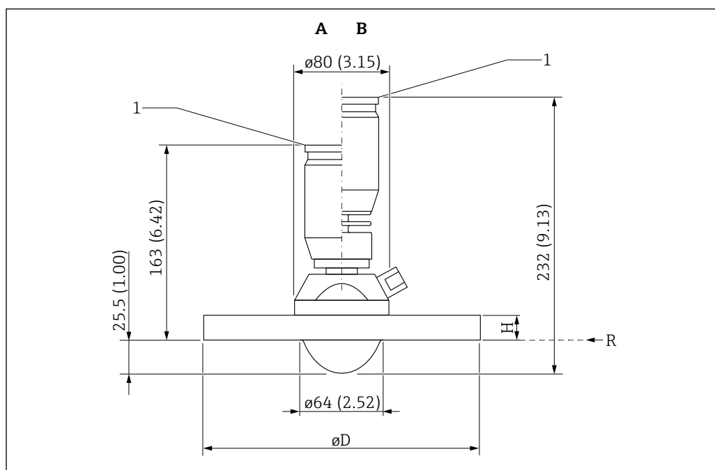
29 Medidas de la antena de montaje enrasado con brida estándar y conexión de aire de purga . Unidad de medida mm (in)
