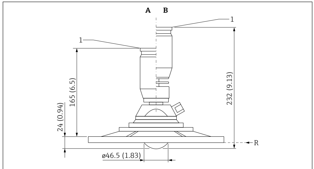
32 Medidas de la antena con brida UNI, unidad de alineación y conexión de aire de purga. Unidad de medida mm (in)
