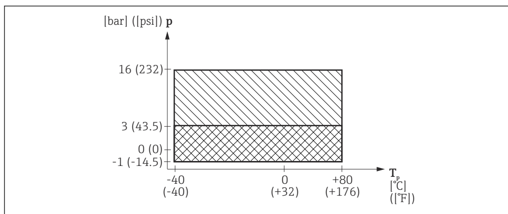
18 FMR67: Rango admisible para la temperatura del proceso y la presión del proceso, antena de goteo, PTFE DN50
