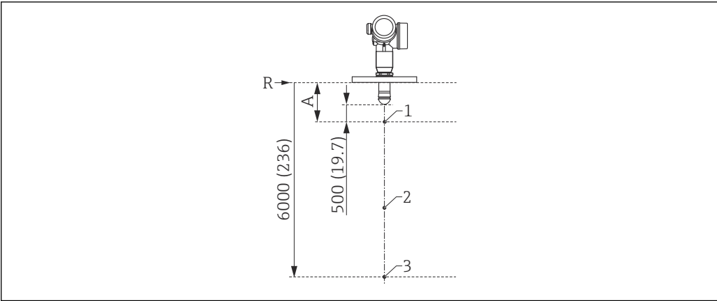
41 Puntos del protocolo de linealización a 3 puntos. Unidad de medida mm (in)
