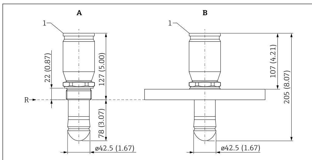
25 Medidas de la antena de goteo, sin conexión de aire de purga. Unidad de medida mm (in)
