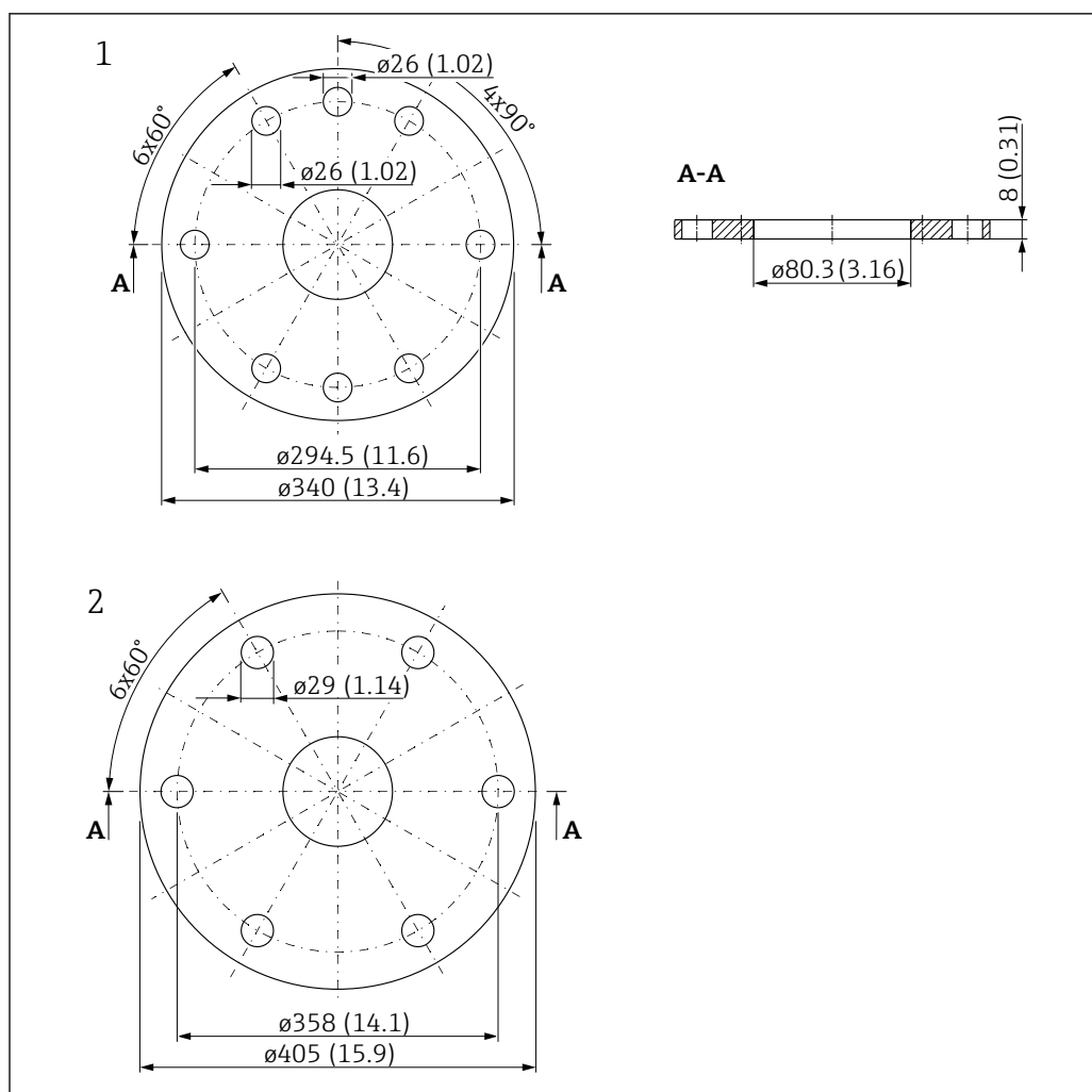
31 Medidas de la brida UNI para FMR67 con conexión de aire de purga. Unidad de medida mm (in)
