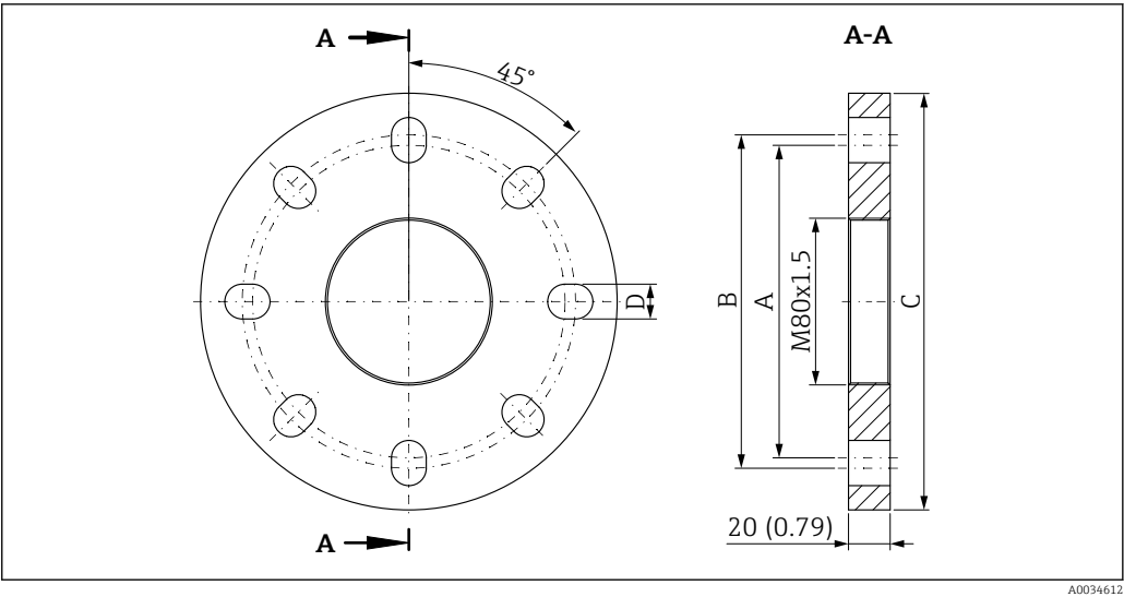
28 Medidas de las bridas UNI para FMR67 con conexión de aire de purga. Unidad de medida mm (in)
