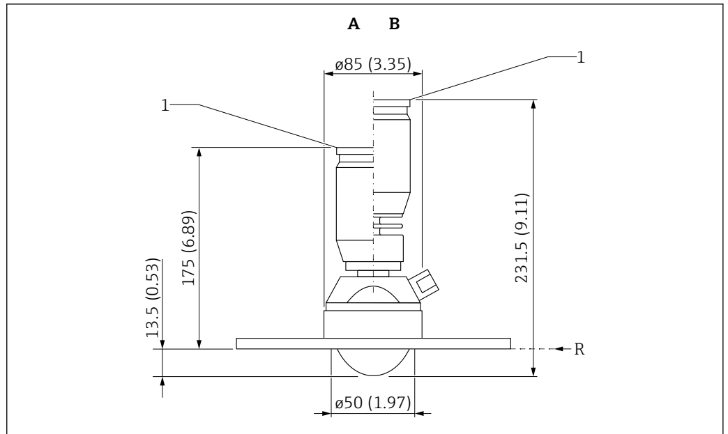
30 Medidas de la antena con brida UNI y conexión de aire de purga. Unidad de medida mm (in)
