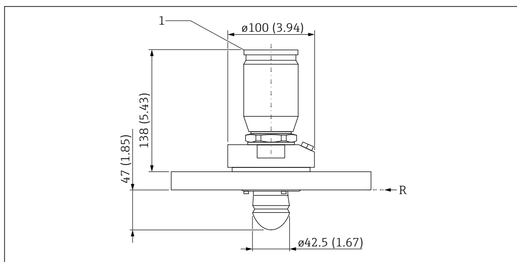
27 Medidas de la antena de goteo, conexión de aire de purga. Unidad de medida mm (in)
