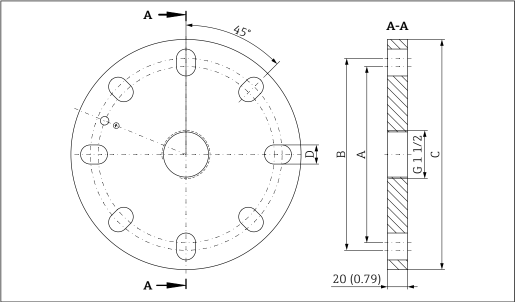
26 Medidas de las bridas UNI para FMR67 sin conexión de aire de purga. Unidad de medida mm (in)
