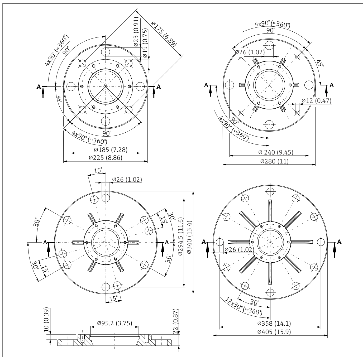
33 Medidas de las bridas UNI para FMR67 con unidad de alineación y conexión de aire de purga. Unidad de medida mm (in)
