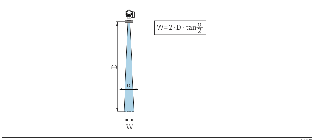
14 Relación entre el ángulo de apertura del haz \alpha , la distancia D y el diámetro del ancho del haz W
