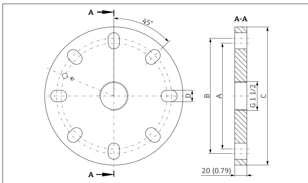
20 Dimensioni: mm (in)
