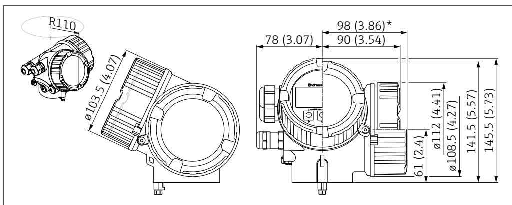
■ 18 Custodia GT20 (con rivestimento alluminio). Unità di misura mm (in)
