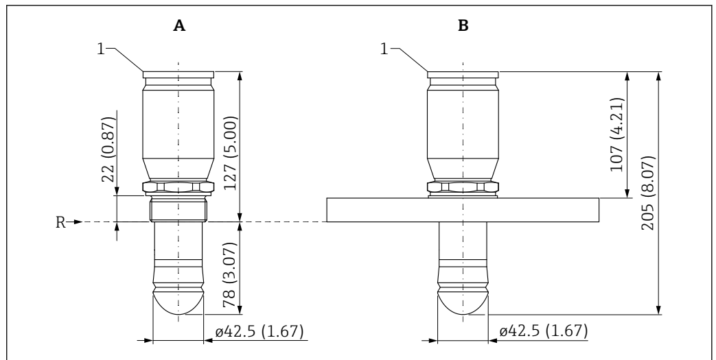
19 Dimensioni: mm (in)
