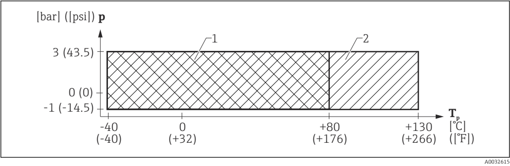
16 FMR60: campo consentito per temperatura e pressione di processo
