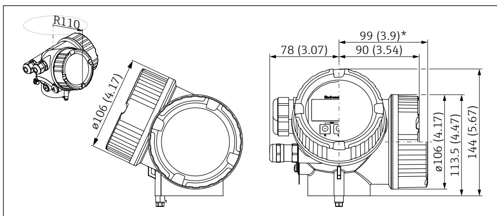
■ 17 Custodia GT19 (plastica PBT). Unità di misura mm (in)
