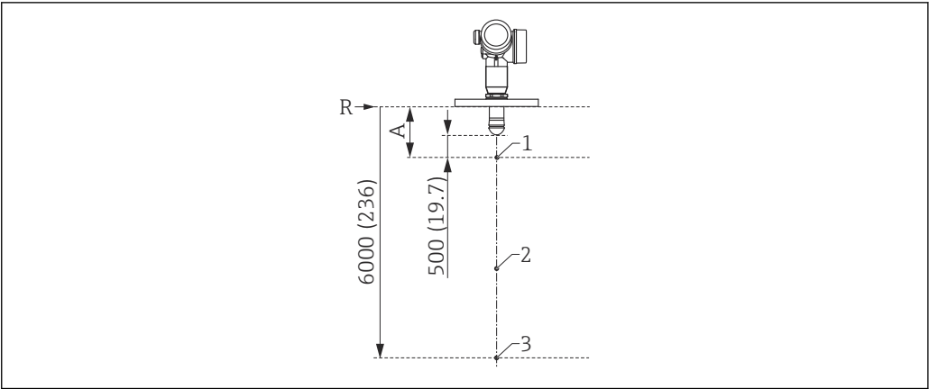
28 Punti del protocollo di linearità a 3 punti. Unità di misura mm (in)
