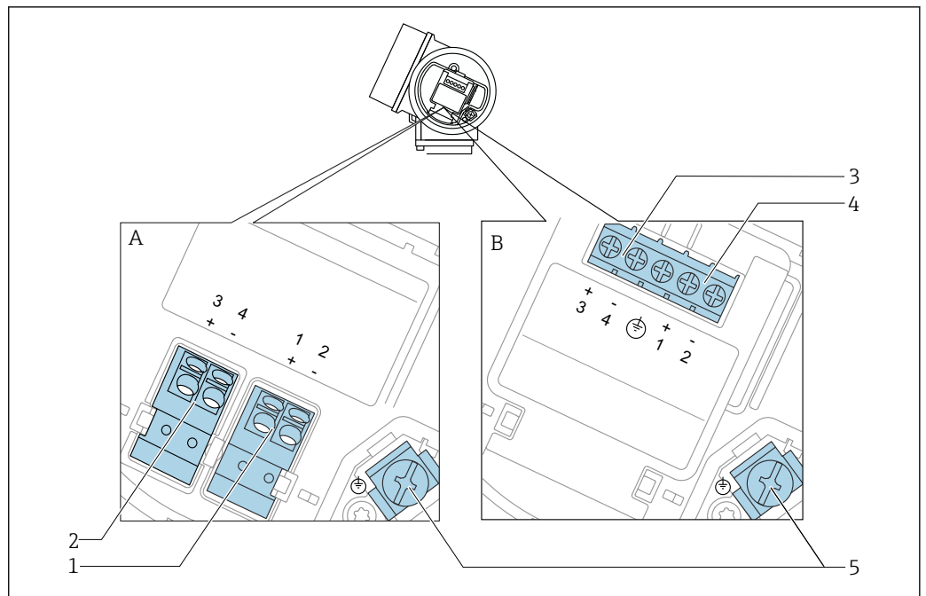
7 Asignación de terminales a 2 hilos: 4-20 mA HART, 4-20 mA
