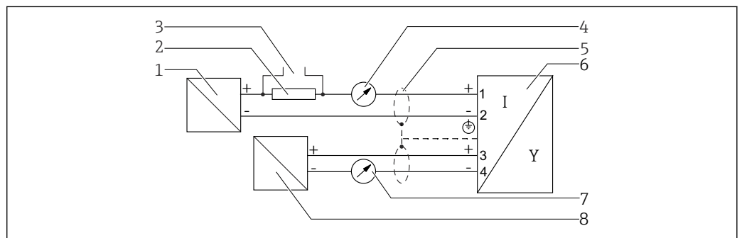
8 Diagrama en bloque a dos hilos: 4-20 mA HART, 4-20 mA
