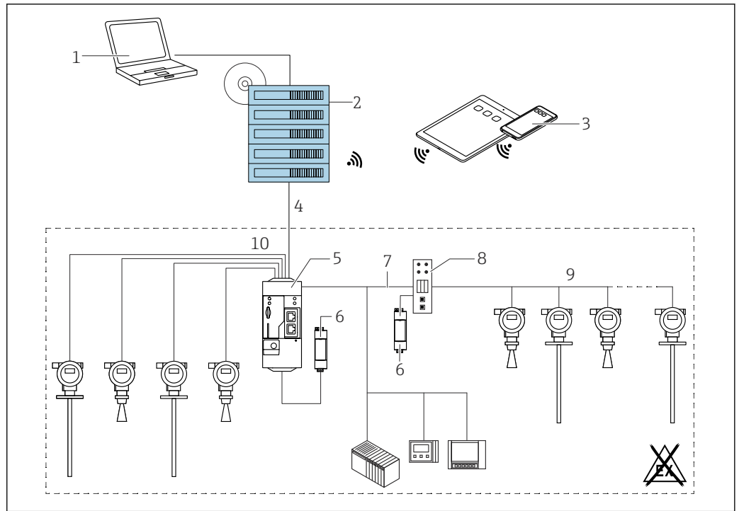
26 Ejemplo de plataforma para la gestión de inventario con SupplyCare Enterprise SCE30B
