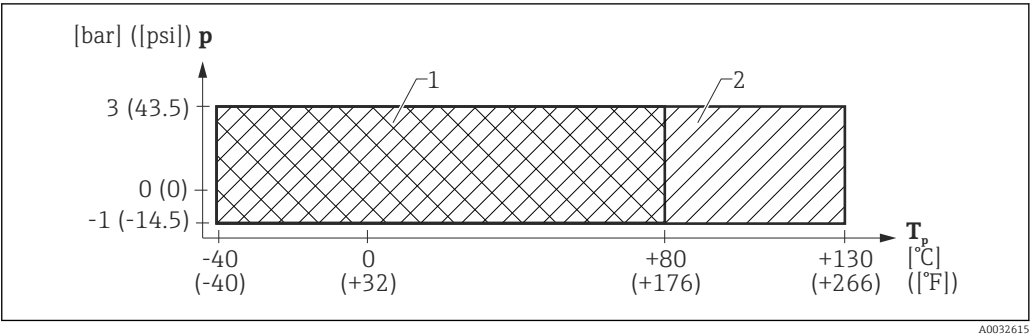
16 FMR60: Rango admisible para la temperatura del proceso y la presión del proceso
