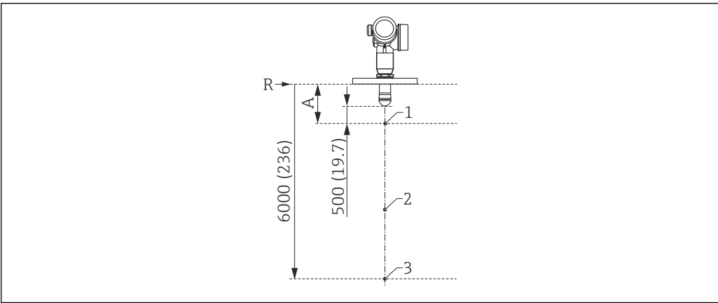
28 Puntos del protocolo de linealización a 3 puntos. Unidad de medida mm (in)
