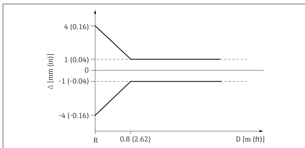
13 Error medido máximo en aplicaciones de rango cercano
