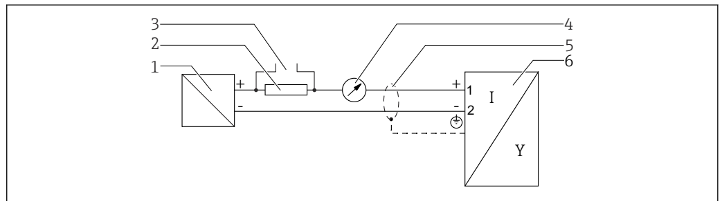
4 Diagrama en bloque a dos hilos: 4-20 mA HART
