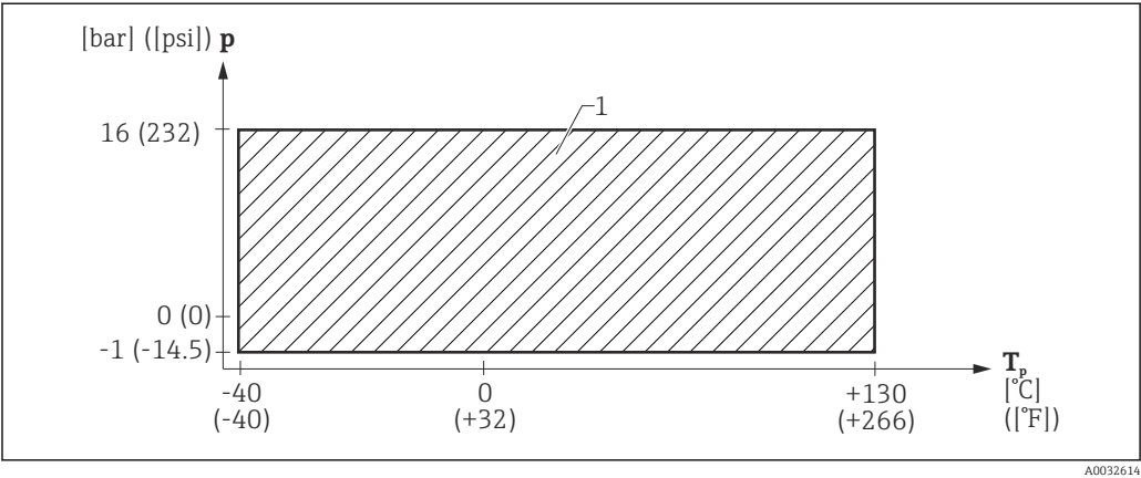
15 FMR60: Rango admisible para la temperatura del proceso y la presión del proceso
