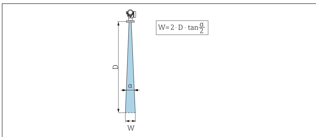
14 Relación entre el ángulo de abertura del haz \alpha , la distancia D y el diámetro del ancho del haz W
