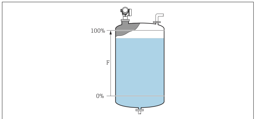
32 Калибровка полной емкости (F) для измерения уровня жидких сред
