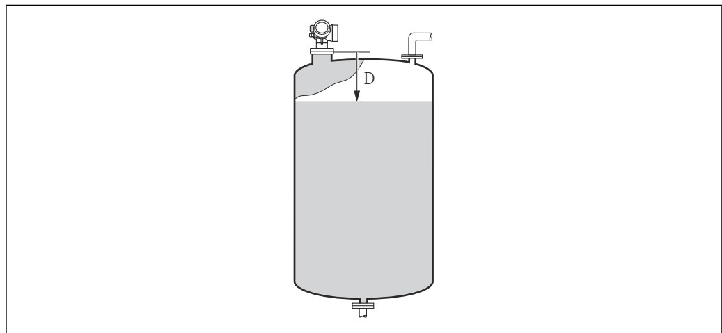
34 Расстояние для измерения в жидких средах
