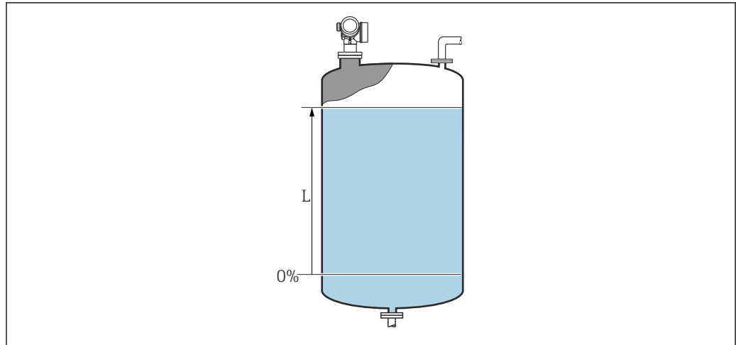
33 Уровень при измерении в жидких средах
