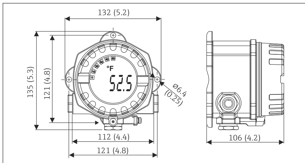
図 8 一般的なアプリケーション用のアルミダイカストハウジングまたはオプションのステンレスハウジング (SUS 316L 相当)
