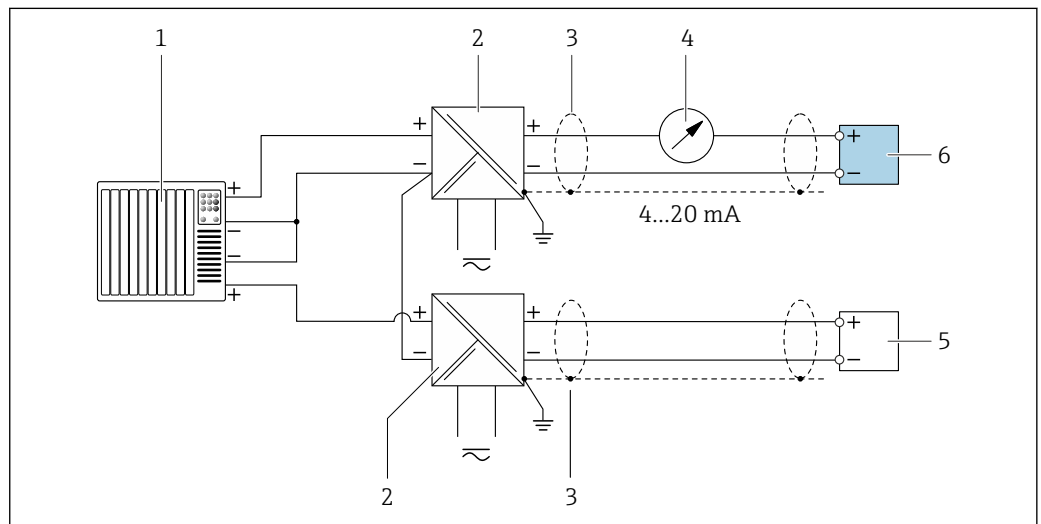
22 Przykład podłączenia dla układu z wejściem HART ze wspólnym "-" (pasywnym)
