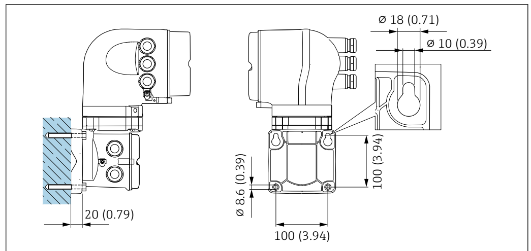
12 Jednostka: mm (in)
