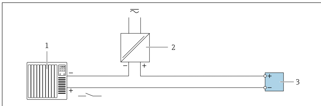
31 Przykład podłączenia wejścia statusu
