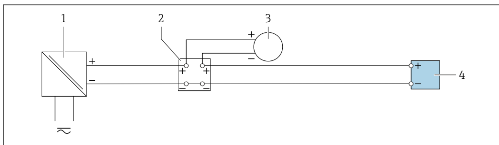
30 Przykład podłączenia wejścia prądowego 4...20 mA
