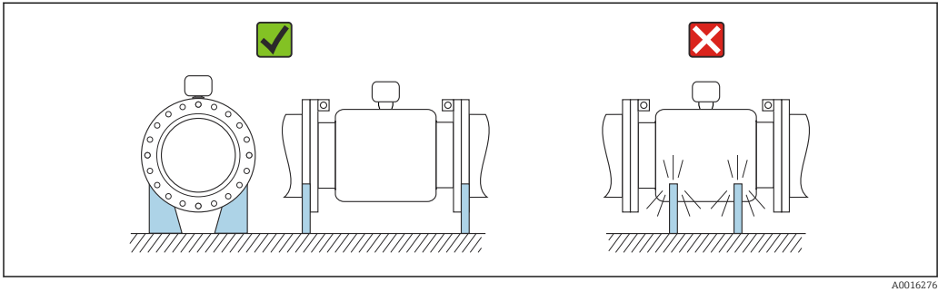
Czujniki o dużej masie DN ≥ 350 (14")
