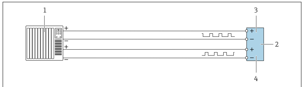
27 Przykład podłączenia podwójnego wyjścia impulsowego (aktywnego)
