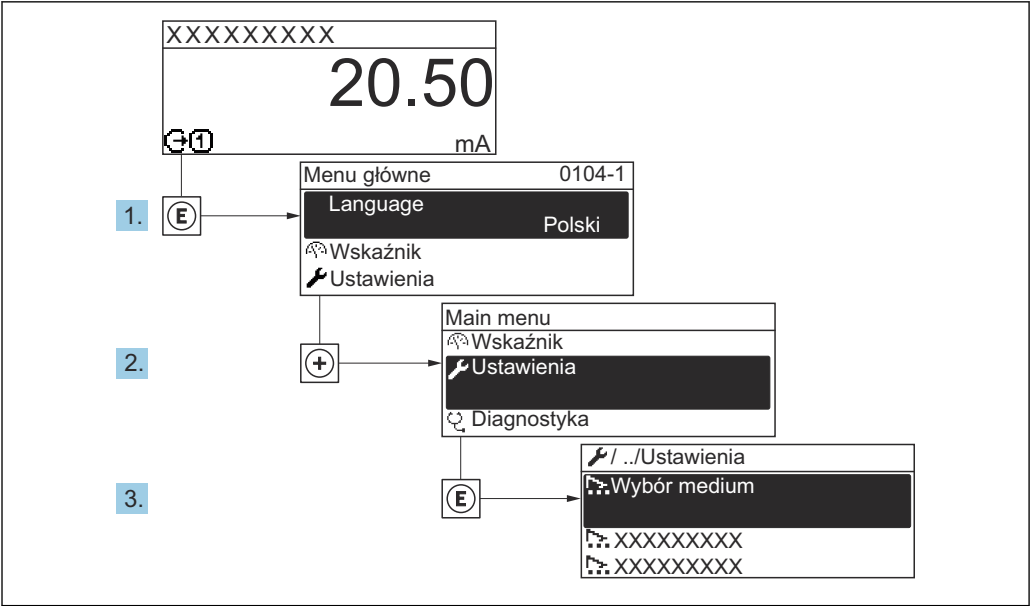
41 Przykład menu na wyświetlaczu lokalnym
