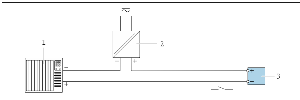
29 Przykład podłączenia wyjścia przekaźnikowego (pasywnego)
