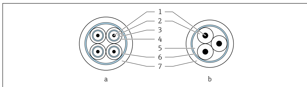
14 Przekrój przewodu
