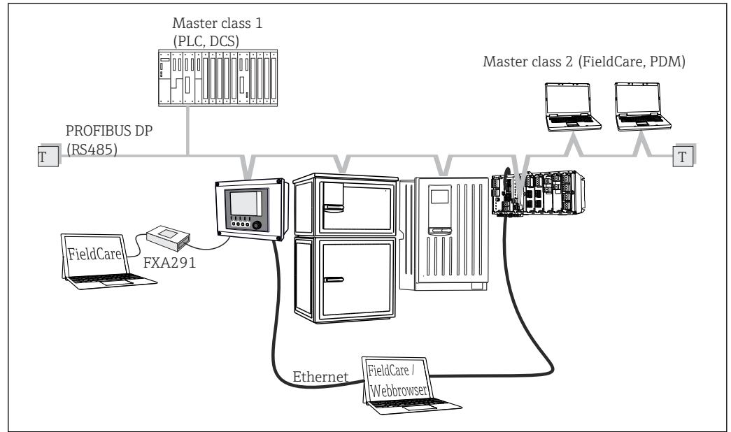
18 PROFIBUS DP
