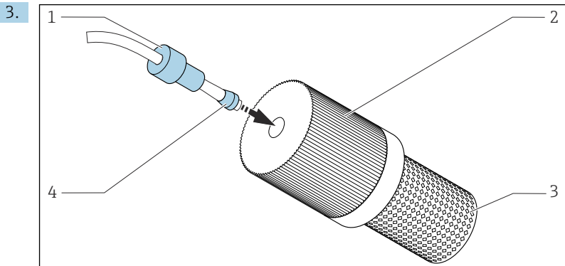
20 Montáž sacího sítka (součást dodávky) na vzorkovou hadičku
