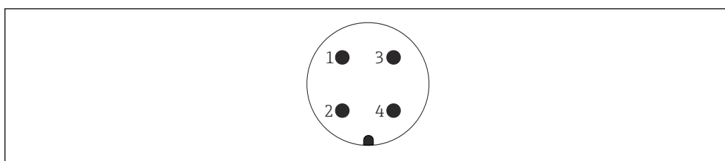
28 Asignación de pins del conector 7/8"
