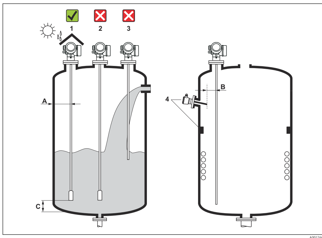
34 Condiciones de instalación para Levelflex
