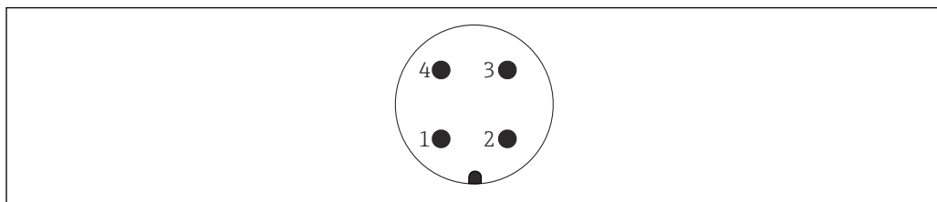
27 Asignación de pins del conector M12
