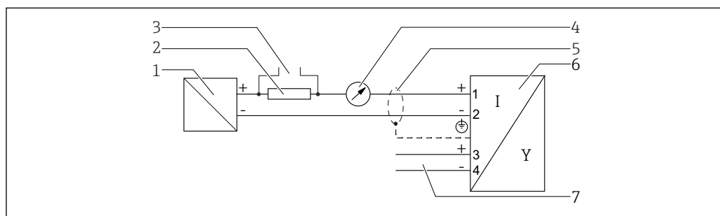
15 Diagrama en bloque a dos hilos: 4-20 mA HART, salida de conmutación
