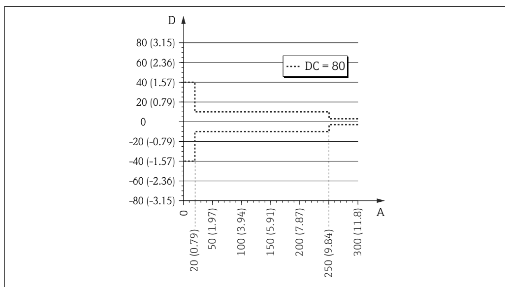
30 Error medido en el extremo de la sonda para sondas de cable
