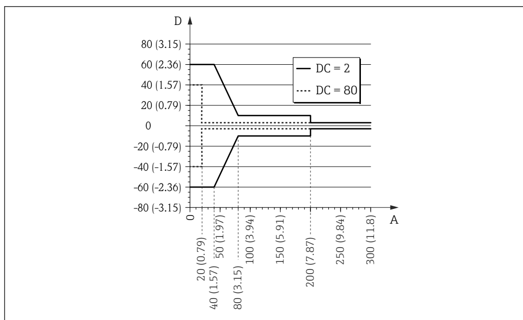
29 Error medido en el extremo de la sonda para sondas de varilla y coaxiales
