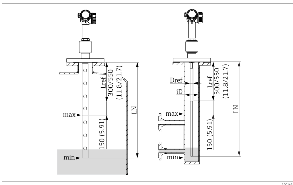
33 FMP54 con señal de referencia para la compensación de la fase gaseosa; unidad física: mm (in)
