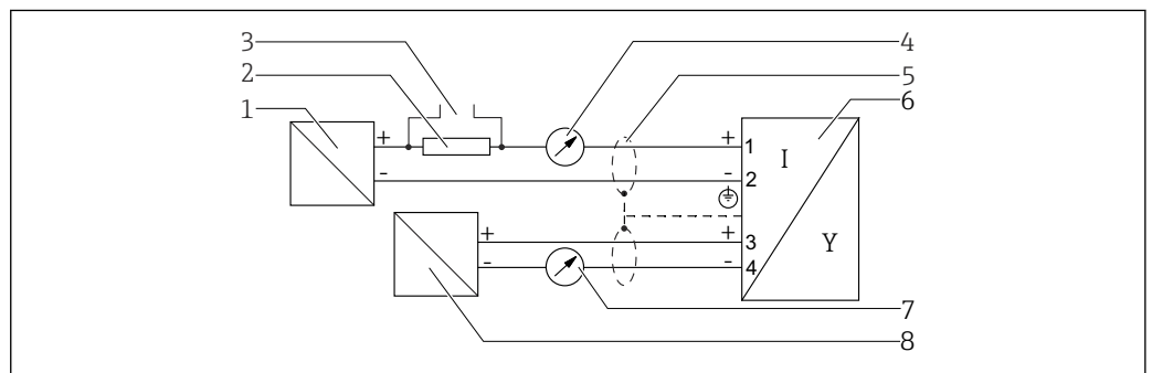
17 Diagrama en bloque a dos hilos: 4-20 mA HART, 4-20 mA
