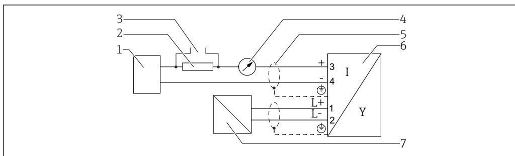
19 Diagrama en bloque a cuatro hilos: 4-20 mA HART (10,4 ... 48 V DC )
