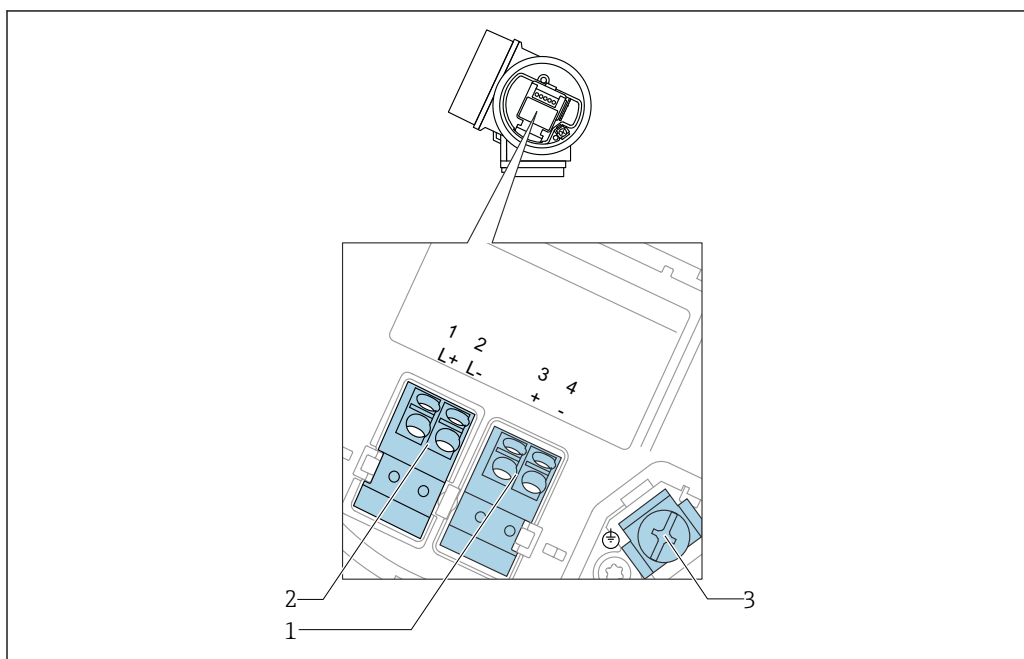
18 Asignación de terminales a cuatro hilos: 4-20 mA HART (10,4 ... 48 V DC )
