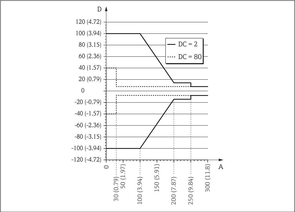
31 Error medido en el extremo de la sonda en el caso de discos de centrado metálicos (estructura de pedido del producto: característica 610 "Accesorio montado", versión OA, OB u OC)
