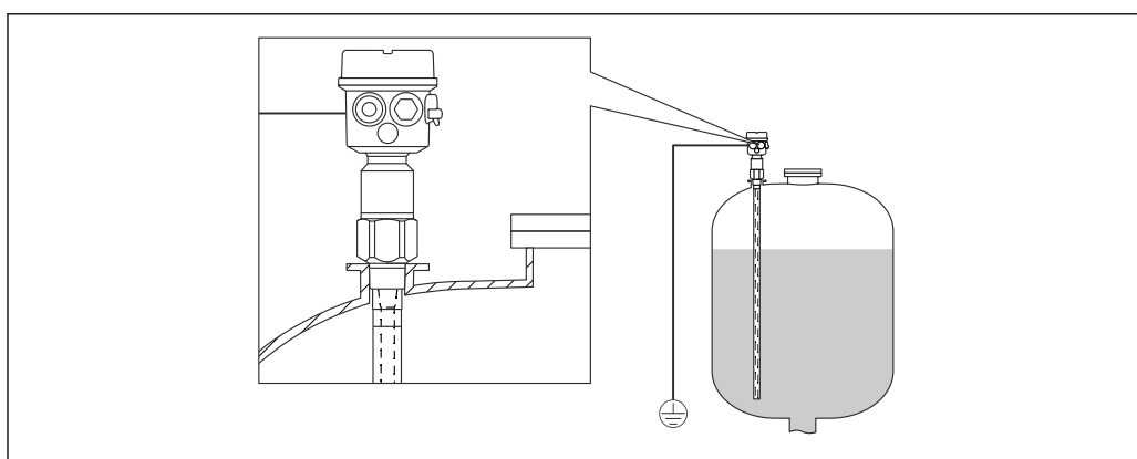
3 Sonde avec tube de masse pour cuves non conductrices
