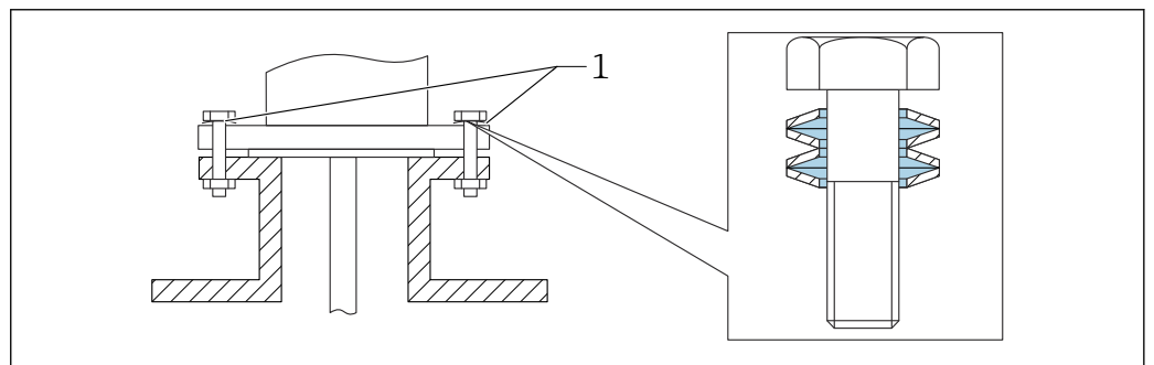
1 Rondelle élastique
