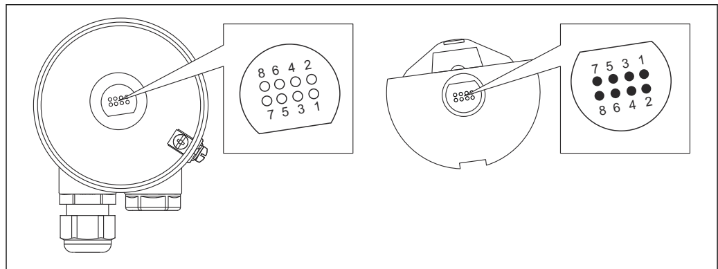
19 Contacts de l'électronique
