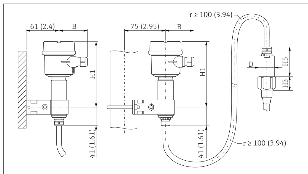
8 Côté boîtier : montage mural, montage sur conduite et côté capteur. Unité de mesure mm (in)
