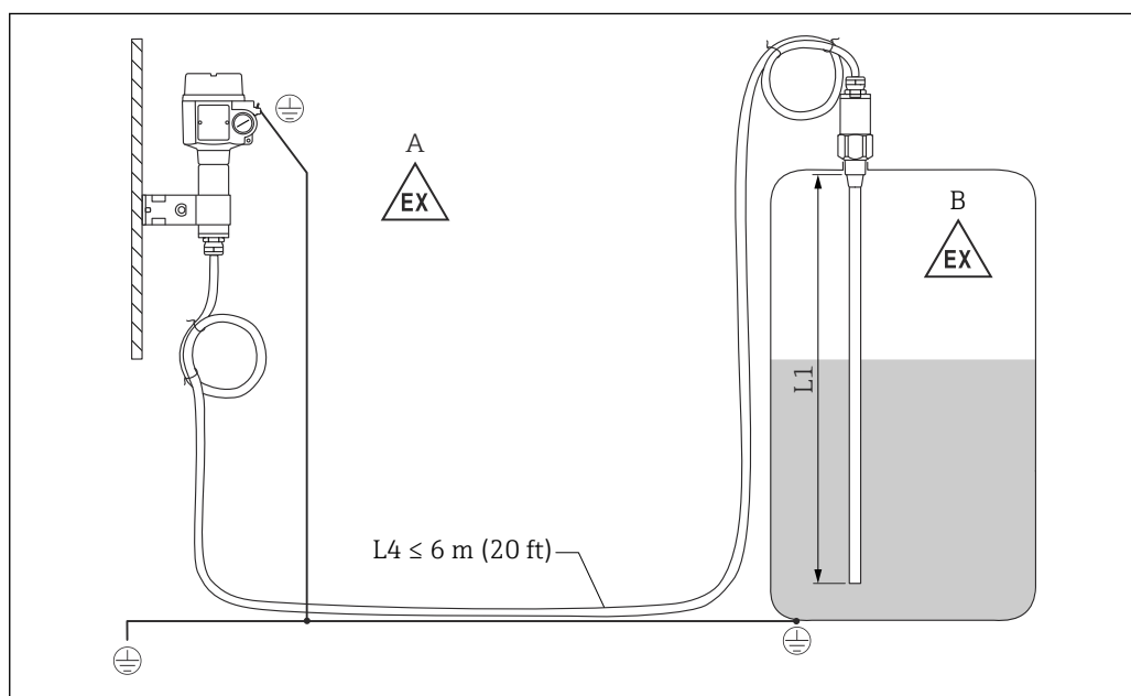
7 Raccordement de la sonde et du boîtier séparé
