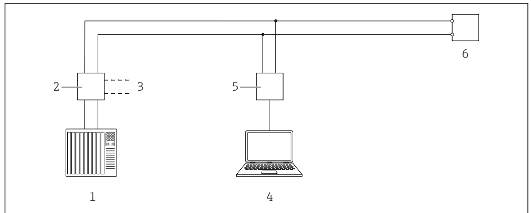
10 Commande à distance via protocole Hart
