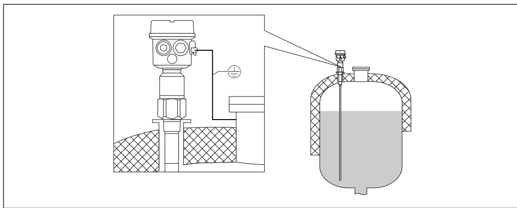
4 Sonde avec longueur inactive pour cuves isolées
