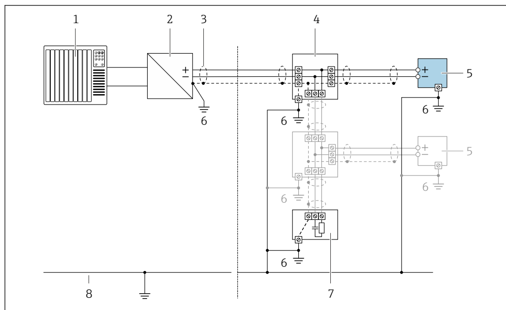
17 Exemple de raccordement pour PROFIBUS PA
