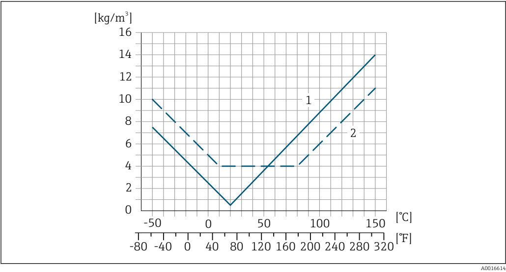
1 Étalonnage sur site de la masse volumique, exemple pour +20 °C (+68 °F) 2 Étalonnage spécial de la masse volumique
