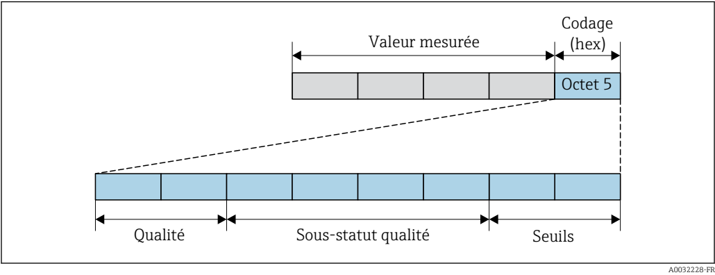
37 Structure du Coding-Byte
