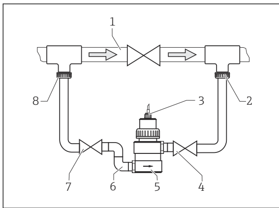
8 Instalação bypass com válvulas acionadas manualmente ou válvulas solenoide
