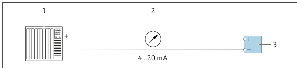
Fig. 18 Ejemplo de conexión de salida de corriente de 4-20 mA (activa)
