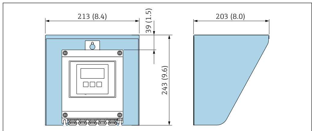
8 Cubierta protectora para Proline 500, digital; unidad física: mm (in)
