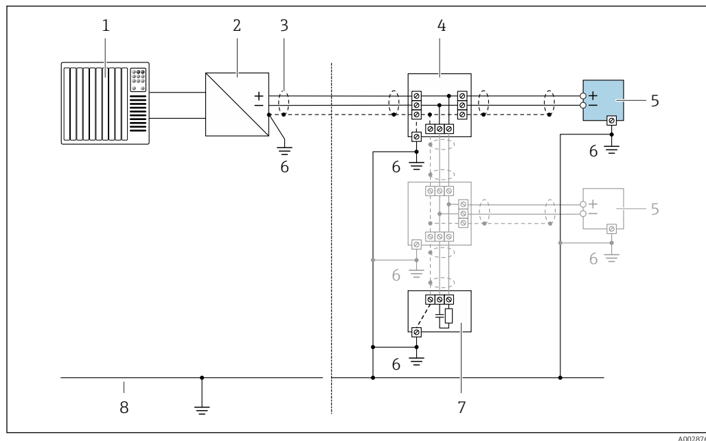
17 Exemplo de conexão elétrica para PROFIBUS PA
