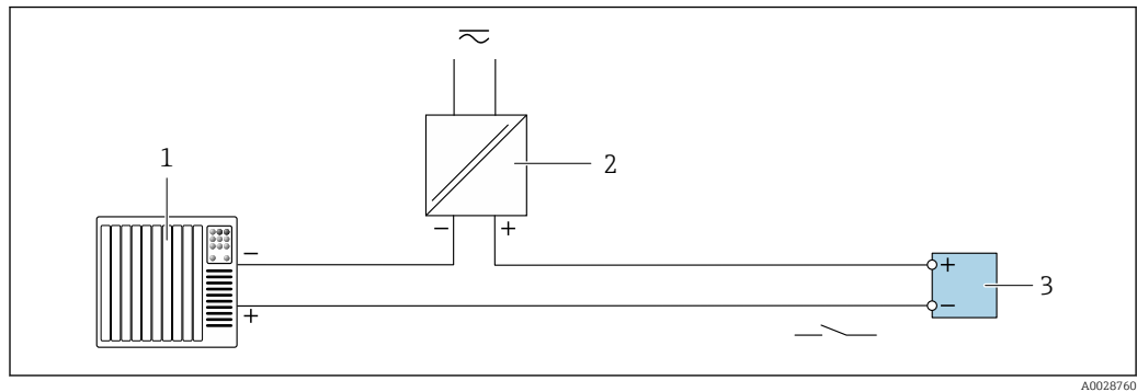
22 Exemplo de conexão para saída a relé (passiva)
