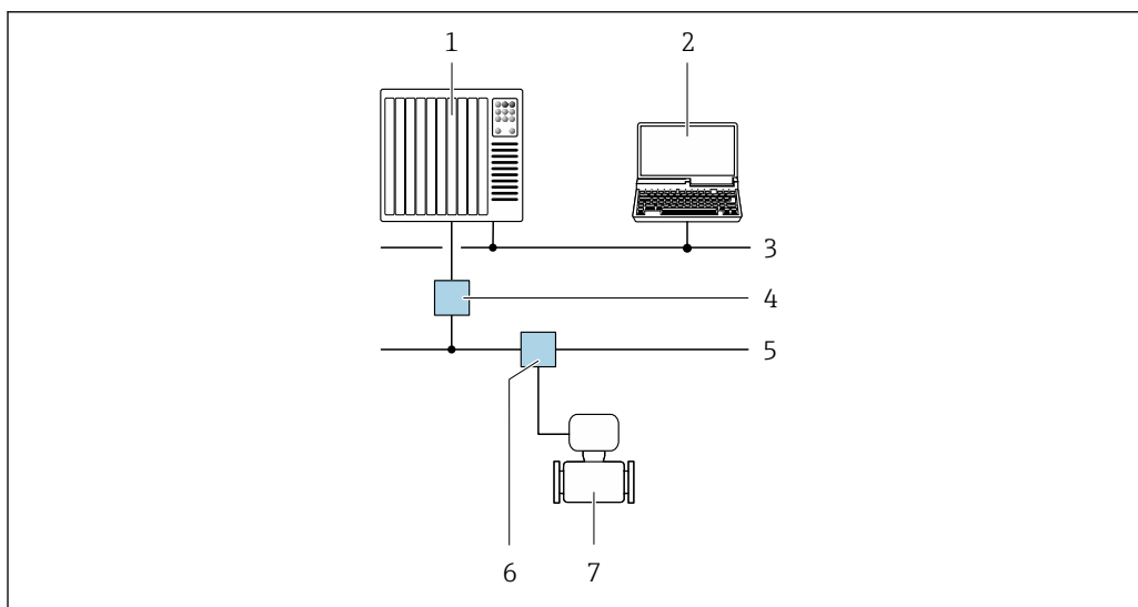
29 Opções para operação remota através da rede PROFIBUS PA
