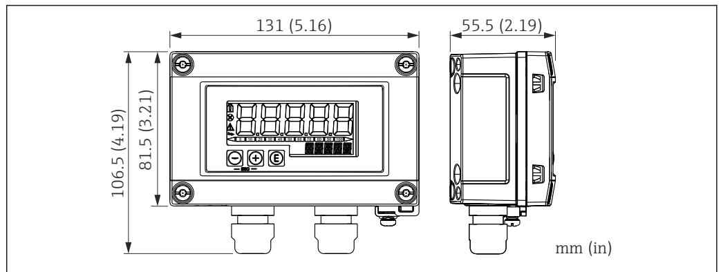
51 Dimensions du RIA15 en boîtier de terrain, unité de mesure : mm (in)
