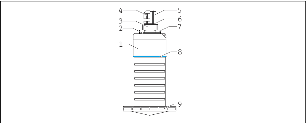
32 Aperçu des matériaux
