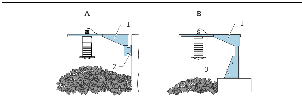
40 Type de montage raccord process arrière
