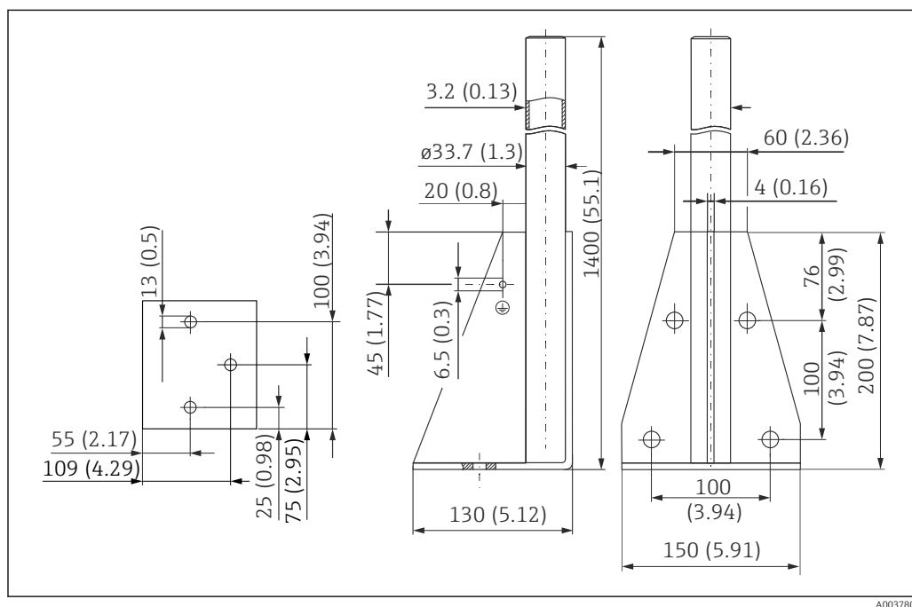
44 Dimensions. Unité de mesure mm (in)
