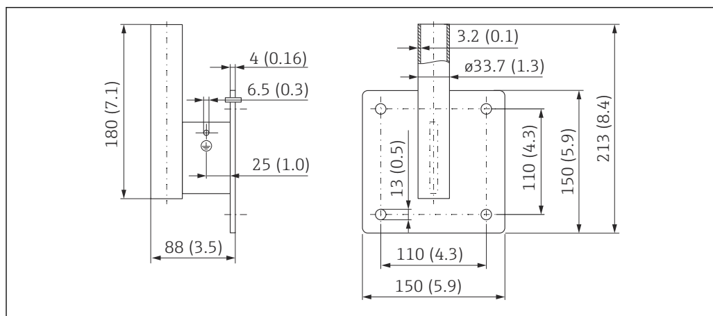
45 Dimensions du support mural. Unité de mesure mm (in)
