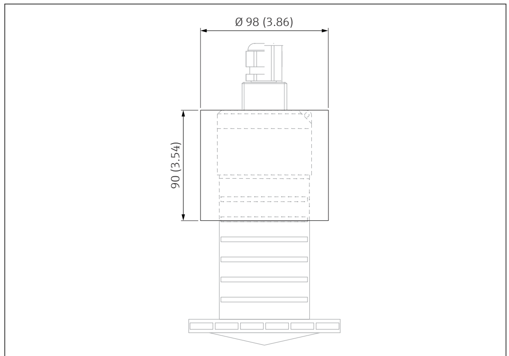
35 Dimensions du capot de protection climatique, unité de mesure : mm (in)
