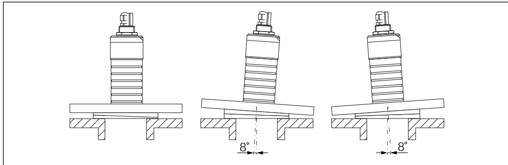
24 Micropilot FMR20 avec joint de bride biseauté
