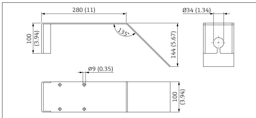
48 Dimensions de l'étrier de montage horizontal. Unité de mesure mm (in)
