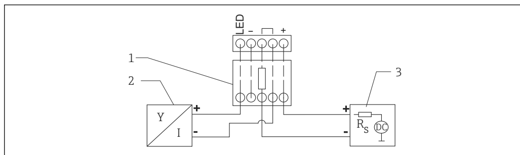
8 Schéma de principe de l'appareil HART, RIA15 avec rétroéclairage, module de résistance pour communication HART
