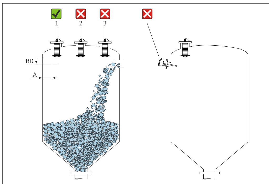
11 Position de montage sur un réservoir
