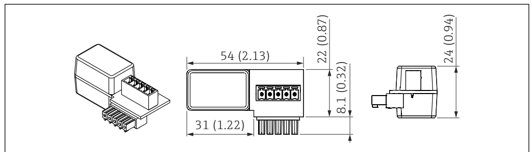
52 Dimensions de la résistance de communication HART, unité de mesure : mm (in)
