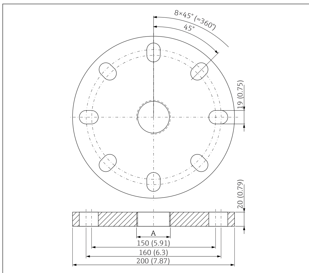
38 Dimensions de la bride UNI 3"/DN80/80, unité de mesure : mm (in)
