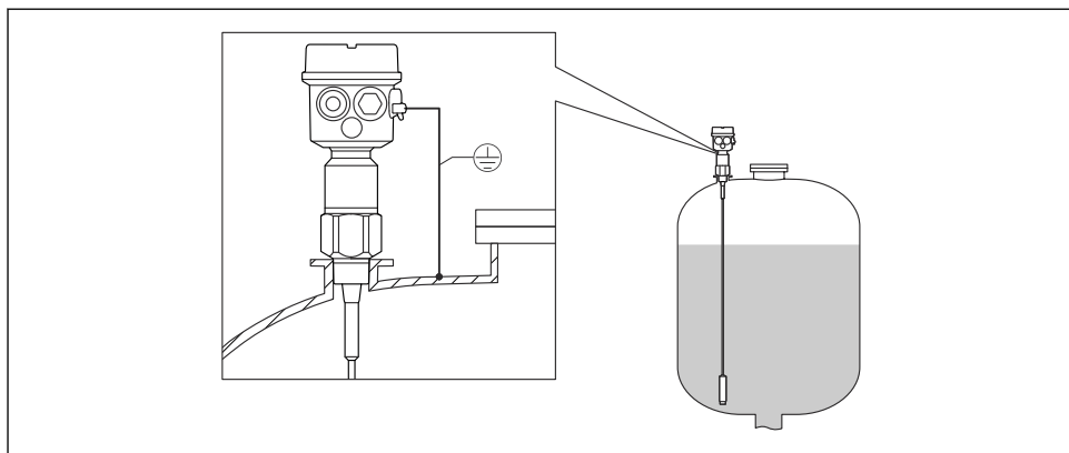
図 1 ローププローブ
