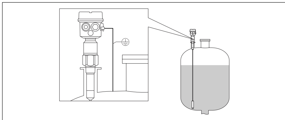
図 3 ノズル取付用の完全絶縁不感帯付きプローブ
