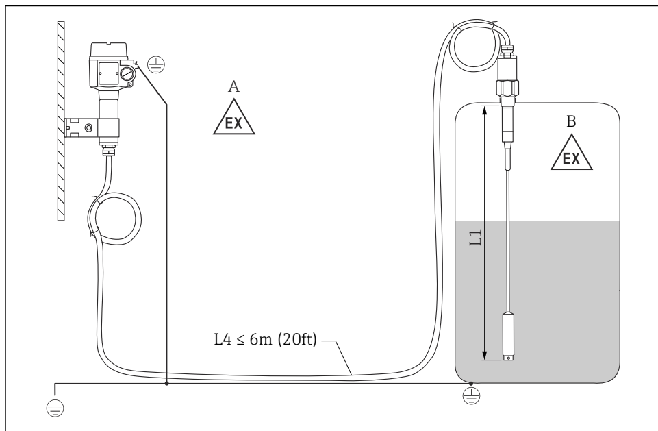
図 4 プローブと分離型ハウジングの接続
