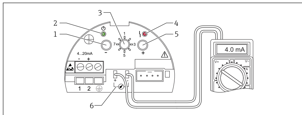
図 6 FEI50H エレクトロニックインサート
