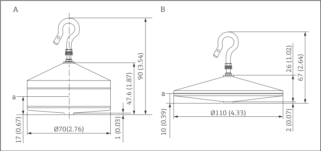
A Desplazador cónico de Ø70 mm (2,76 in) de 316L B Desplazador cónico de Ø110 mm (4,33 in) de 316L a Punto de inmersión
