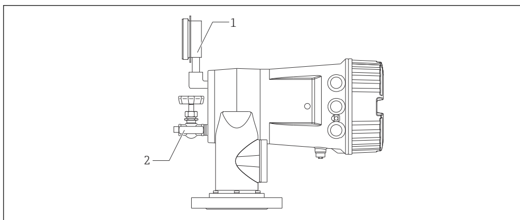
27 Posición de montaje de la válvula de descarga y el medidor de presión
