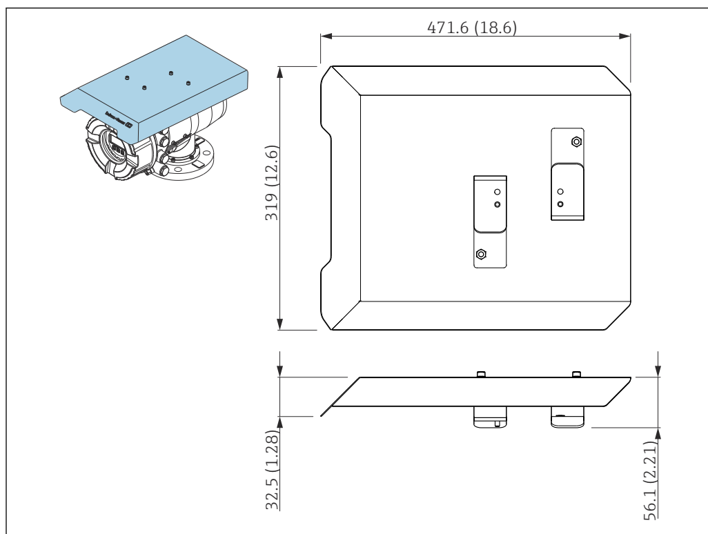
24 Tapa de protección ambiental, medidas: mm (in)
