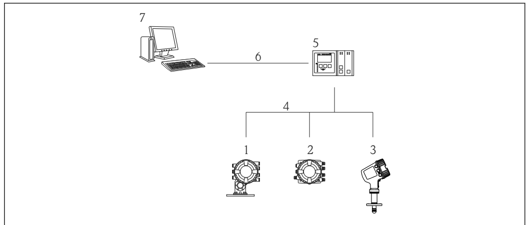
21 Configuración a distancia de equipos de medición de depósitos
