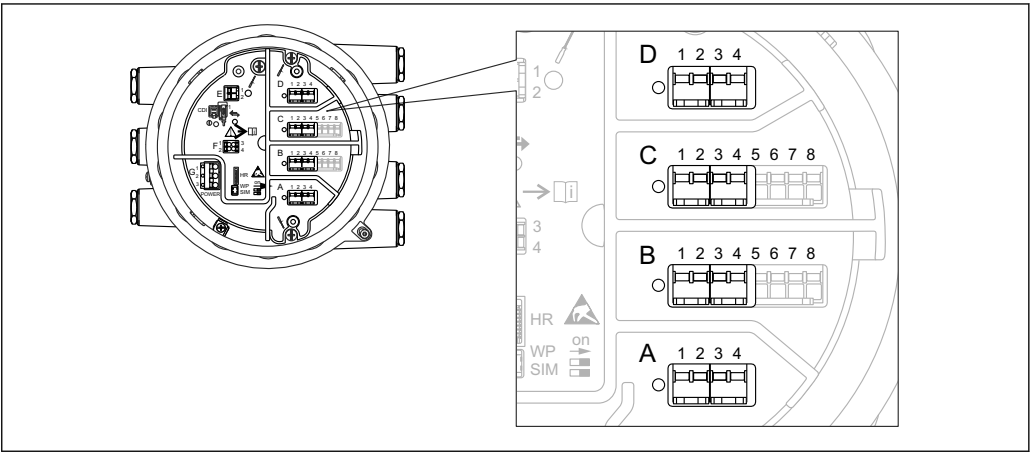
8 Posición de los módulos de E/S en el compartimento de terminales
