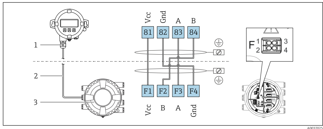
13 Conexión del módulo de indicación y configuración a distancia DKX001 al equipo de medición de depósitos (NMR8x, NMS8x o NRF8x)
