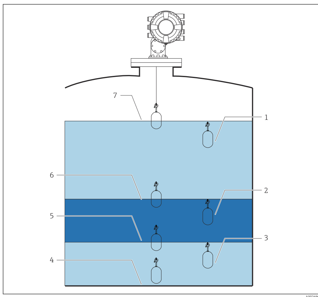
4 NMS8x con medición estándar de nivel, interfase x 2, fondo del depósito y densidad puntual x 3
