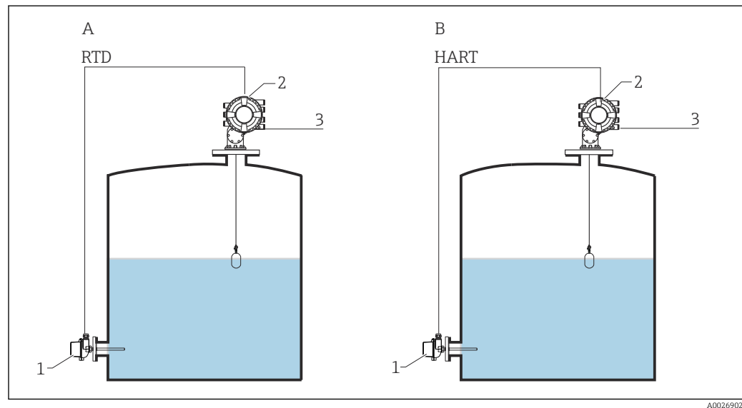
2 Sistema de medición para NMS83
