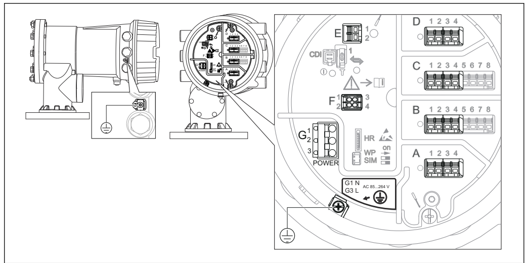
11 Compartimento de terminales (ejemplo típico) y bornes de tierra
