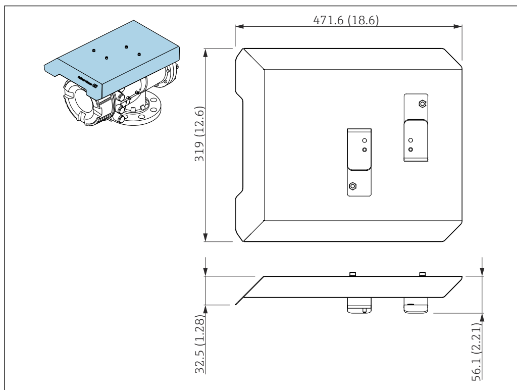
23 Tapa de protección ambiental, medidas: mm (in)
