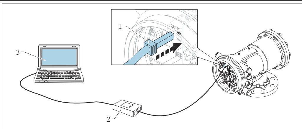
21 Configuración a través de la interfaz de servicio
