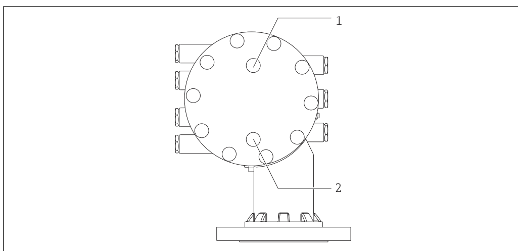
27 Orificios para la boquilla de limpieza y la tubuladura de purga de gas
