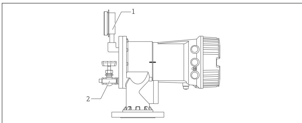
26 Posición de montaje de la válvula de descarga y el medidor de presión
