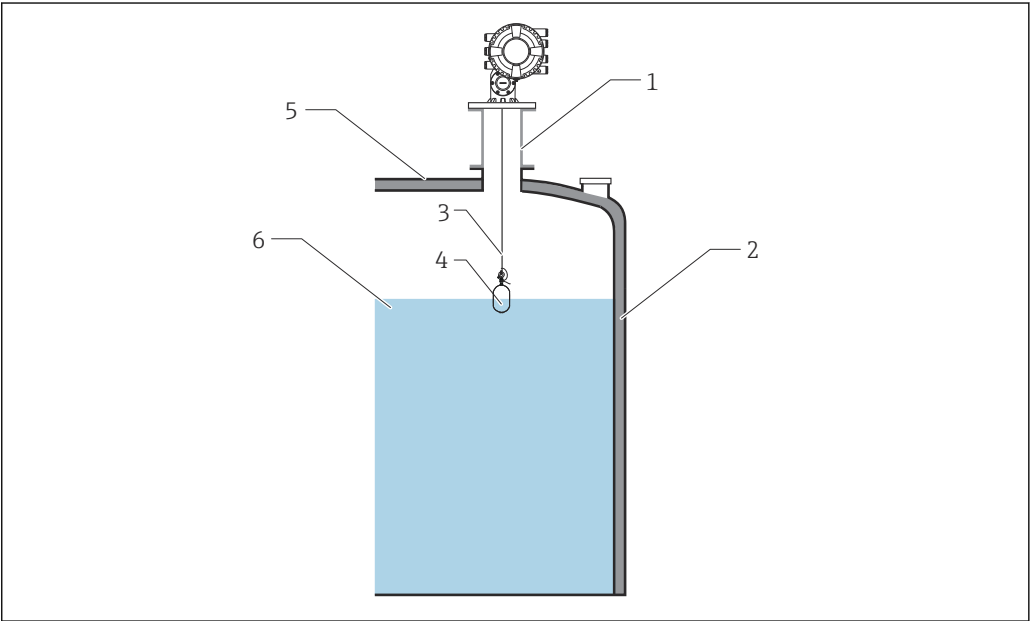
17 Sellado del proceso
