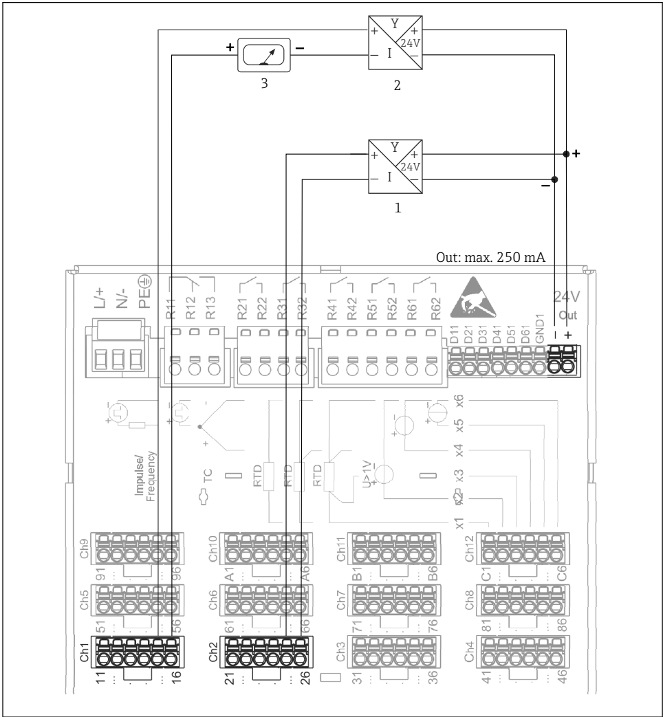
4 Anschluss des Hilfsspannungsausgangs bei Verwendung als Messumformerspeisung (MUS) für 4-Leiter-Sensoren im Strommessbereich. (Bei Anschluss von Kanal CH3-12 siehe Steckerbelegung CH1-2.)
