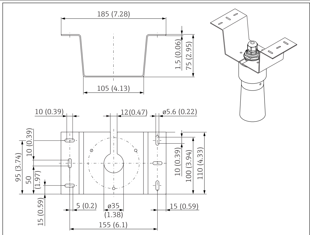
☐ 22 천장 설치용 설치 브래킷. 측정 단위 mm (in)
