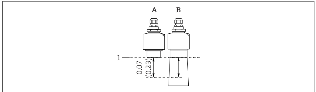
☐ 1 초음파 센서의 불감대. 공학 단위 m (ft)
