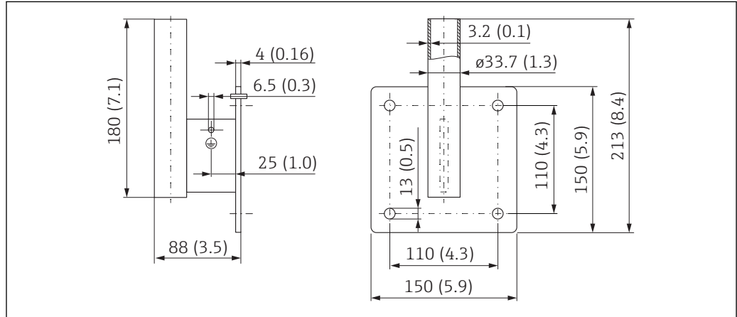
☐ 21 벽 브래킷 치수. 측정 단위 mm (in)
