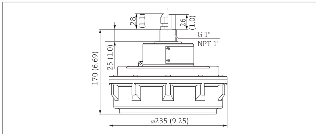
8 Wymiary. Jednostka miary mm (in)
