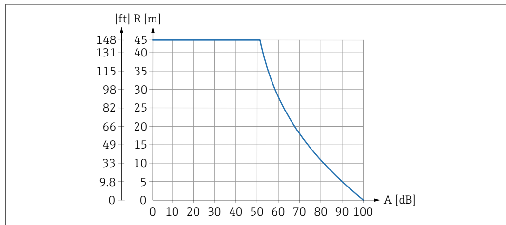
2 Zakresy pomiarowe czujników ultradźwiękowych
