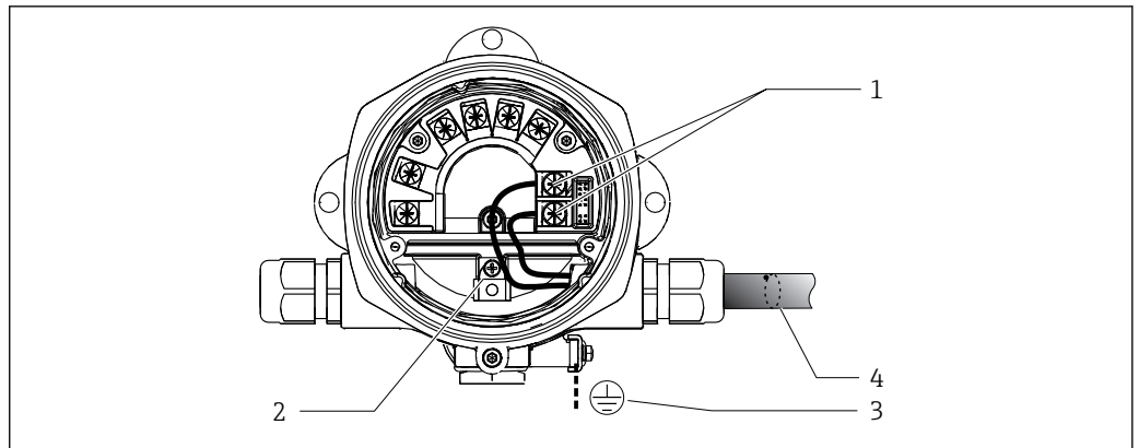
■ 7 Conexión al cable del bus de campo FOUNDATION Fieldbus™
