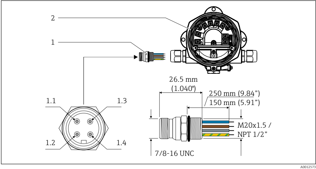
8 Conectores para la conexión del FOUNDATION Fieldbus™
