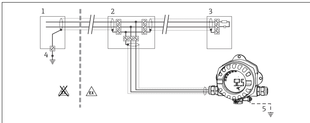
9 Blindaje y conexión a tierra unilateral del blindaje del cable de bus de campo
