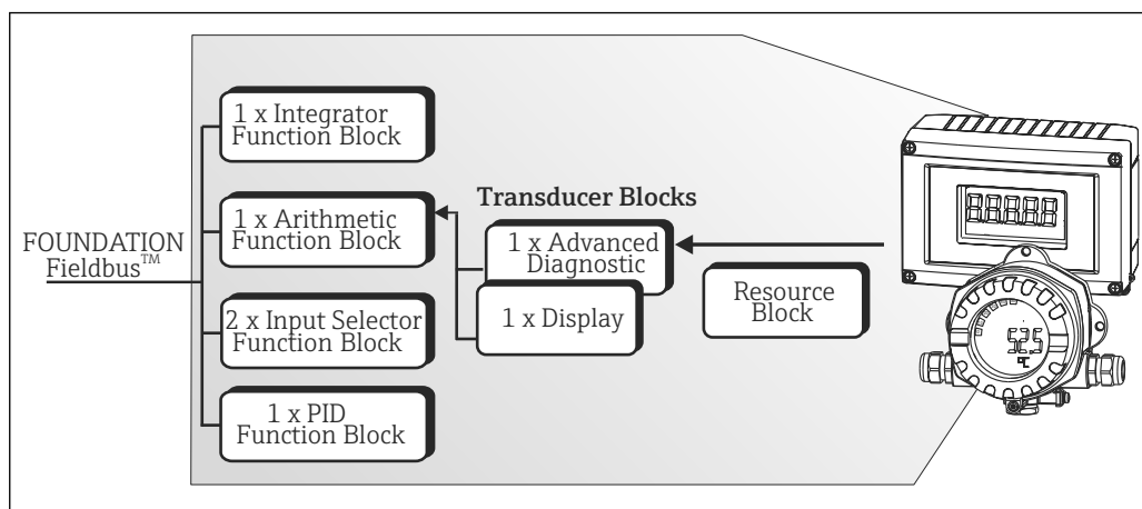
18 Esquema en bloques RID1x
