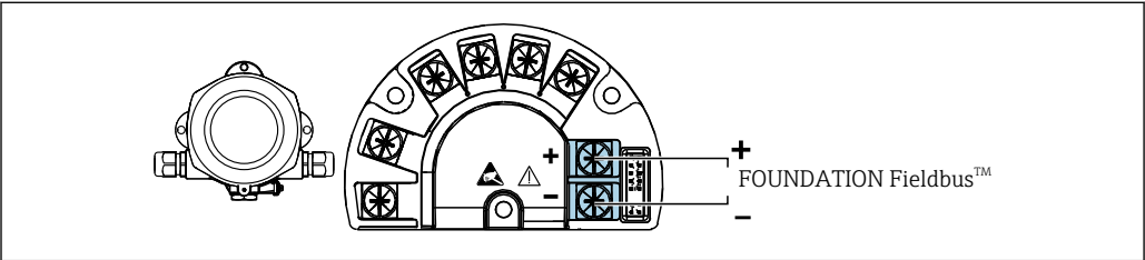
6 Asignación de terminales
