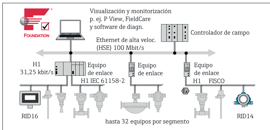
Fig. 12 Integración del sistema con FOUNDATION Fieldbus™
