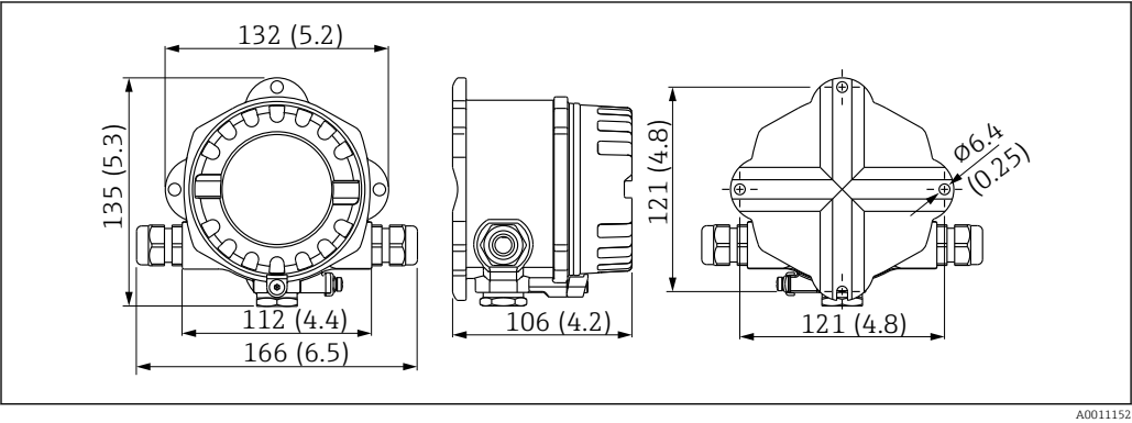
16 Dimensiones del indicador de campo; dimensiones en mm (pulgadas)
