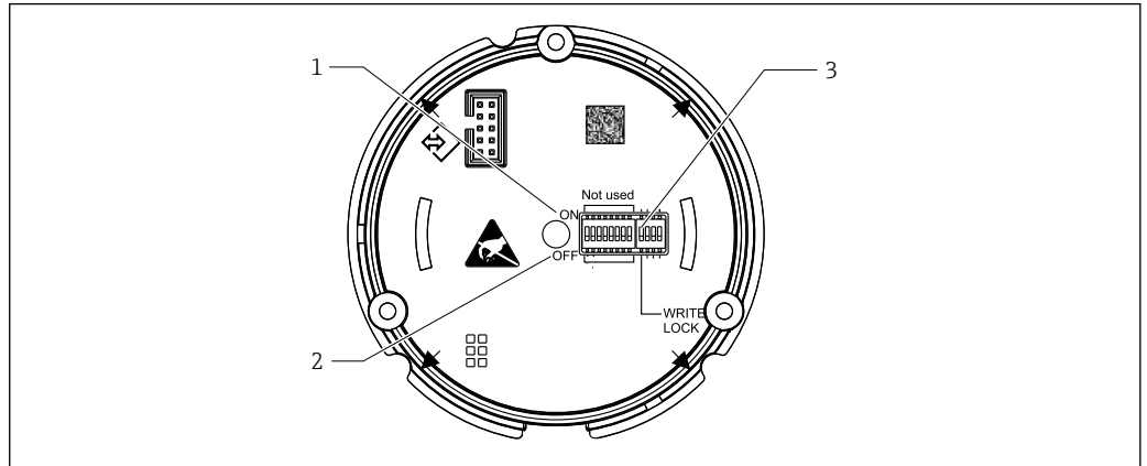
13 Parámetros de configuración del hardware mediante microinterruptores
