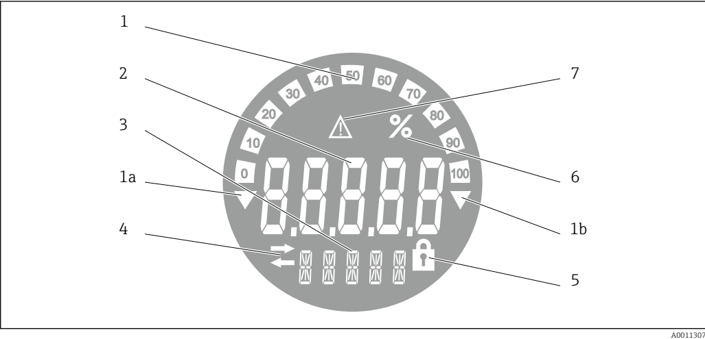
17 Pantalla de cristal líquido del indicador de campo (retroiluminado, puede insertarse en etapas de 90°) 1 Visualizador de gráfico de barras en incrementos del 10% con indicadores para indicación por debajo (elemento 1a) y por encima (elemento 1b) del rango 2 Visualización del valor medido, altura del dígito 20,5 mm (0,8 in), indicación de estado "estado de valor medido malo" 3 Indicador de 14 segmentos para unidades y mensajes 4 Símbolo "Comunicación" 5 Símbolo "Configuración bloqueada" 6 Unidad "%" 7 Símbolo "Estado del valor medido incierto"
