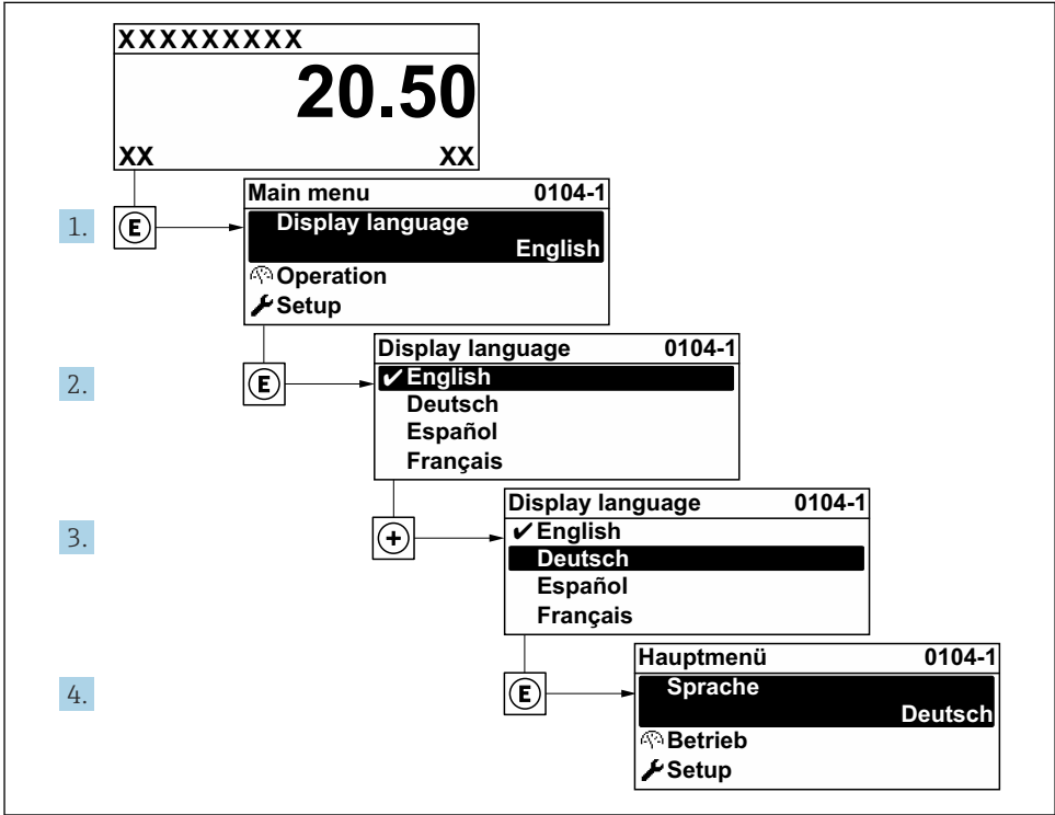
图 2 现场显示示意图
