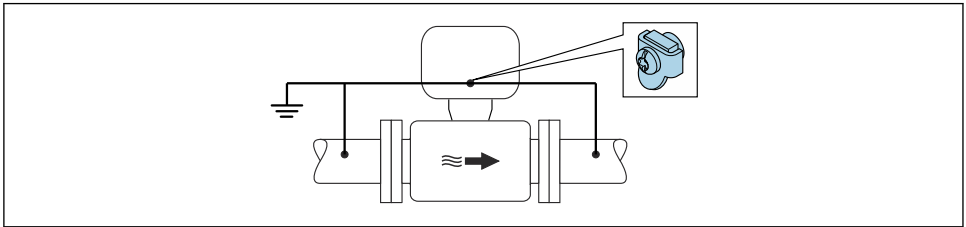
6 Potenzialausgleich über Messrohr
