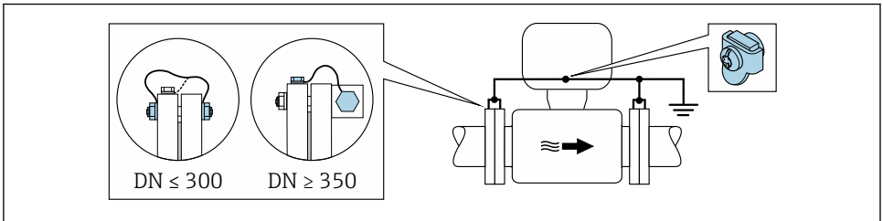
7 Potenzialausgleich über Erdungsklemme und Rohrleitungsflansche
